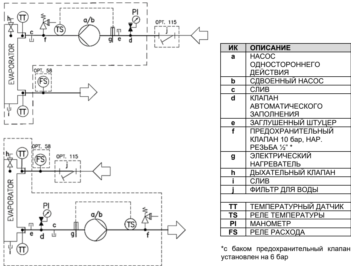
Рисунок 7 - Схема подключения водопроводных труб для испарителя (компл. 78-79-80-81)
