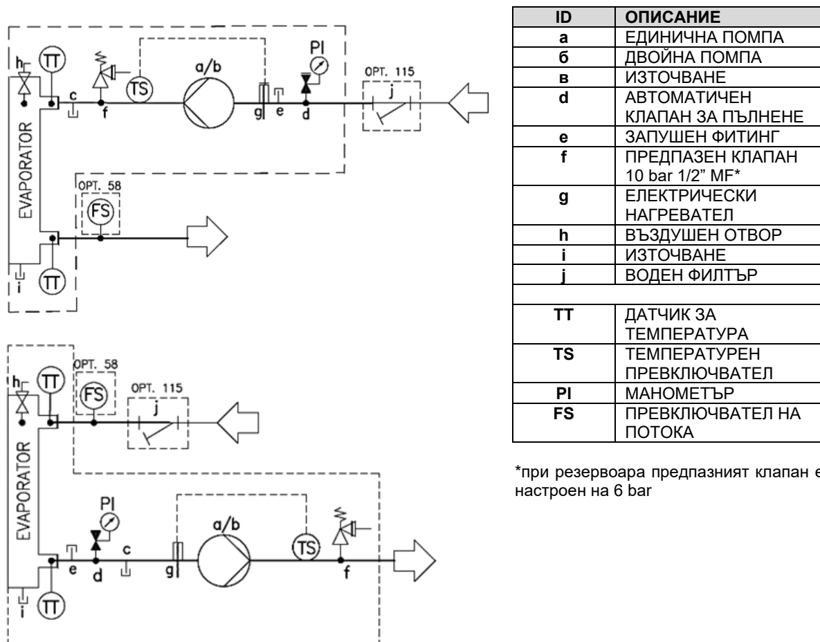
Схема 8. - Свързване на водопроводните тръби на топлообменниците за регенериране на топлинна енергия
