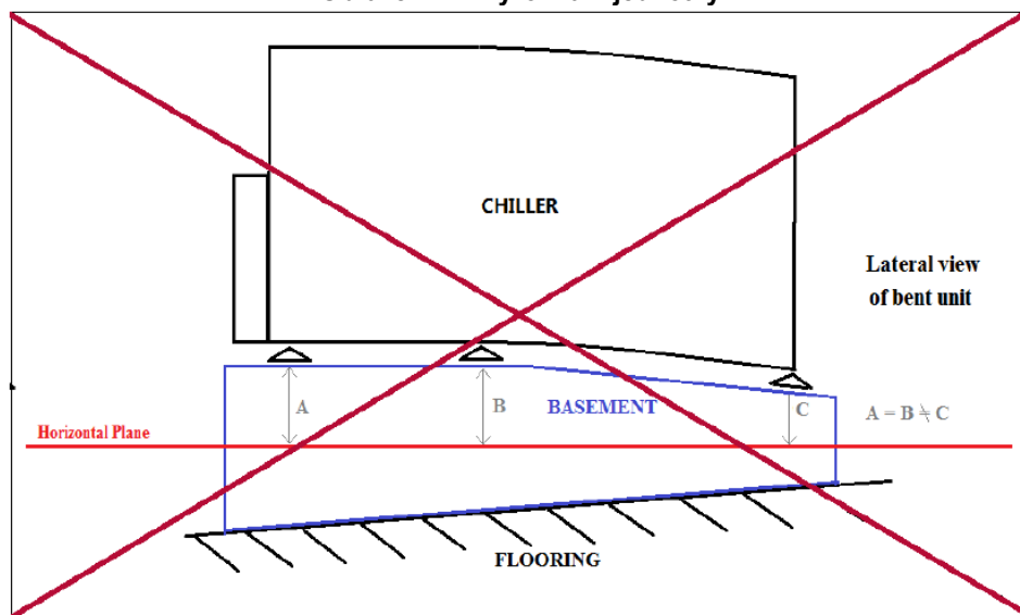
Obrázek 4. – Vyrovnání jednotky
