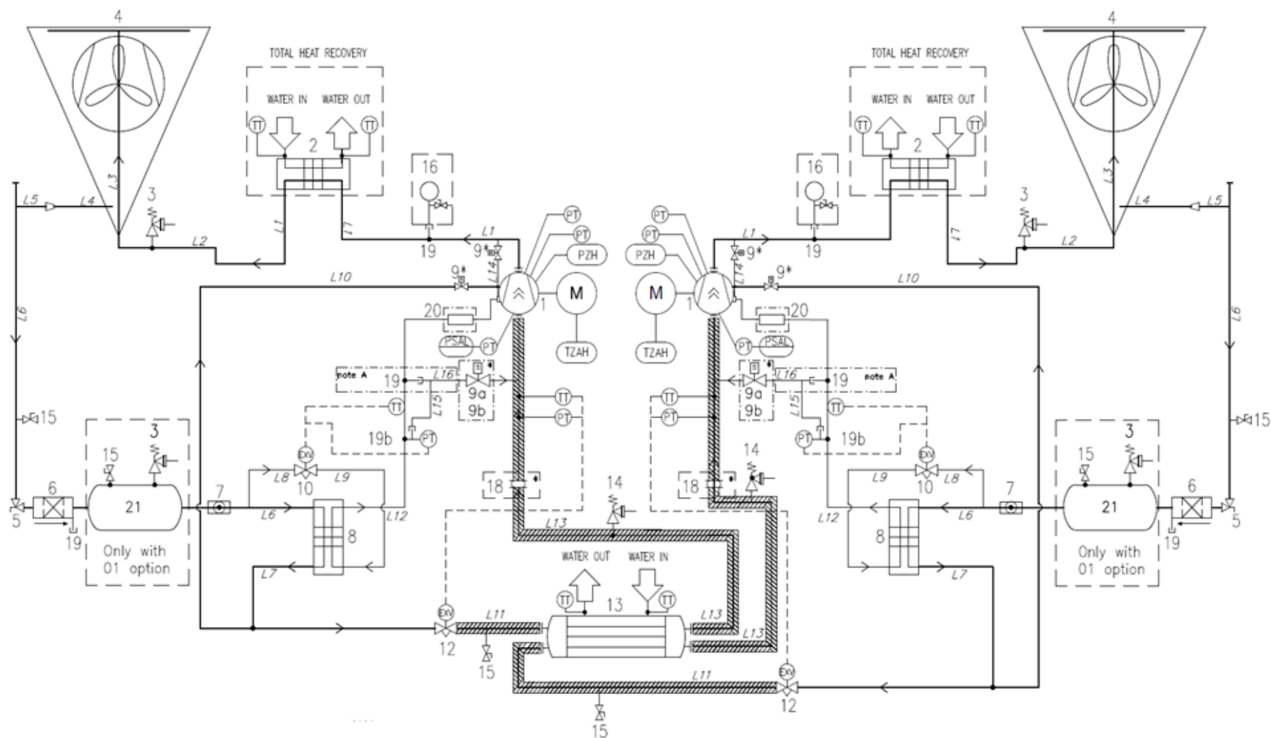
Obrázek 1 - Typický okruh chladiva
