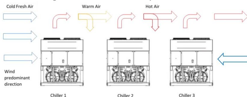
Figura 6 – Instalación de múltiples enfriadores
