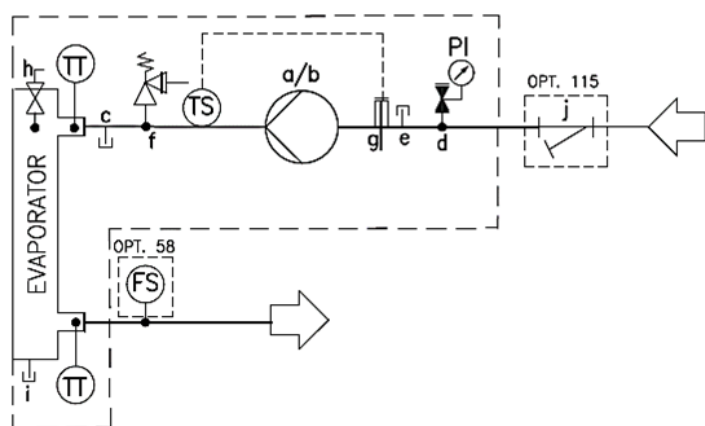
Figura 7 - Conexión de tubos del agua para el evaporador (opc.78-79-80-81)
