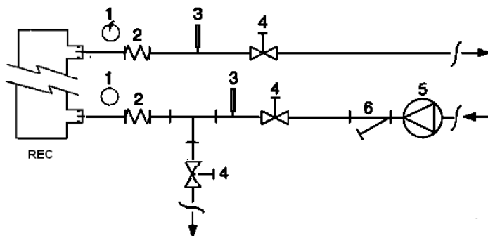
Figura 8 - Collegamento dei tubi dell'acqua per gli scambiatori di recupero di calore
