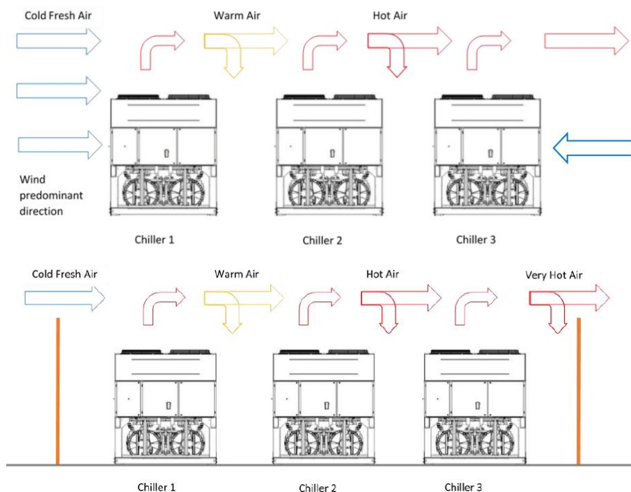
Rysunek 6 – Montaż kilku agregatów chłodniczych
