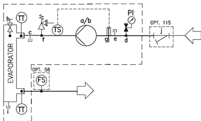
Figura 7. - Racord pentru conducta de apă pentru evaporator (opțional 78-79-80-81)
