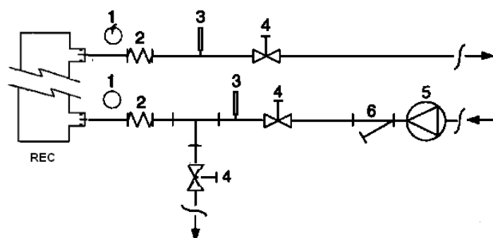
Figura 8. - Racordarea conductelor de apă pentru schimbătoarele de recuperare a căldurii
