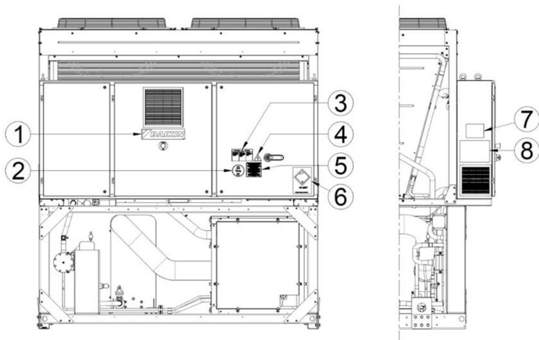
Figur 2. - Beskrivelse av etikettene på det elektriske panelet
