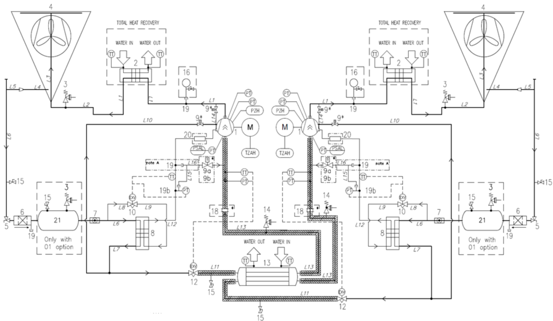
Vanninntak og -utløp er veiledende. Se maskindimensjonsdiagrammene for nøyaktige vanntilkoblinger
