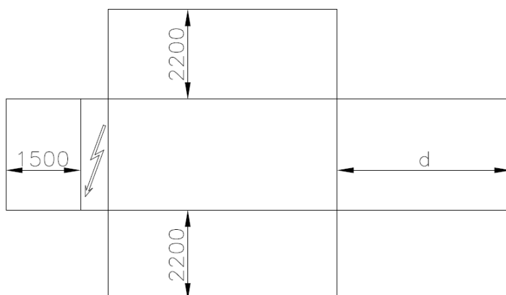
Rysunek 5- Minimalne wymagania dotyczące wolnej przestrzeni
