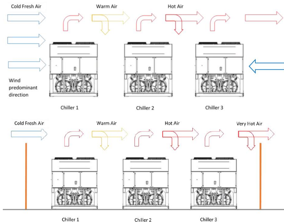
Figura 6 – Instalação de refrigerador múltiplo
