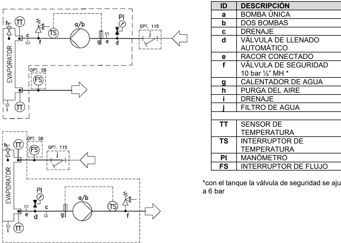
Figura 7 - Conexión de tubos del agua para el evaporador (opc.78-79-80-81)
