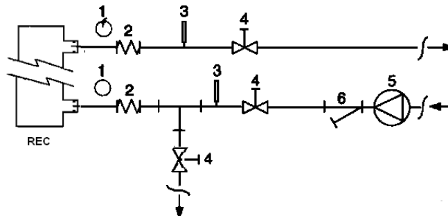
Figure 8 - Raccordement des tuyaux d'eau pour les échangeurs de récupération de chaleur
