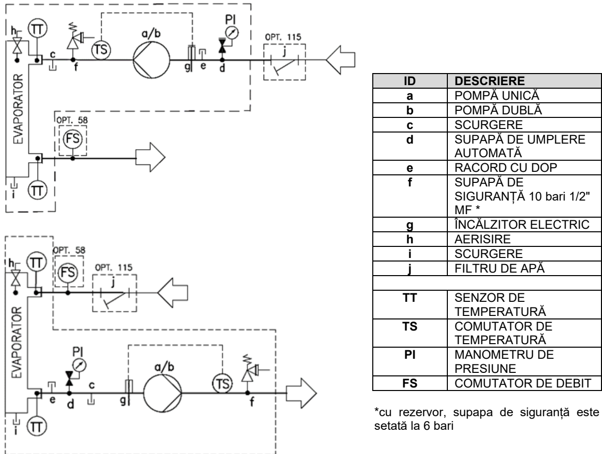
Figura 7. - Racord pentru conducta de apă pentru evaporator (opțional 78-79-80-81)
