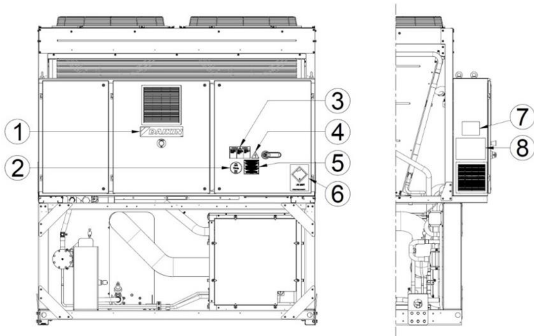
Рисунок 2 - Описание этикеток на электрическом щите
