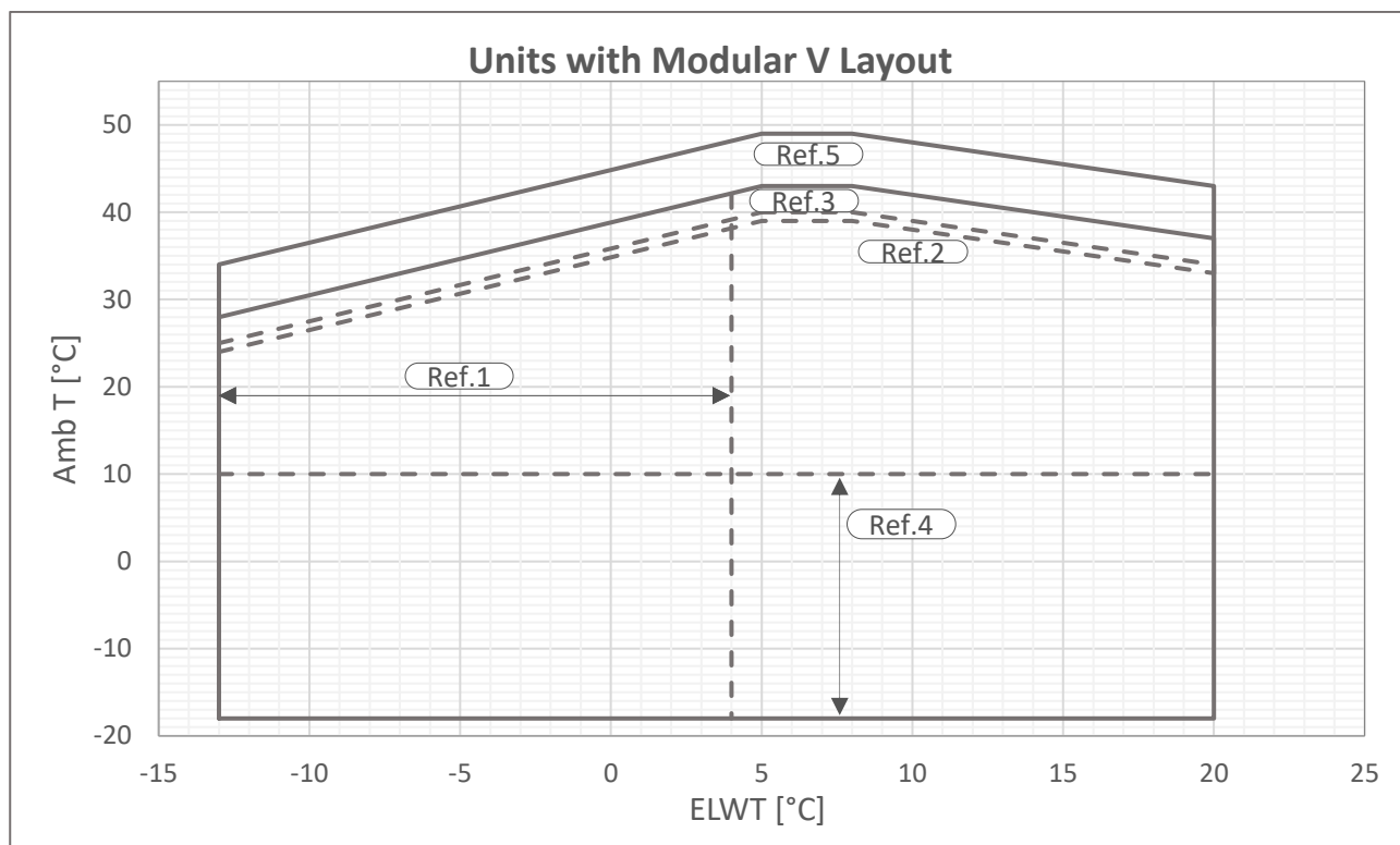
Εικ. 9 – Πολλαπλά V - Όρια λειτουργίας Silver
