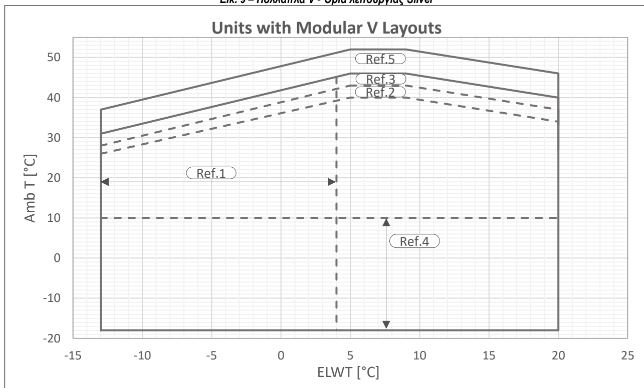
Εικ. 10 – Πολλαπλά V - Όρια λειτουργίας Gold
