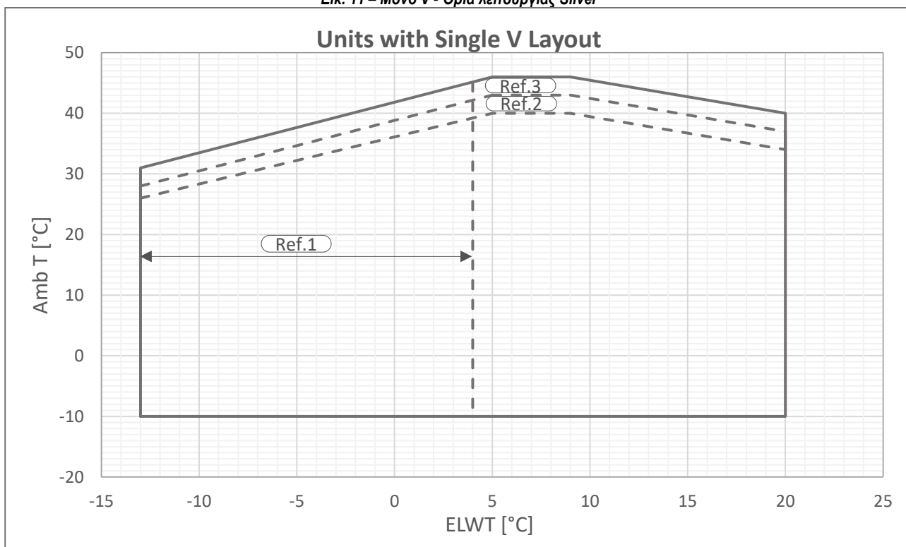
Εικ. 12 – Μονό V - Όρια λειτουργίας Gold
