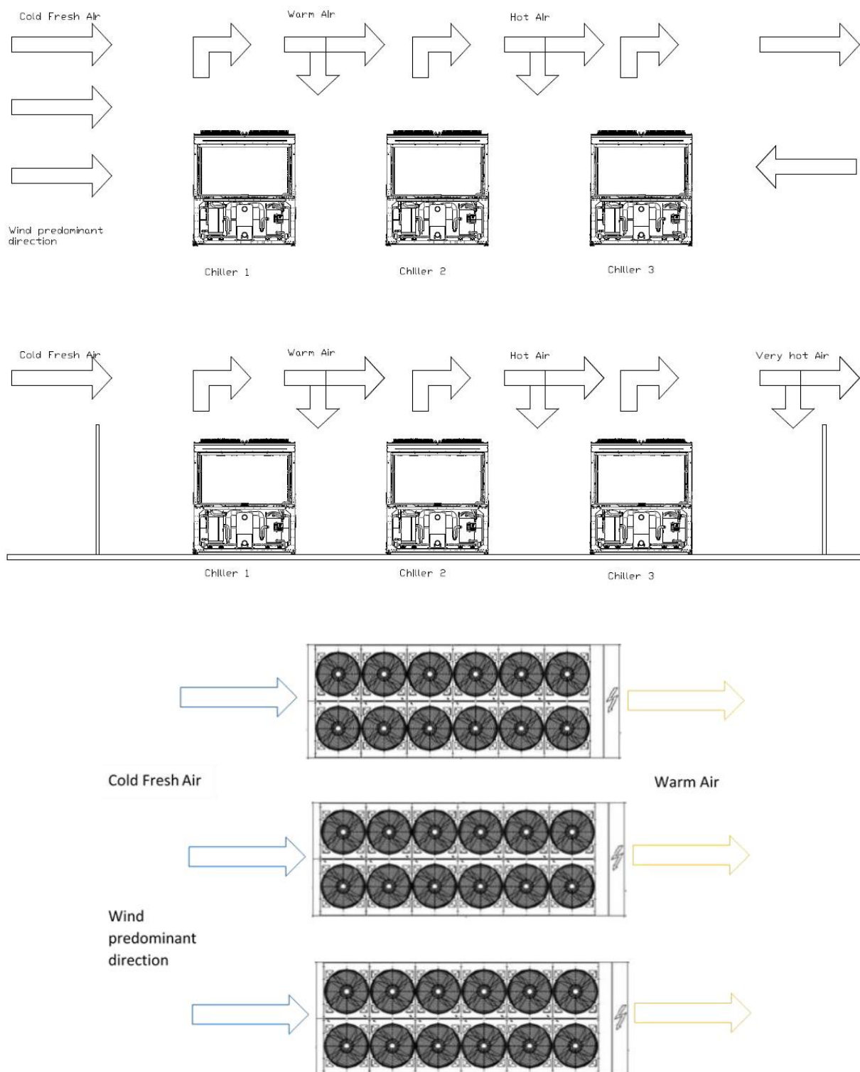
Fig. 4 – Instalación de Múltiples Refrigeradores
