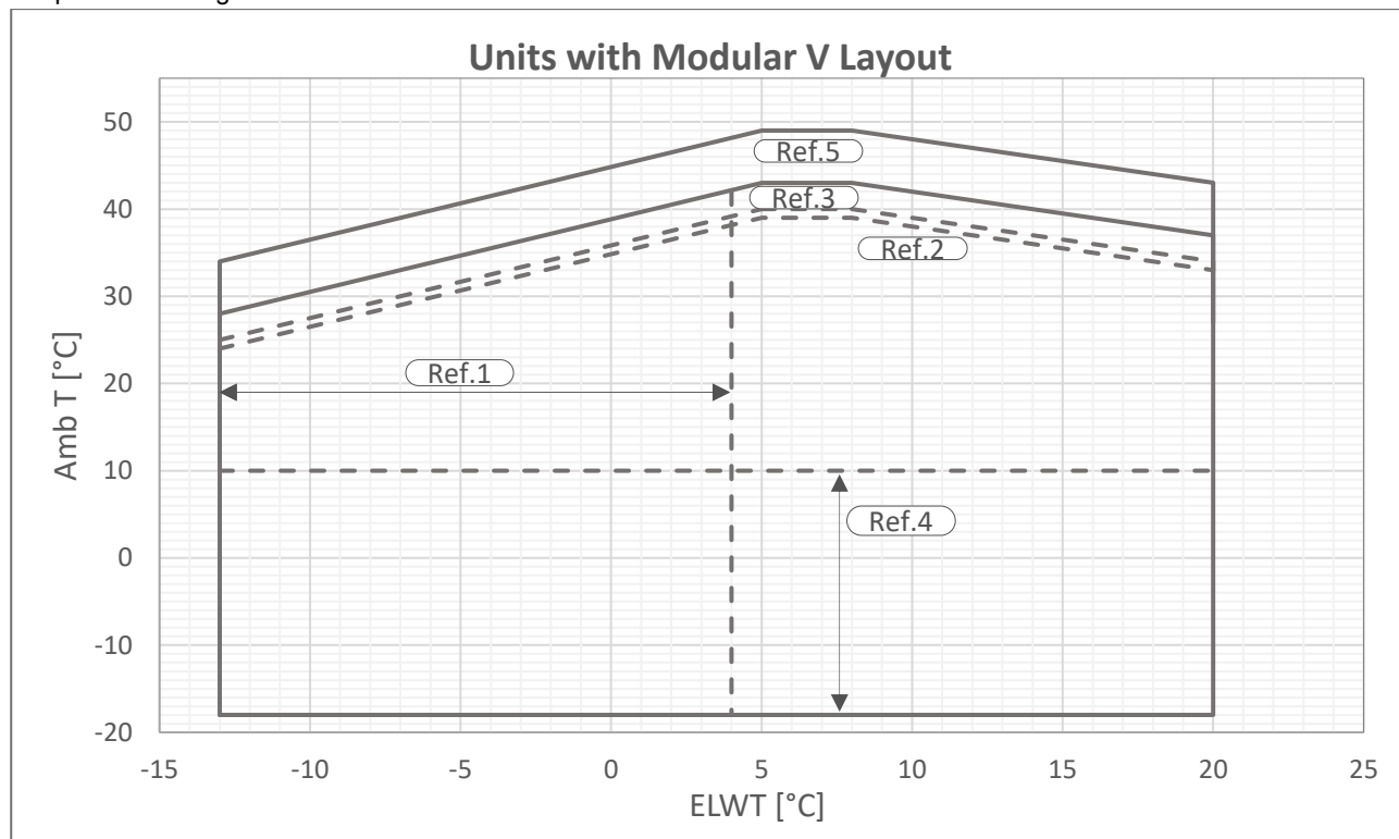
Fig. 9 - Límites operativos de Multi V-Plata
