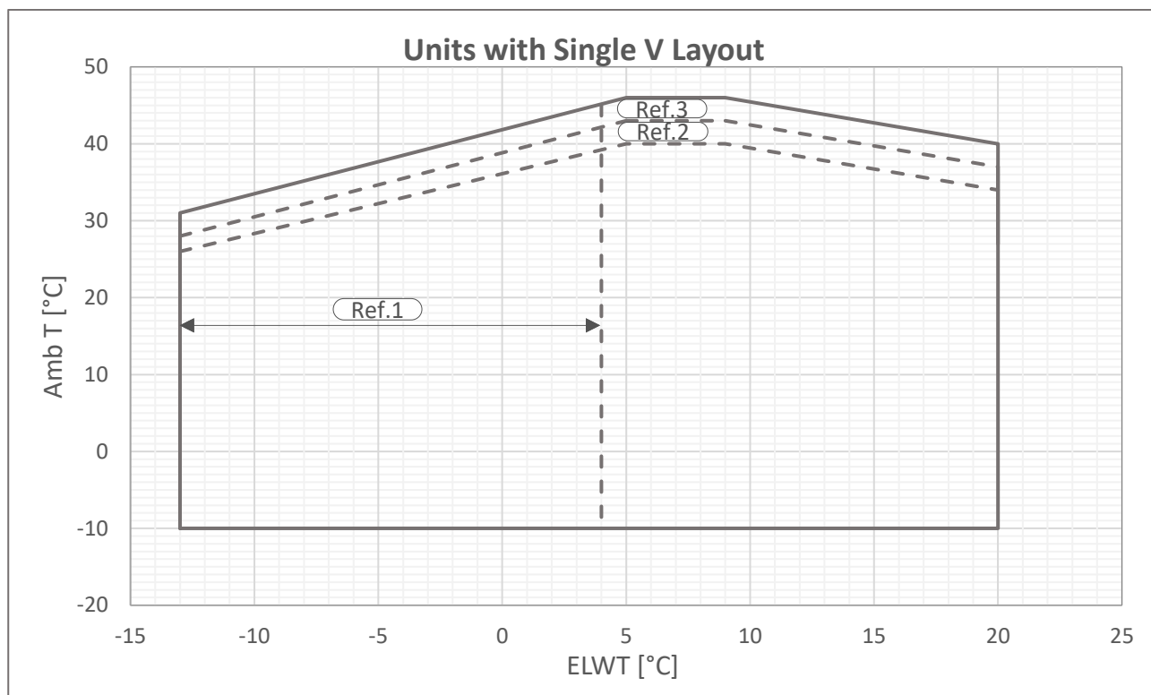
Fig. 12 - Límites operativos de Mono V-Oro
