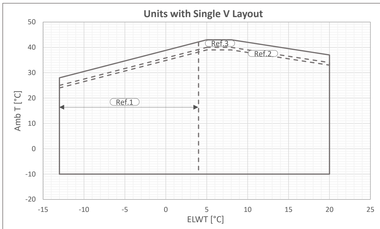
Fig. 11 - Limites opérationnelles Single V-Silver
