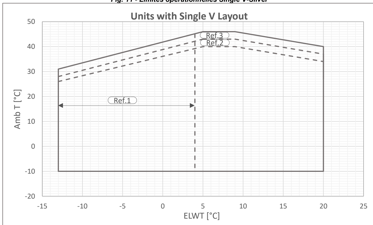
Fig. 12 - Limites opérationnelles Single V-Gold
