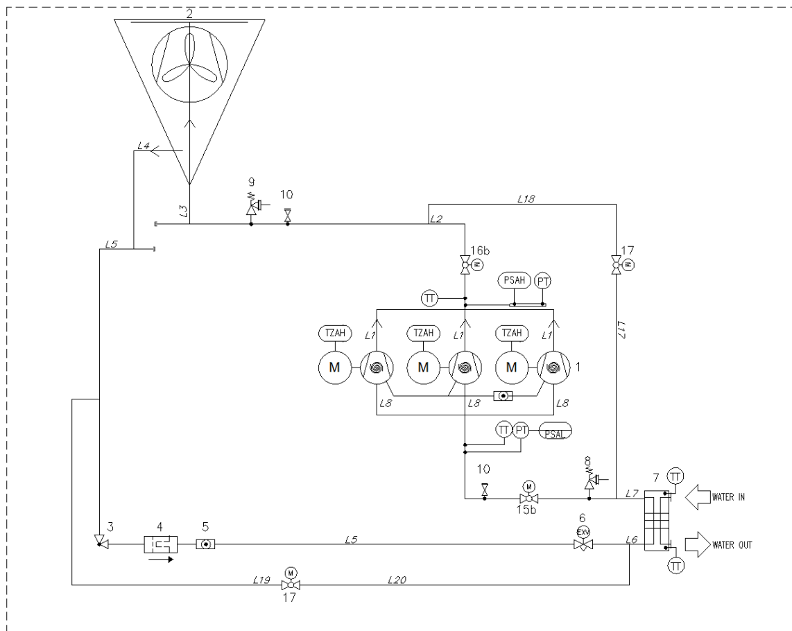
Fig. 14 - Schéma du circuit réfrigérant (P & ID) unité à circuit unique
