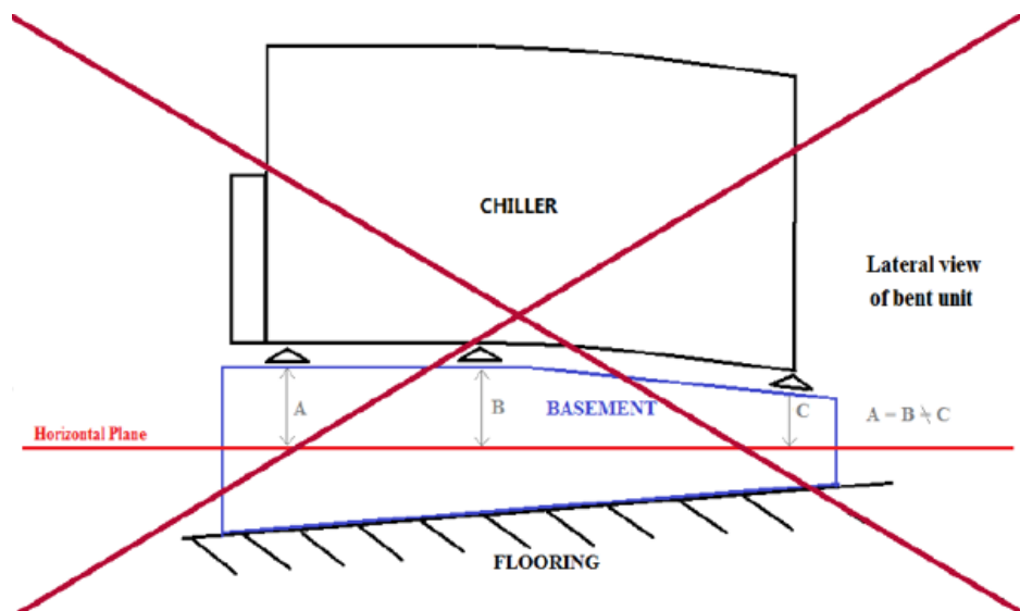
Slika 2 – Niveliranje jedinice
