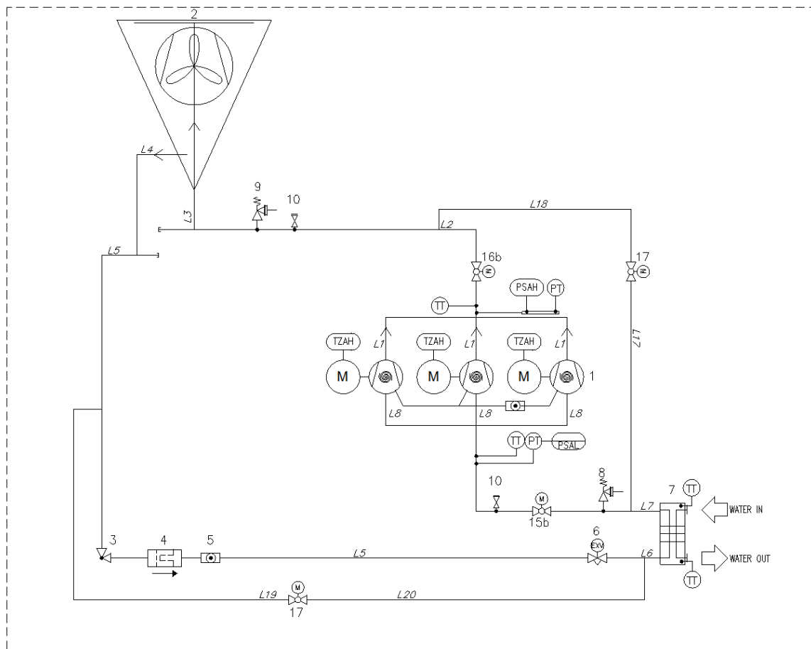
Fig. 14 - Schema del circuito del refrigerante (P&ID) con opzione free-cooling leggero dell'unità mono-circuito
