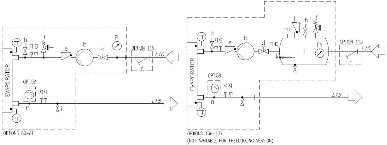
Şekil 7 – Tek V (EWATxx5B) çift pompa için hidrolik diyagram (ops. 80-81/136-137) (maks. çalışma basıncı 6 bar)
