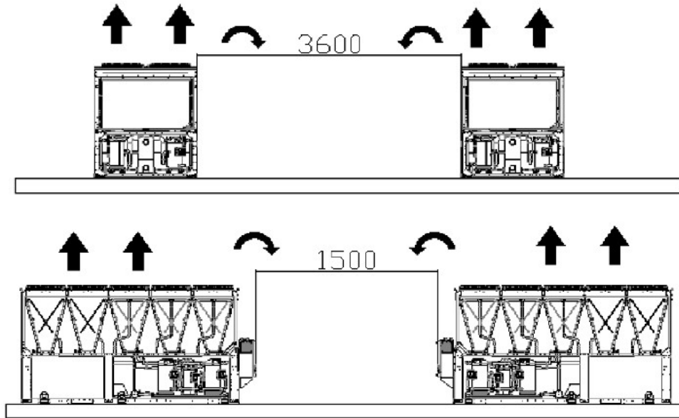
Şek. 3 - Minimum alan gereksinimleri
