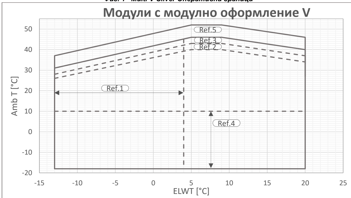
Фиг. 2 –Multi V-Gold Оперативни ограничения
