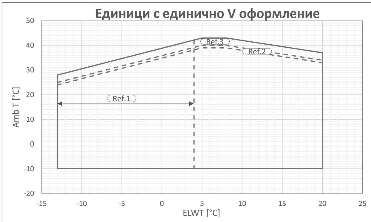
Фиг. 3 –Единични V-Silver Оперативни граници
