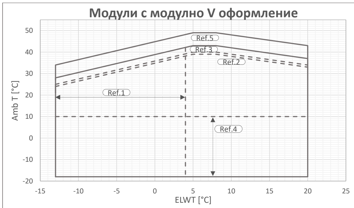
Фиг. 1 –Multi V-Silver Оперативни граници
