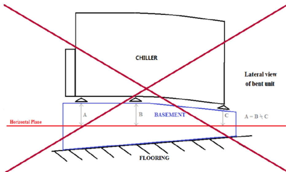
Фиг. 6 – Нивелиране на агрегата
