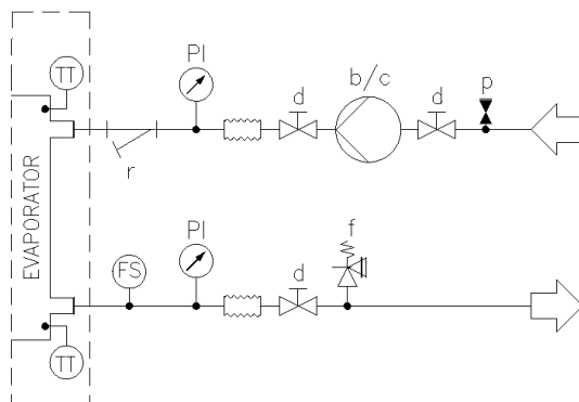
Фиг. 9 – Хидравлична схема без помпа(и) на борда (максимално работно налягане 20 bar)
