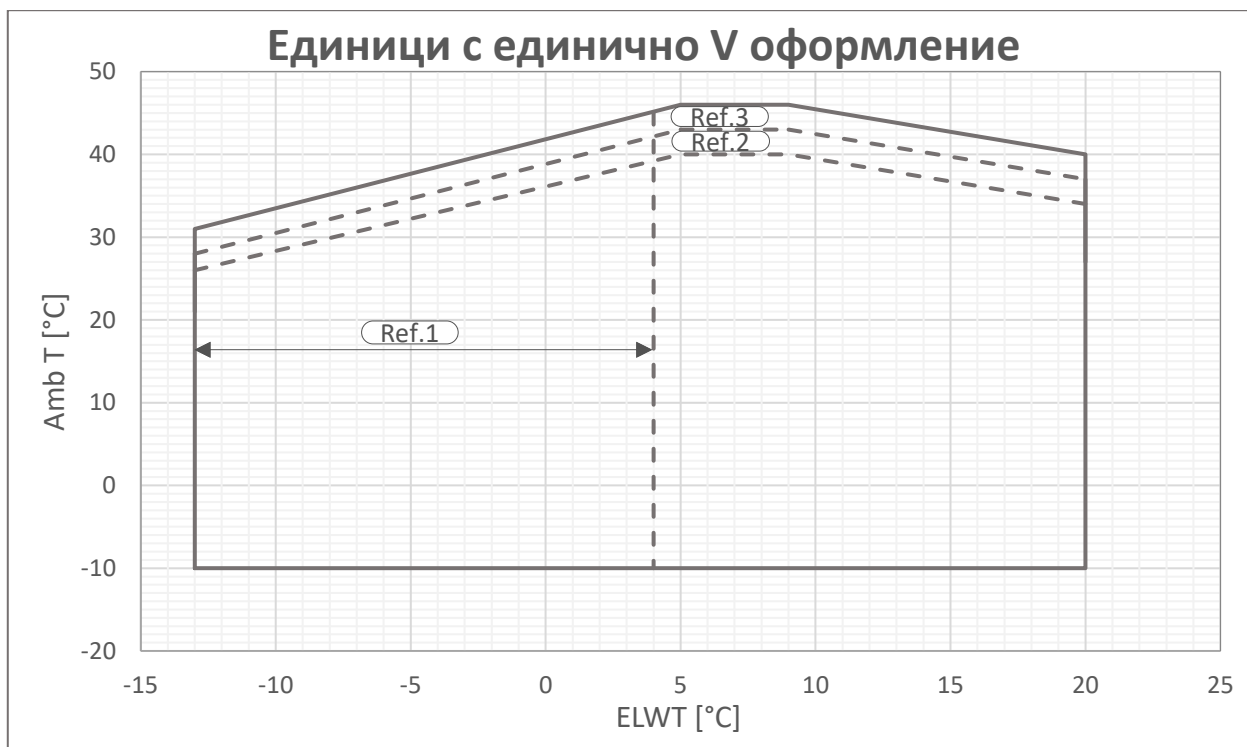
Фиг. 4 –Единични оперативни граници на V-Gold
