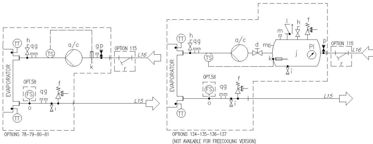
Фиг. 12 – Хидравлична схема за модул V (EWATxx0B) (опт. 78-79-80-81/134-135-136-137) (максимално работно налягане 6 bar)
