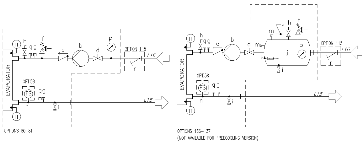
Фиг. 11 – Хидравлична схема за двойна помпа с единична V (EWATxx5B) (опт. 80-81/136-137) (максимално работно налягане 6 bar)
