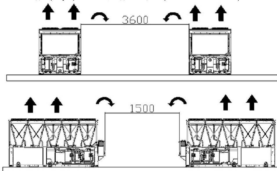
Фиг. 7 – Изисквания за минимално пространство
