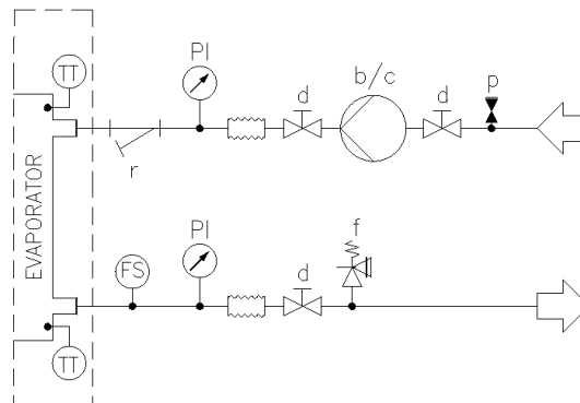
Abb. 8 – Hydraulikschema ohne eingebaute Pumpe(n) (max. Betriebsdruck 20 bar)
