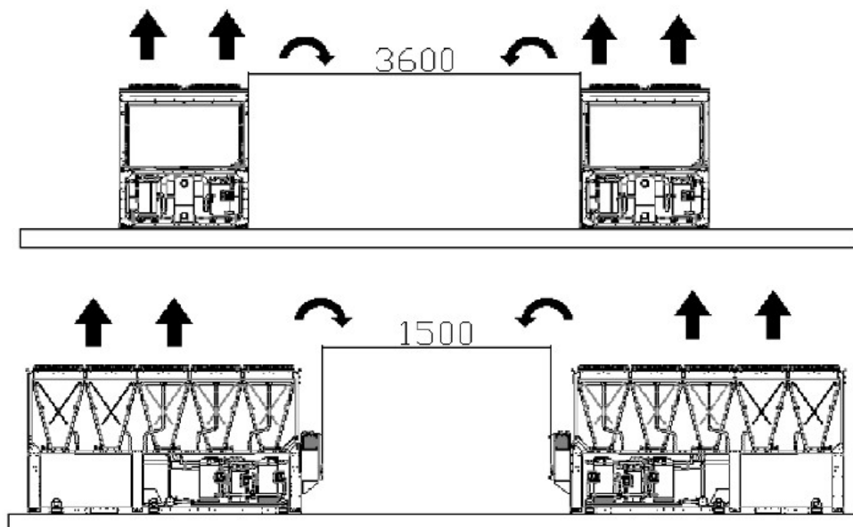
Abb. 6 - Mindestabstände
