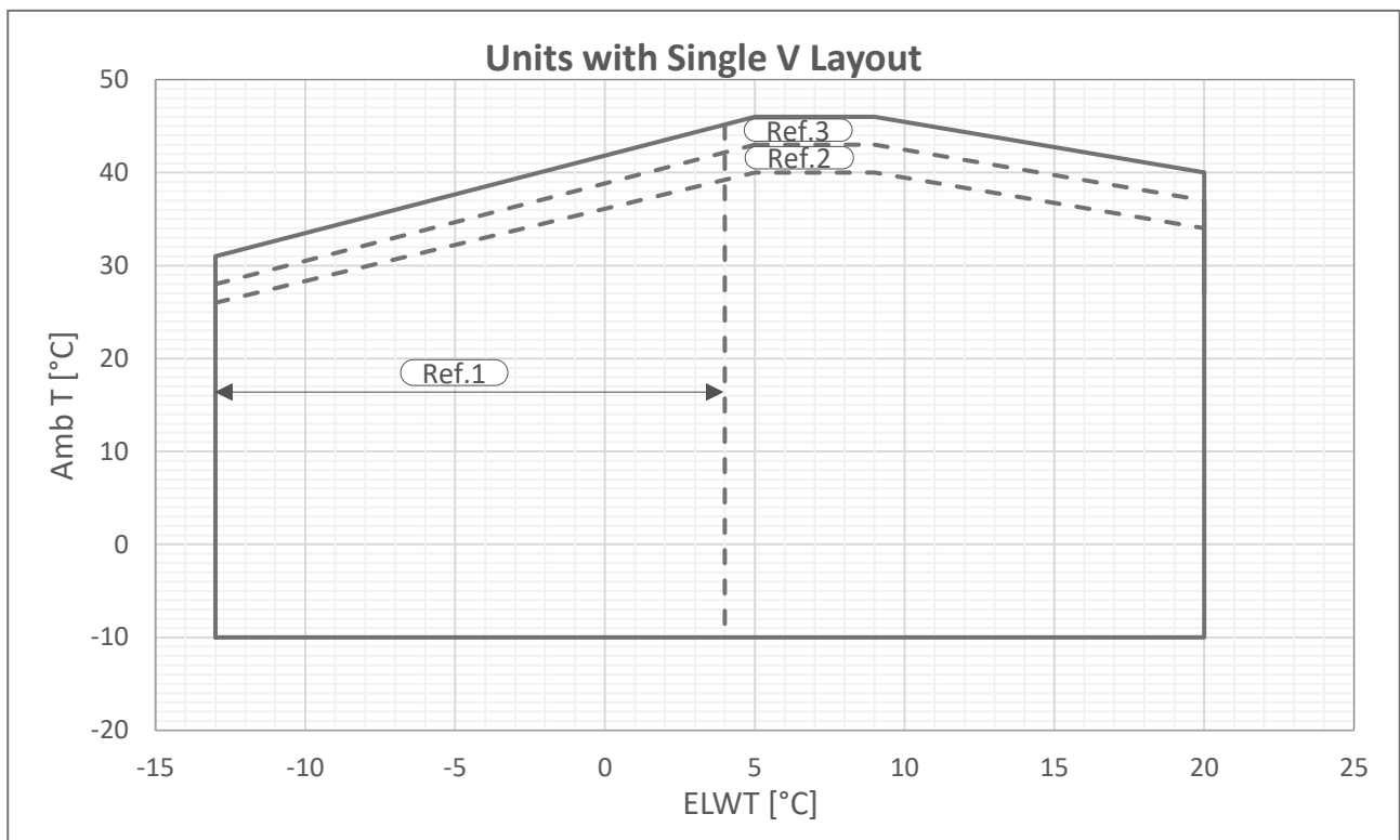
Abb. 3 - Einzelner V-Gold Betriebsgrenzen
