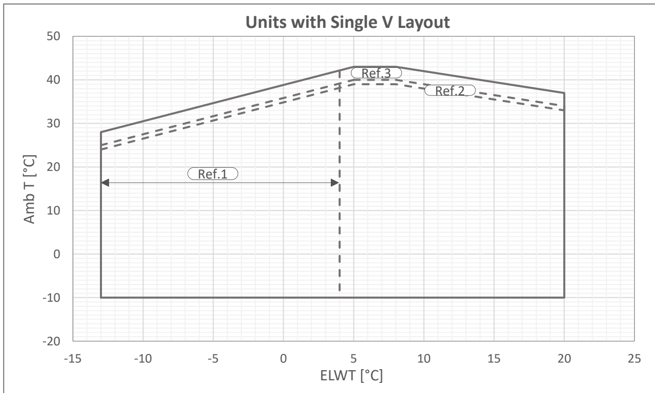
Abb. 1 - Einzelner V-Silber Betriebsgrenzen
