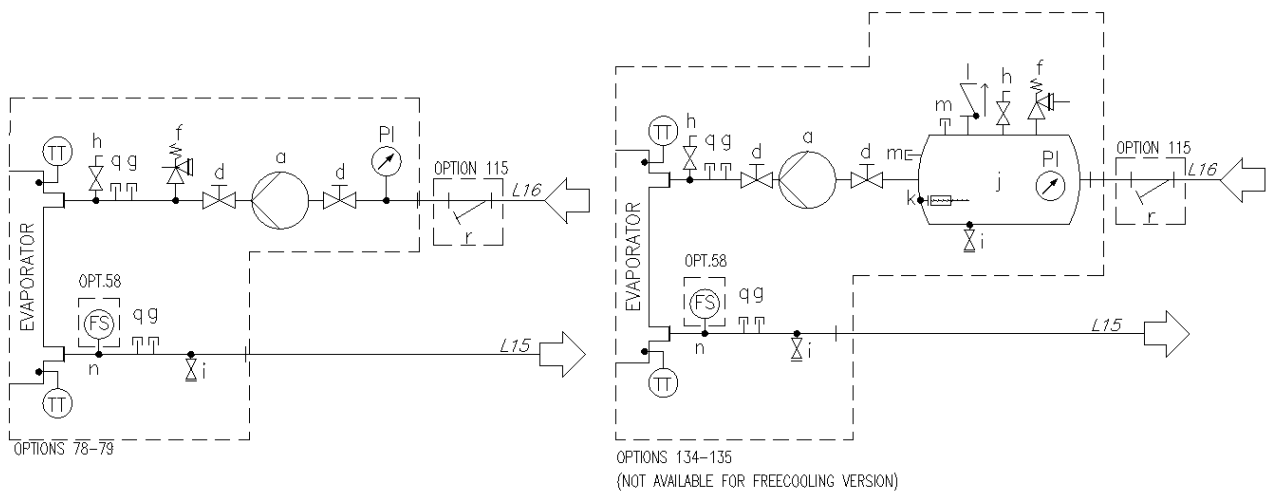
Abb. 9 – Hydraulikschema für einzelne V-Anlage (EWATxx5B) einfache Pumpe (Opt. 78-79/134-135) (max. Betriebsdruck 6 bar)
