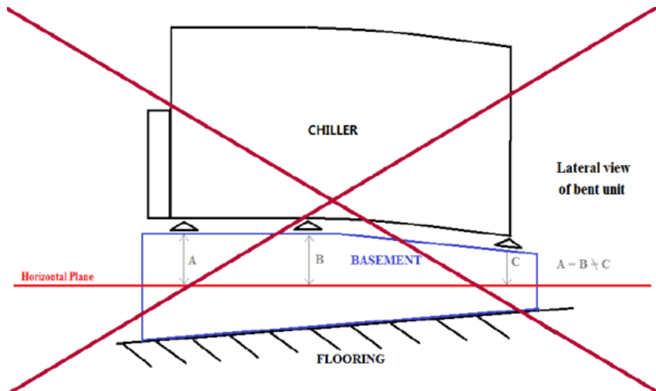
Abb. 5 - Ausrichtung der Einheit
