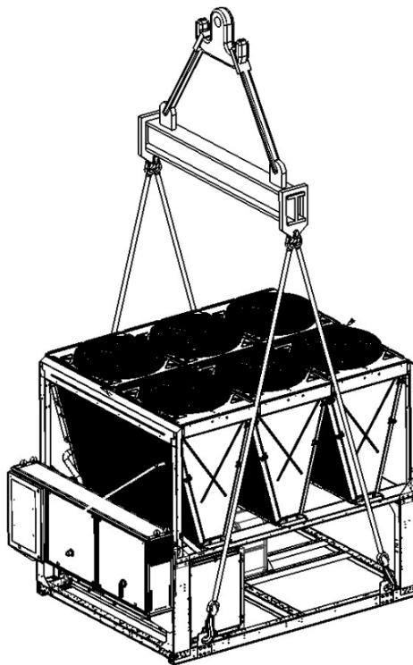
Einheit mit 4 Hebepunkten
