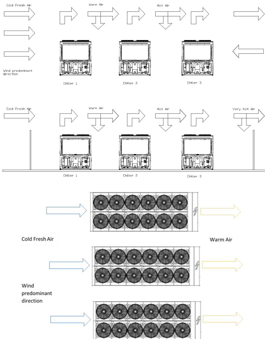
Abb. 7 – Reiheninstallation mehrerer Chiller
