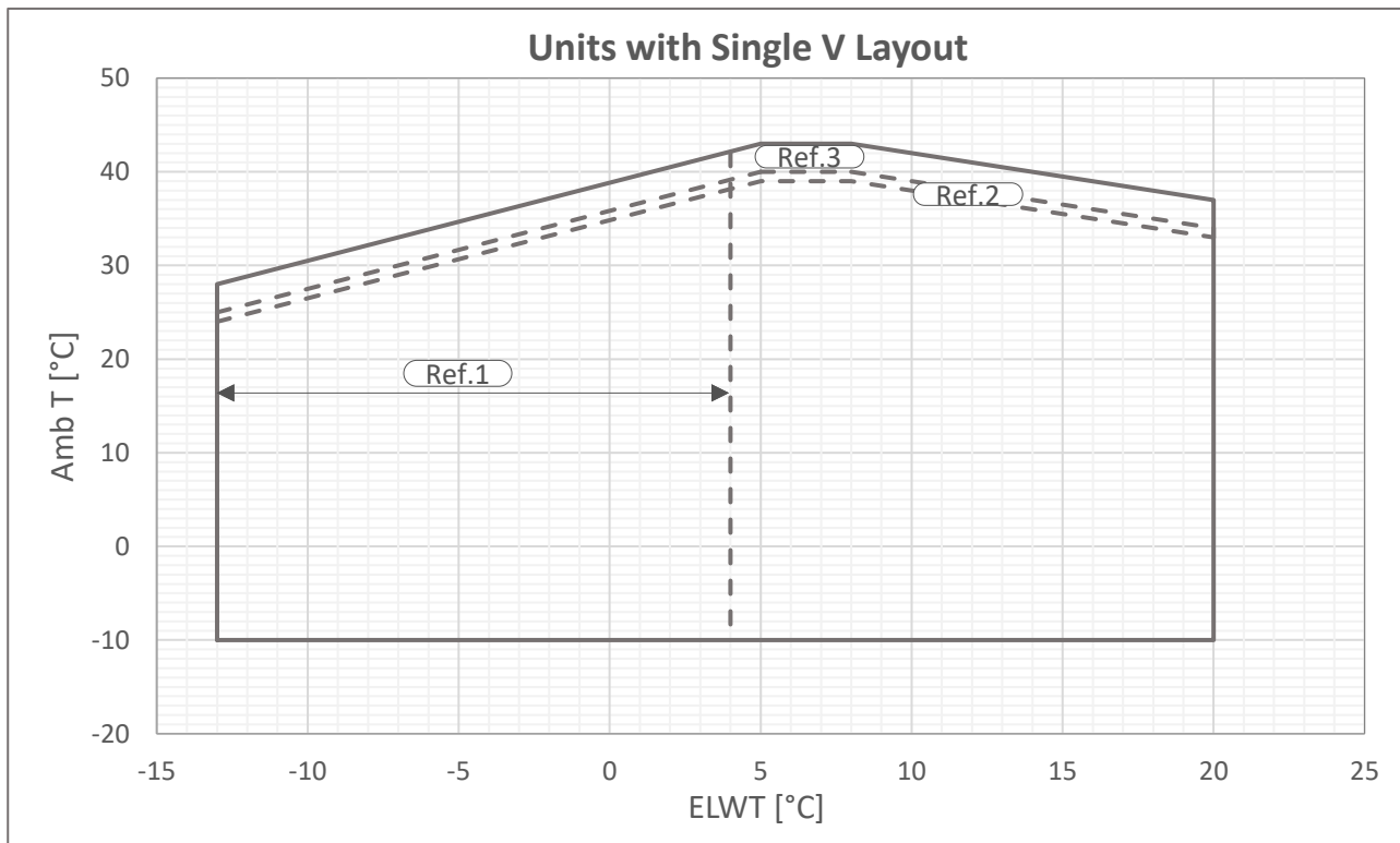
Εικ. 3 – Μονό V - Όρια λειτουργίας Silver
