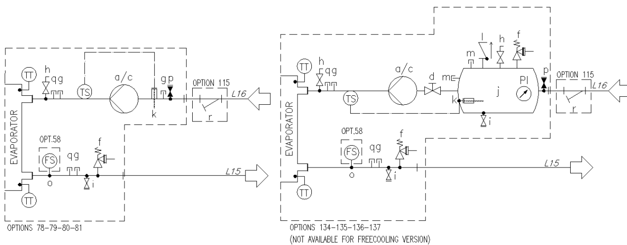
Εικ. 12 – Διάγραμμα υδραυλικού κυκλώματος για Αρθρωτό V (EWATxx0B) (επιλογές 78-79-80-81/134-135-136-137) (μέγιστη πίεση λειτουργίας 6 bar)
