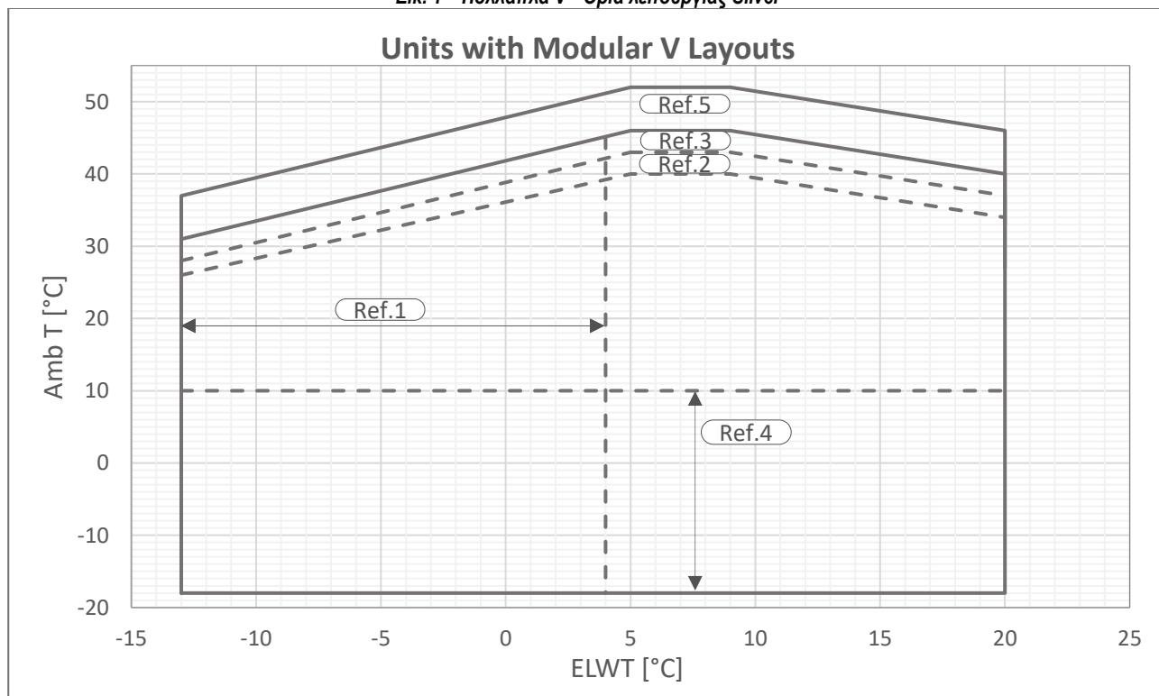
Εικ. 2 – Πολλαπλά V - Όρια λειτουργίας Gold
