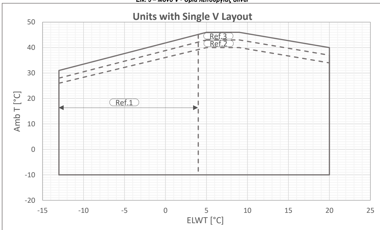
Εικ. 4 – Μονό V - Όρια λειτουργίας Gold
