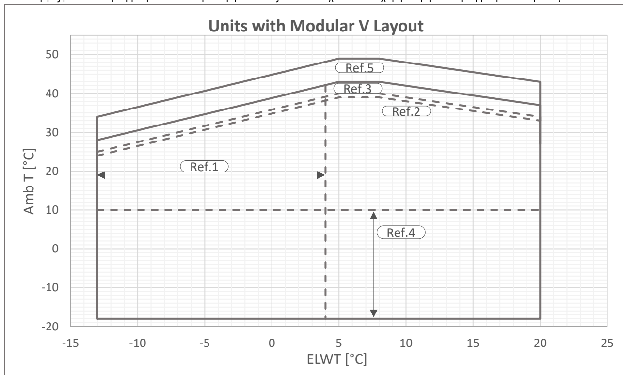
Εικ. 1 – Πολλαπλά V - Όρια λειτουργίας Silver
