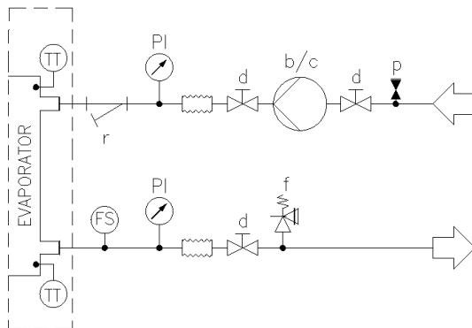
Εικ. 9 – Διάγραμμα υδραυλικού κυκλώματος χωρίς ενσωματωμένες αντλίες (μέγιστη πίεση λειτουργίας 20 bar)
