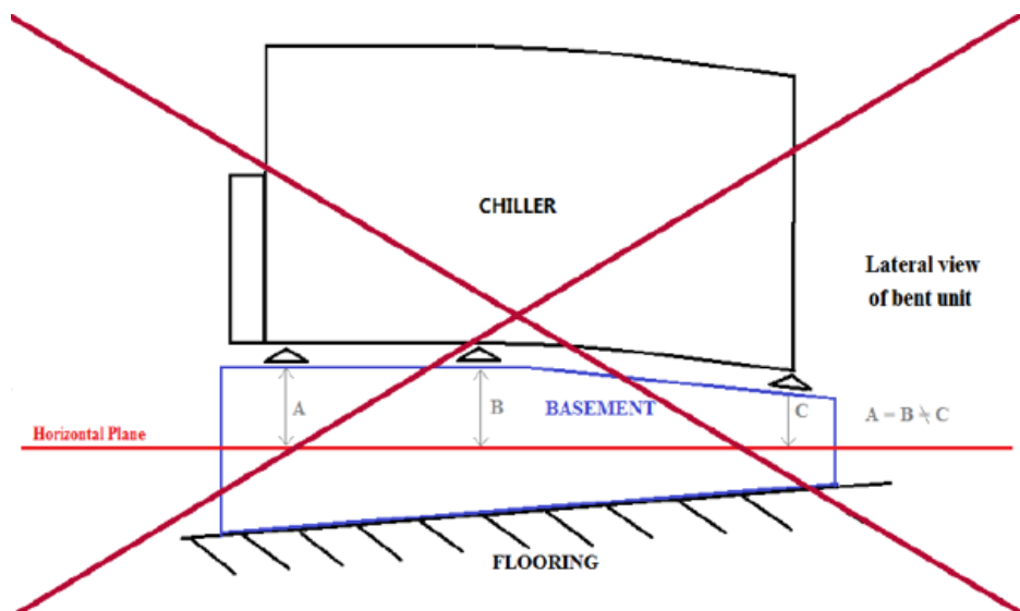
Εικ. 6 – Οριζοντίωση μονάδας
