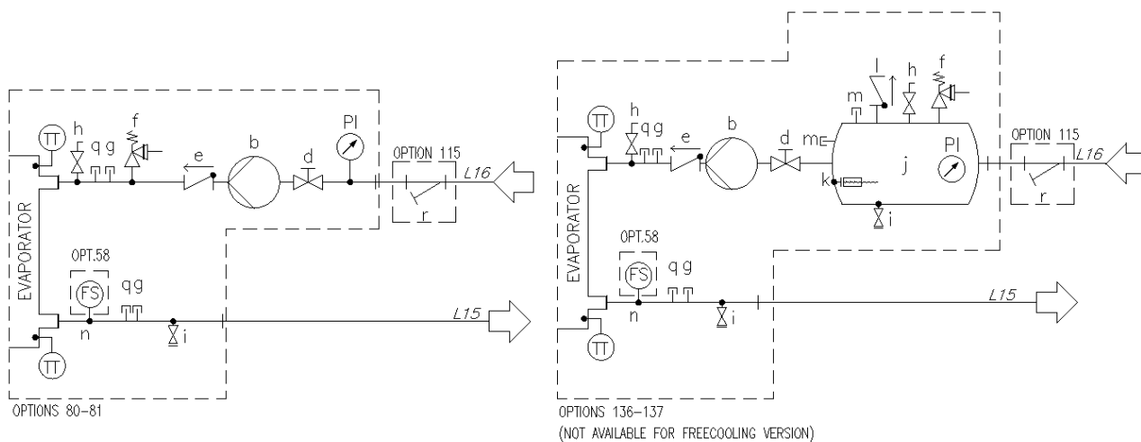
Εικ. 11 – Διάγραμμα υδραυλικού κυκλώματος για διπλή αντλία μονού V (EWATxx5B) (επιλογές 80-81/136-137) (μέγιστη πίεση λειτουργίας 6 bar)
