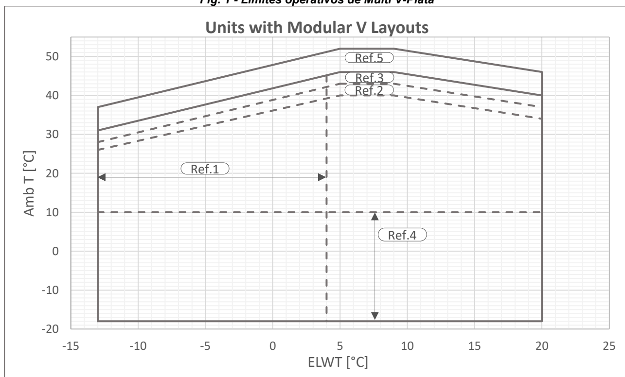
Fig. 2 - Límites operativos de Multi V-Oro
