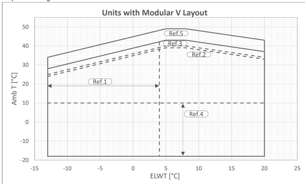
Fig. 1 - Límites operativos de Multi V-Plata
