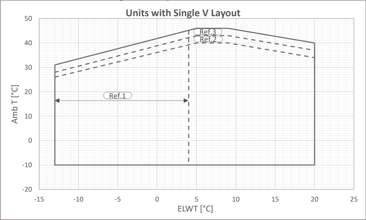
Fig. 4 - Límites operativos de Mono V-Oro
