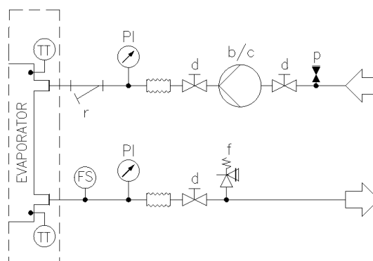
Fig. 9 - Schéma hydraulique sans pompe(s) à bord (pression de fonctionnement max. 20 bar)
