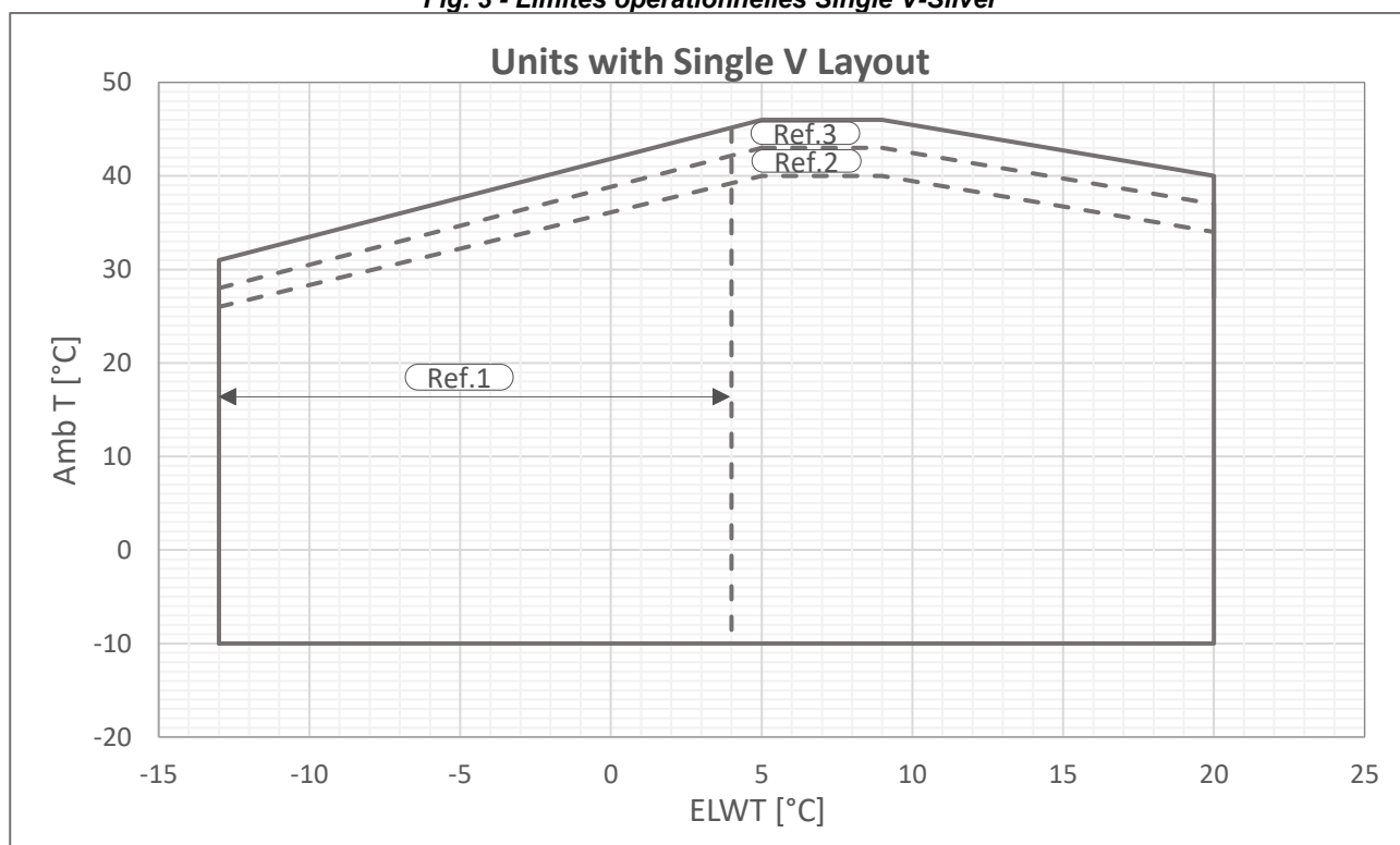
Fig. 4 - Limites opérationnelles Single V-Gold
