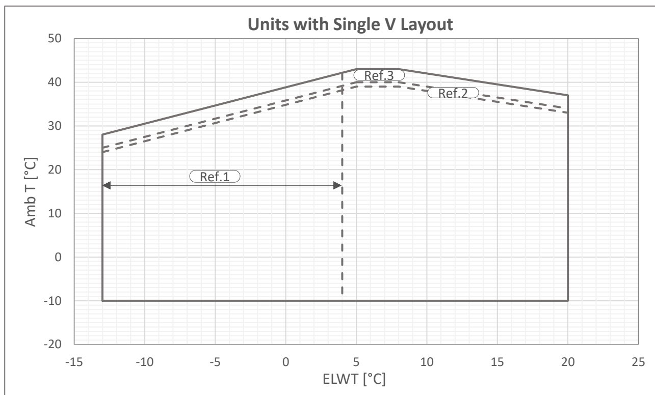
Fig. 3 - Limites opérationnelles Single V-Silver
