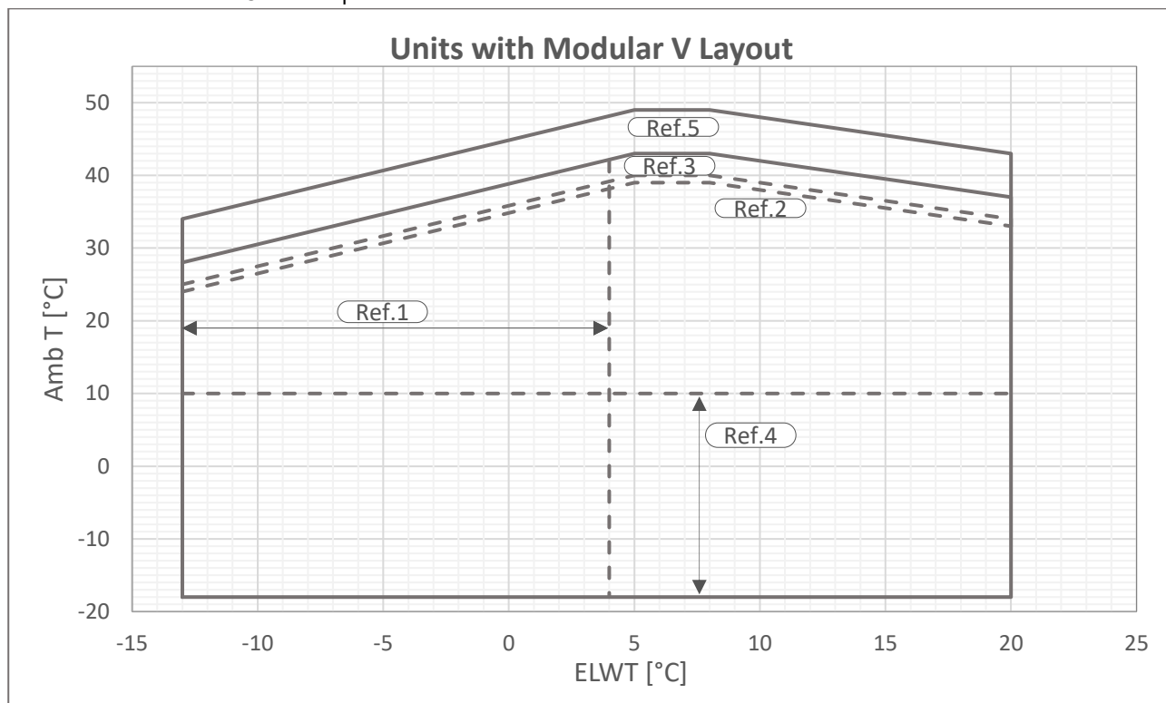
Fig. 1 - Limites opérationnelles Multi V-Silver
