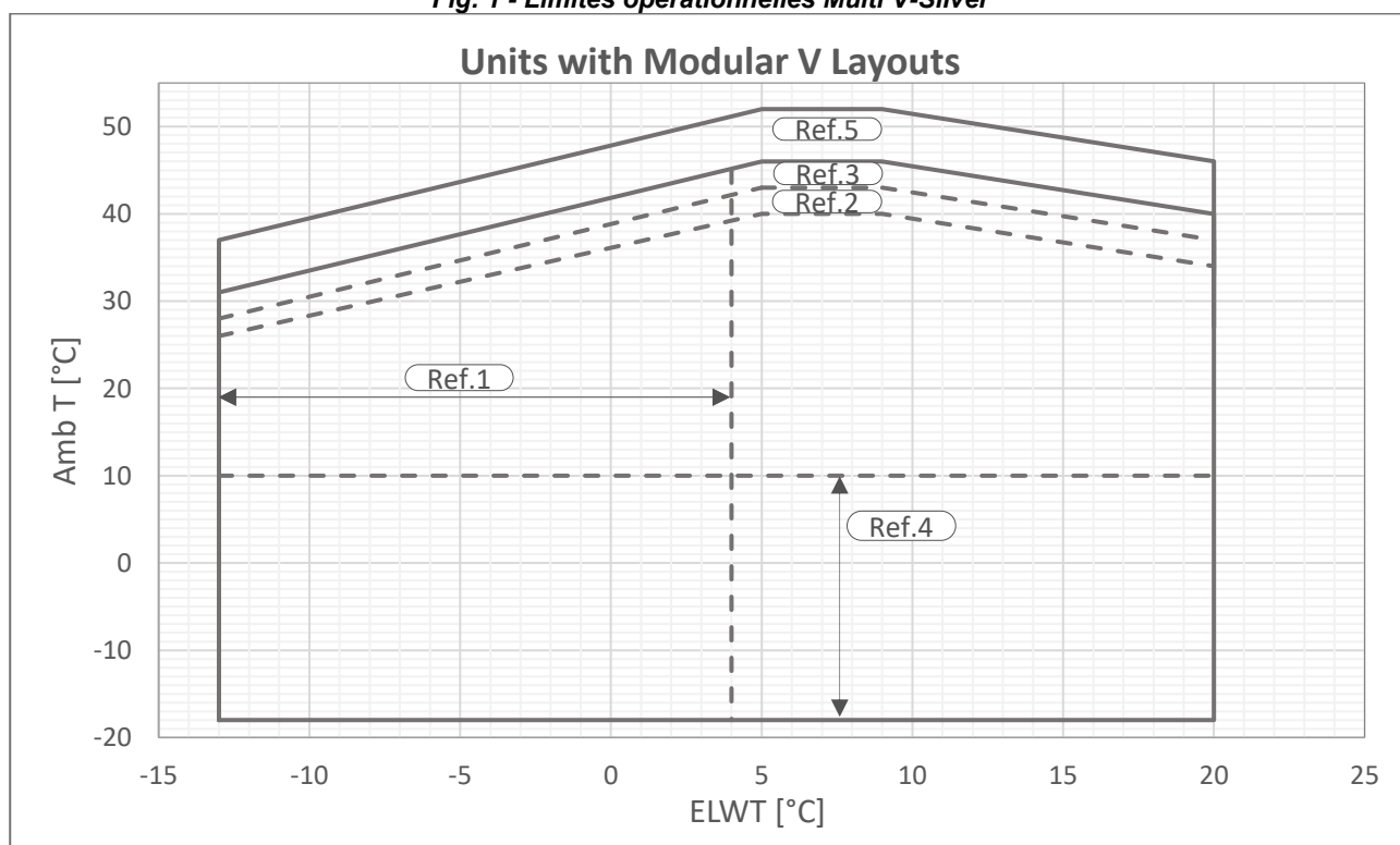
Fig. 2 - Limites opérationnelles Multi V-Gold
