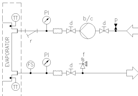
Slika 9 – Hidraulički dijagram bez ugrađenih pumpi (maks. radni tlak 20 bara)
