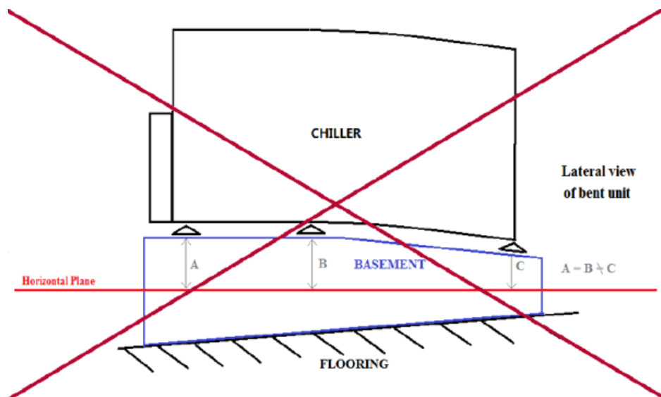
Slika 6 – Niveliranje jedinice
