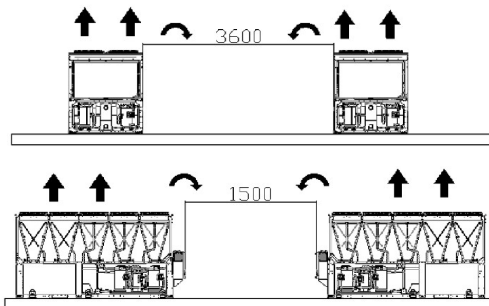
Slika 7 – Minimalni zahtjevi za prostor
