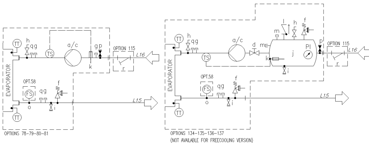
Slika 12 – Hidraulički dijagram za Modular V (EWATxx0B) (opc. 78-79-80-81/134-135-136-137) (maks. radni tlak 6 bara)
