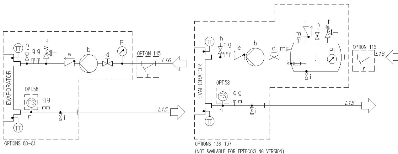
Slika 11 – Hidraulički dijagram za single V (EWATxx5B) dvostruku pumpu (opt. 80-81/136-137) (maks. radni tlak 6 bara)
