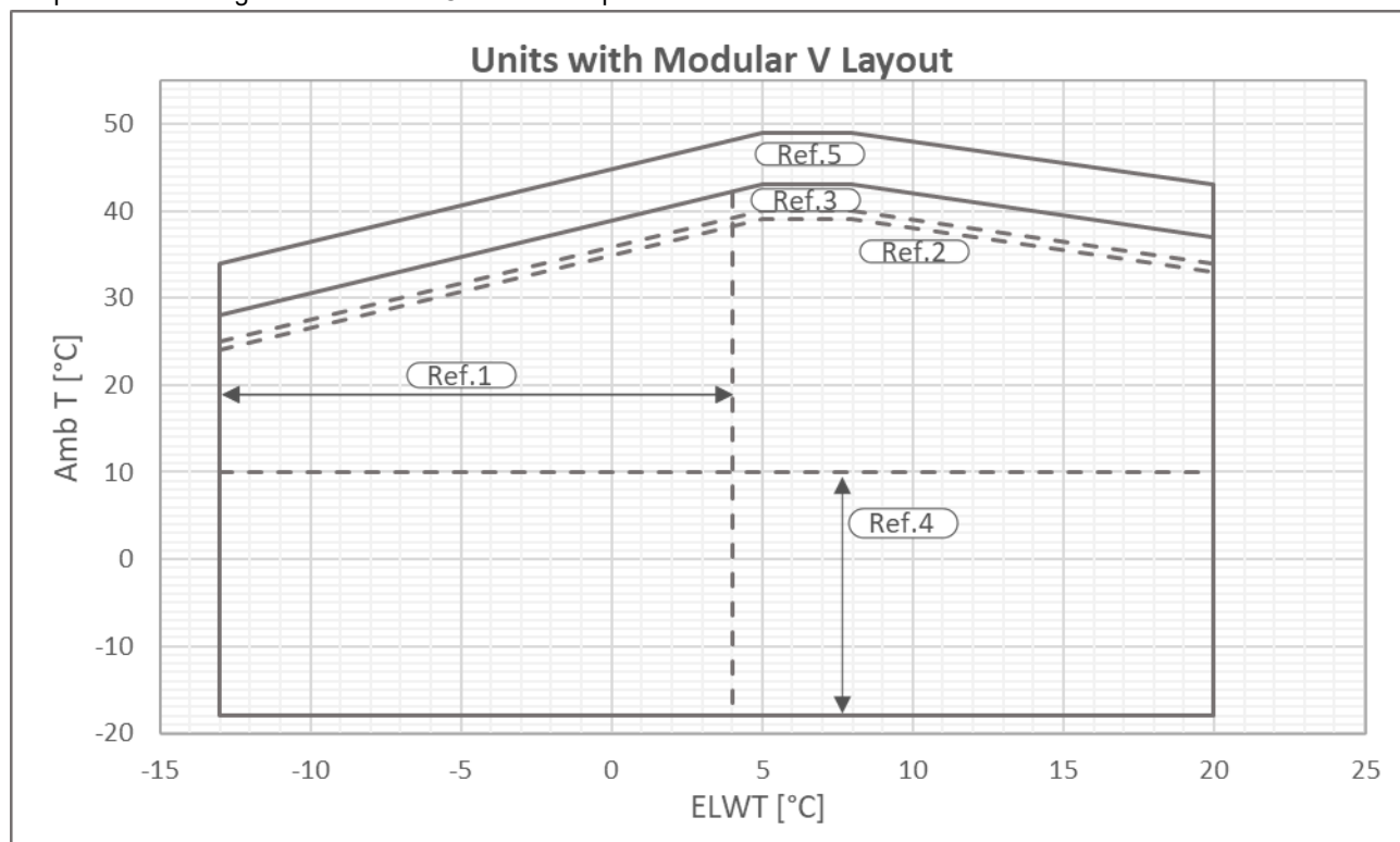
Slika 1 – Višestruke V-srebrna radna ograničenja
