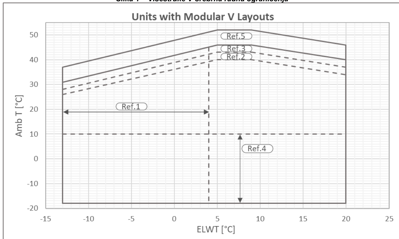
Slika 2 – Višestruka V-zlatna radna ograničenja
