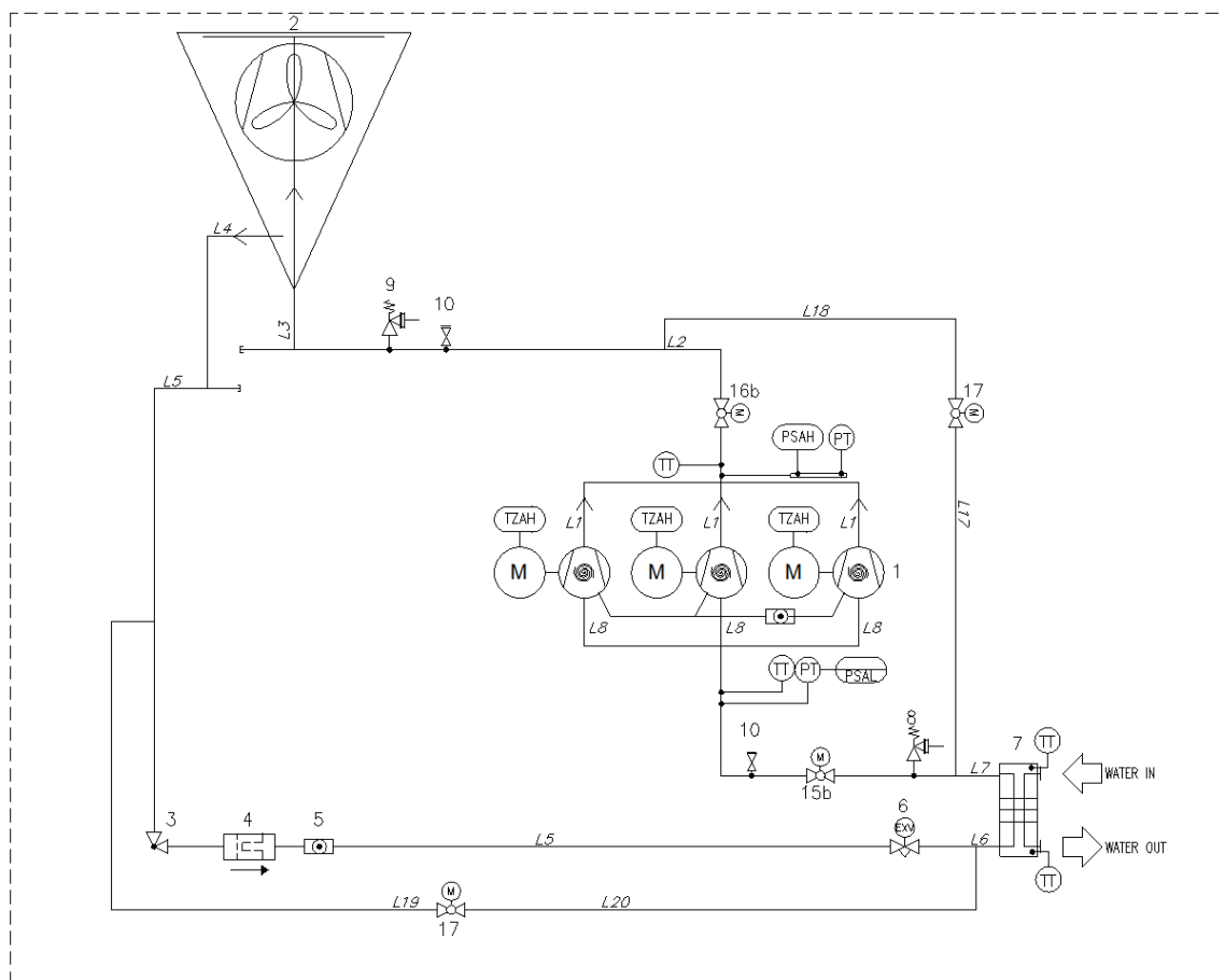
Slika 14 – Dijagram rashladnog kruga (P&ID) s jednokružnom jedinicom s opcijom laganog slobodnog hlađenja
