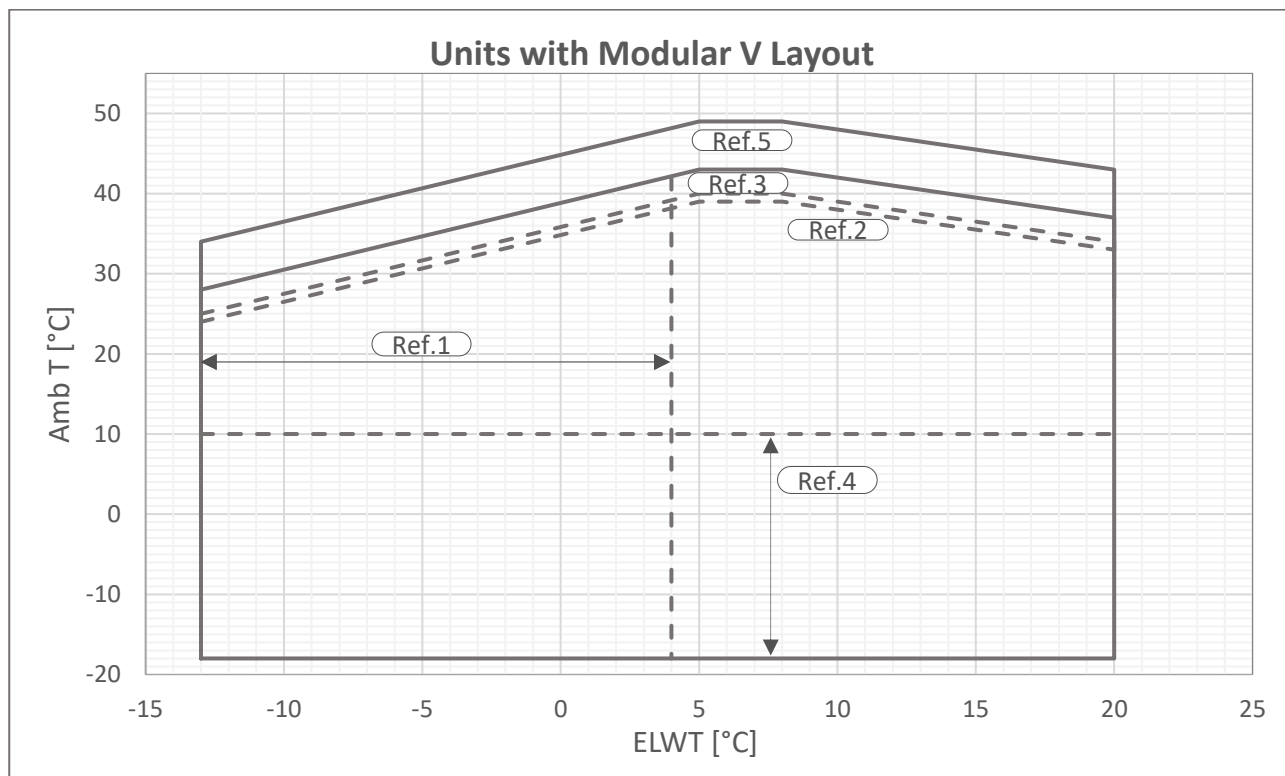
1. ábra - Több ventilátoros V-Silver egység üzemi tartományai
