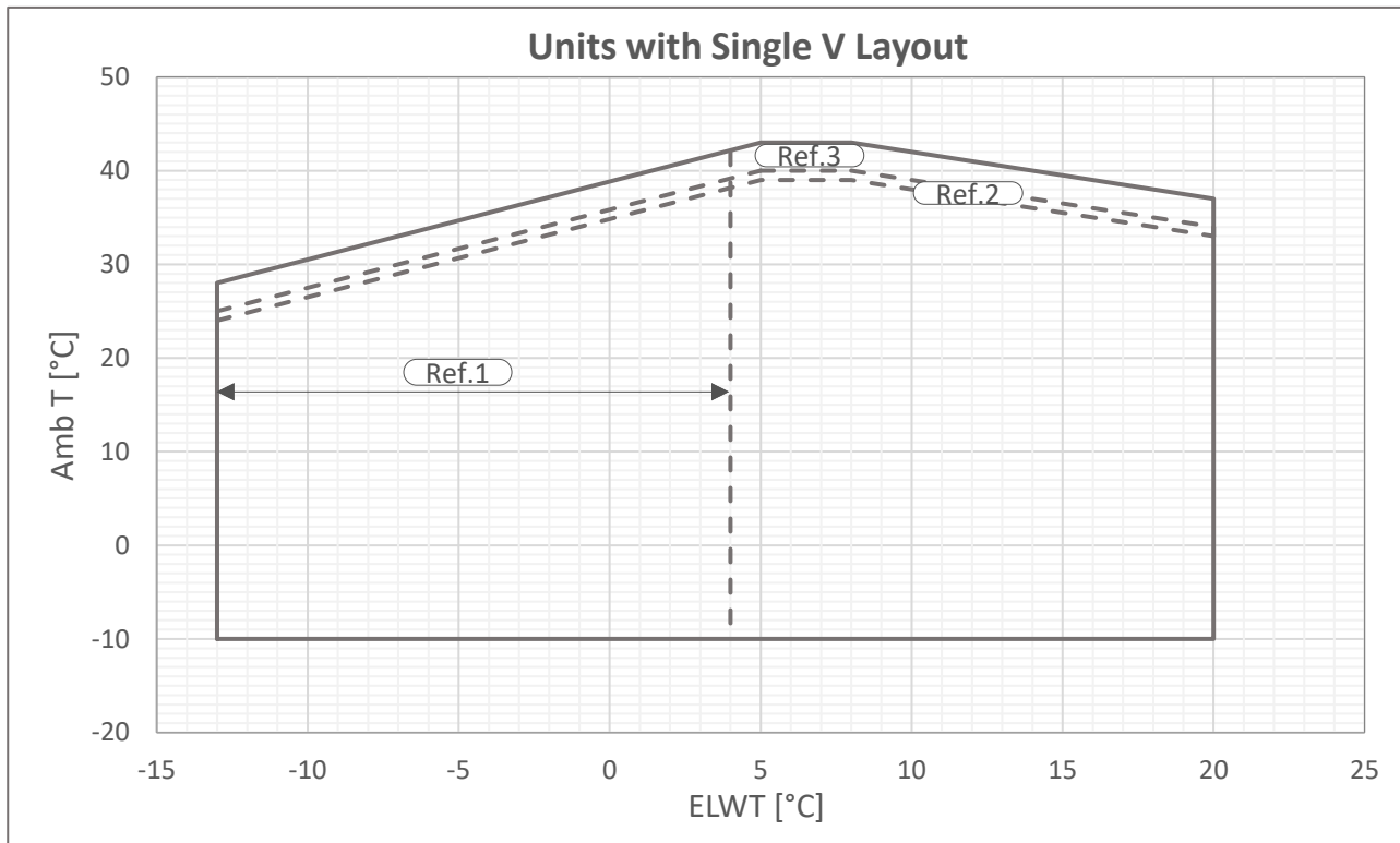
3. ábra - Egy ventilátoros V-Silver egység üzemi tartományai
