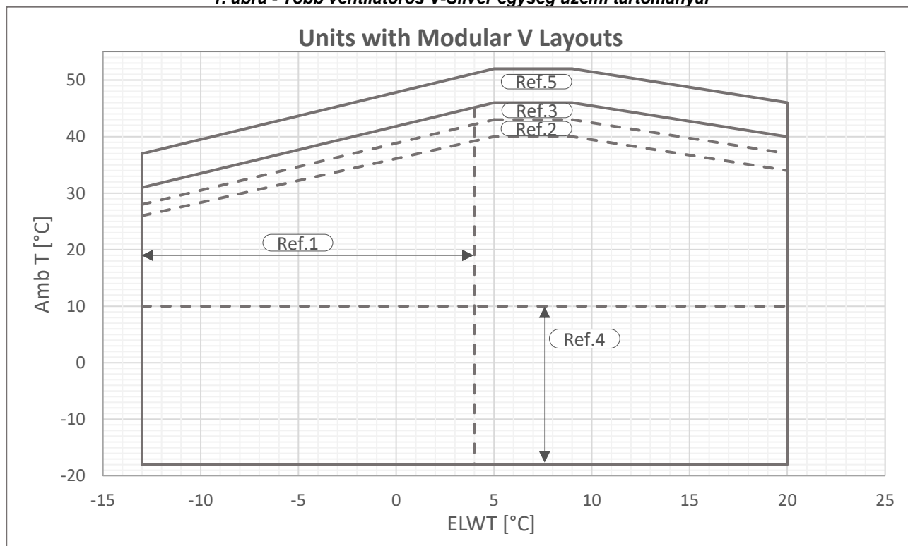
2. ábra - Több ventilátoros V-Gold egység üzemi tartományai
