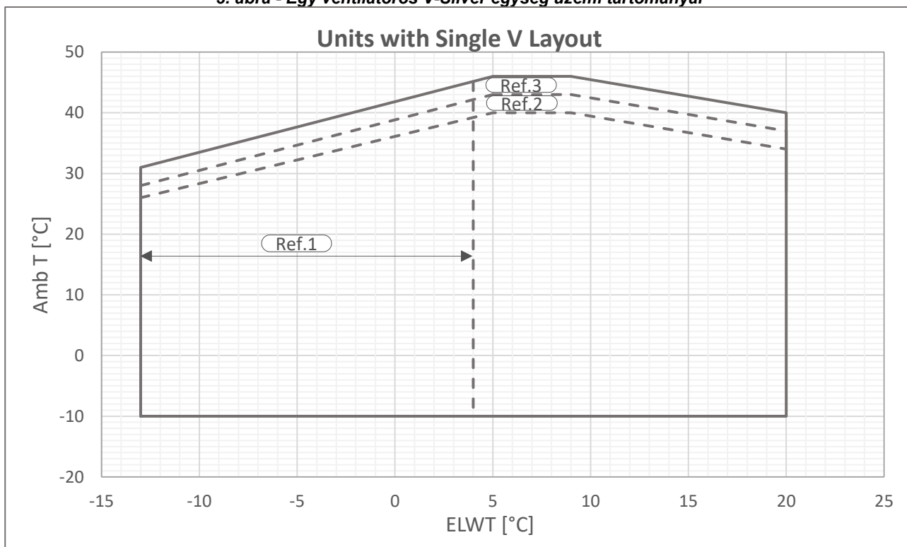
4. ábra - Egy ventilátoros V-Gold egység üzemi tartományai
