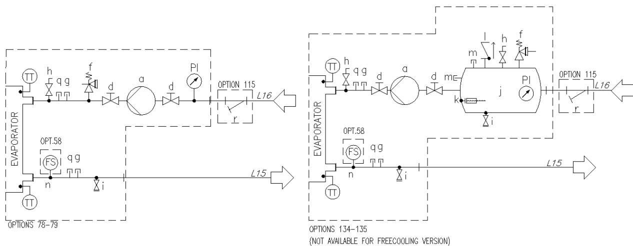
10 pav. – Vieno siurblio V (EWATxx5B) siurblio hidraulikos schema (pas. 78-79/134-135) (maks. darbinis slėgis 6 barai)
