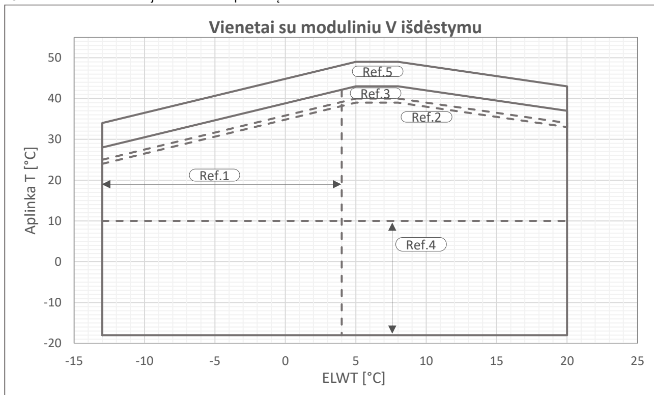
1 pav. – "Multi V-Silver" veikimo ribos
