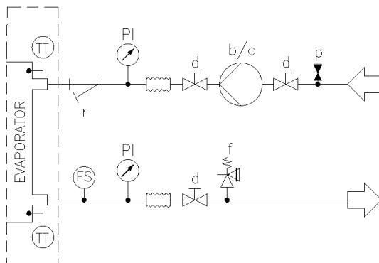
9 pav. – Hidraulinės schema be įrengto siurblio (-ių) (maks. darbinis slėgis 20 barų)
