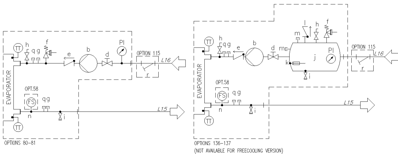
11 pav. – Vieno siurblio V (EWATxx5B) dvigubo siurblio hidraulikos schema (pas. 80-81/136-137) (maks. darbinis slėgis 6 barai)
