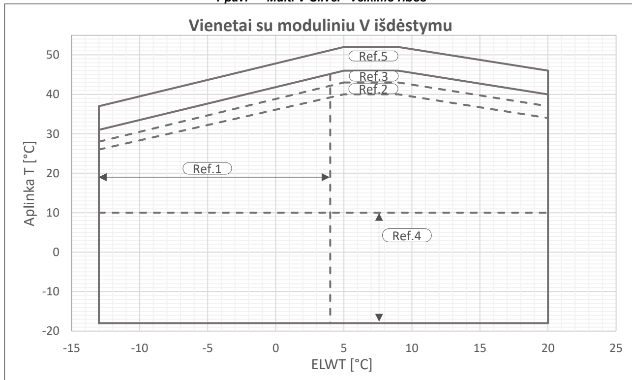
2 pav. – "Multi V-Gold" veikimo ribos
