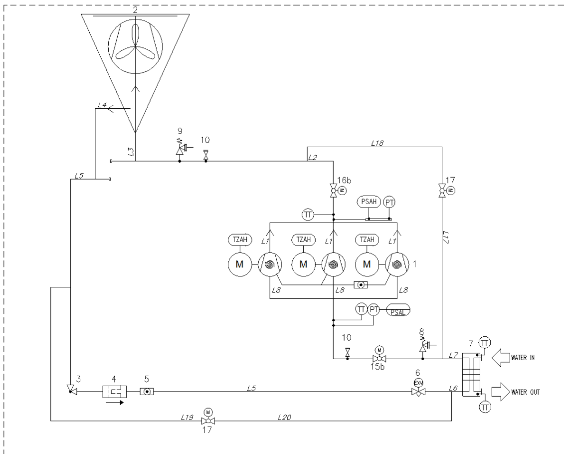
Afb. 14 - Schema koelcircuit (P&ID) systeem enkel circuit en optie light freecooling
