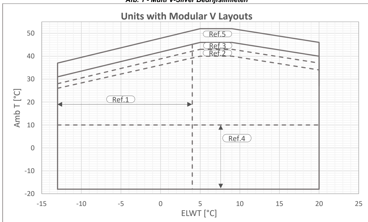
Afb. 2 - Multi V-Gold Bedrijfslimieten
