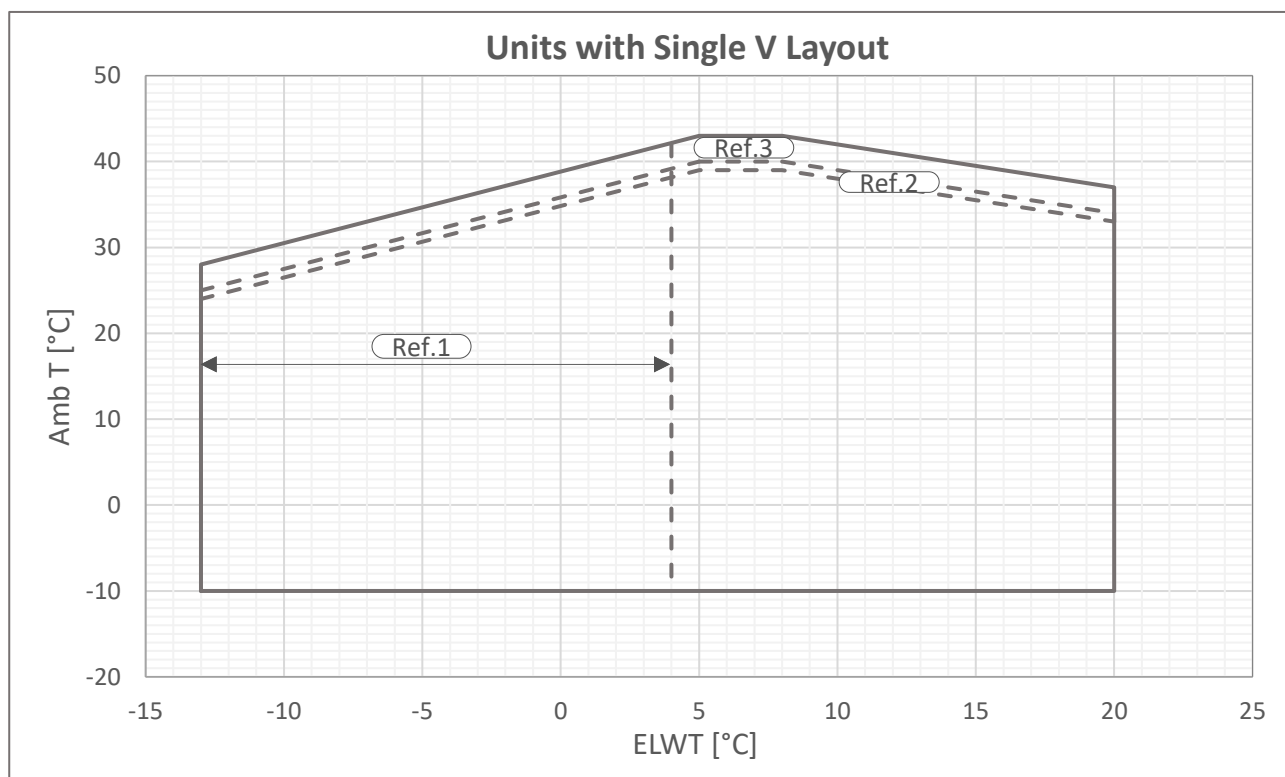
Afb. 3 - Enkele V-Silver Bedrijfslimieten
