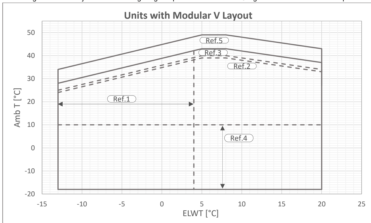
Afb. 1 - Multi V-Silver Bedrijfslimieten
