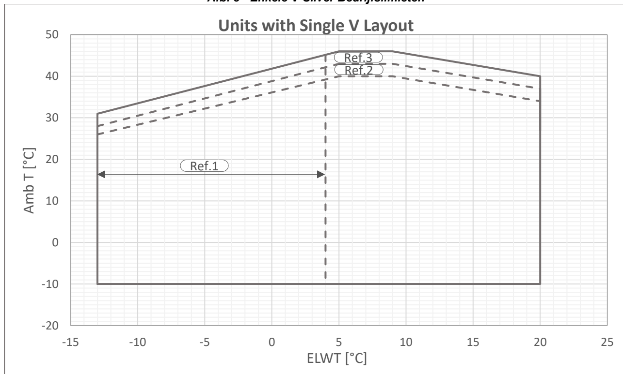
Afb. 4 - Enkele V-Gold Bedrijfslimieten
