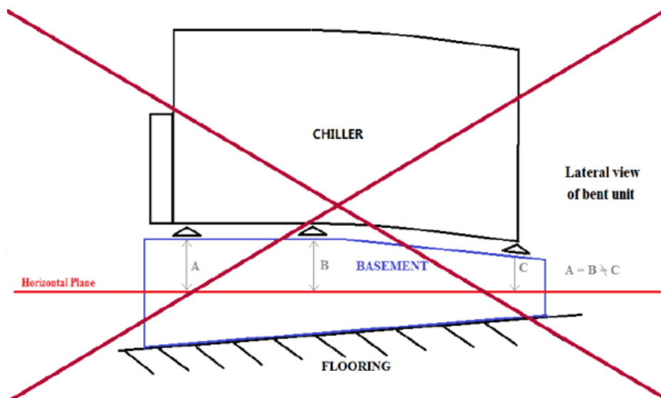
Rys. 6 - Poziomowanie jednostki
