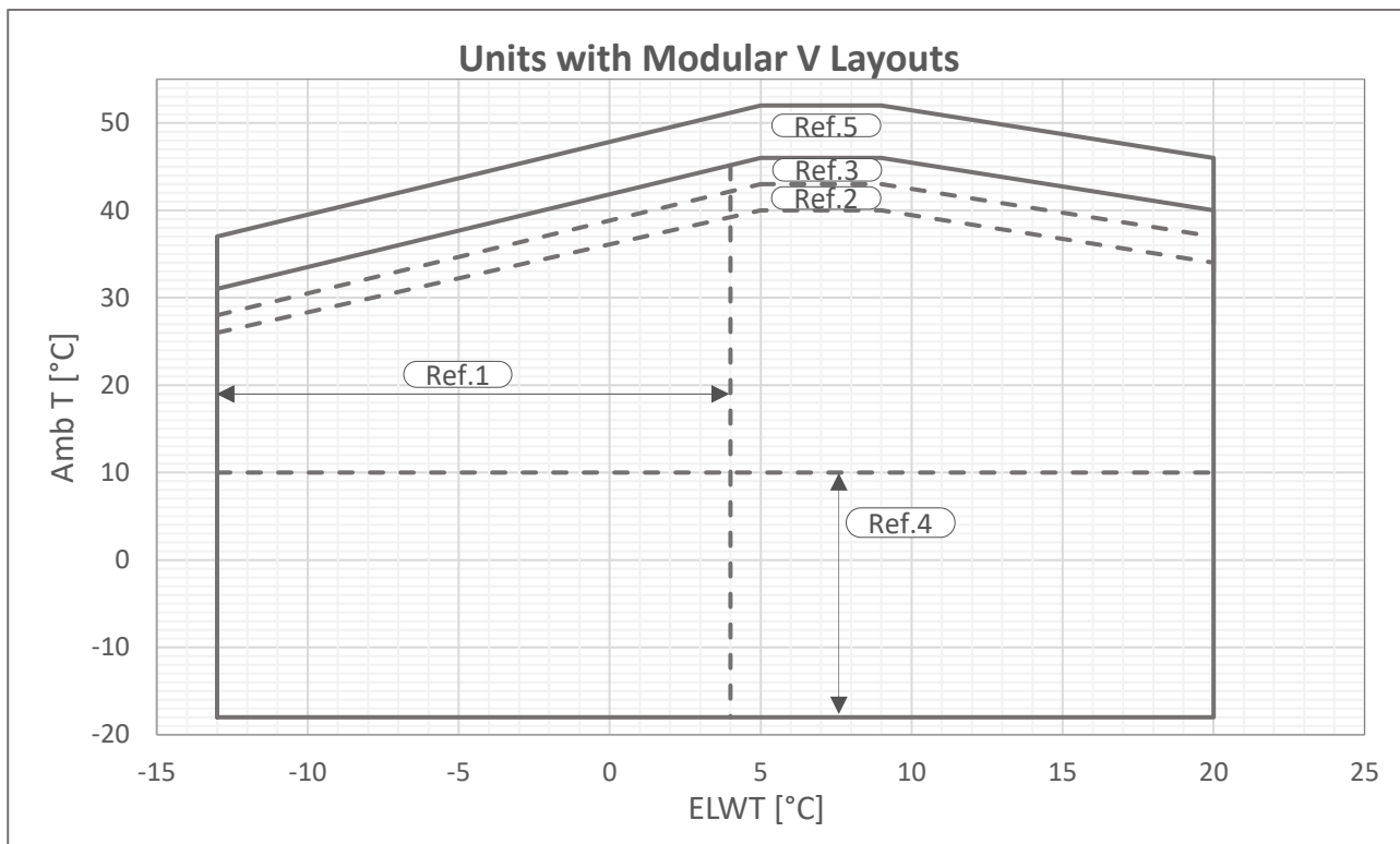
Rys. 2 — Robocze wartości graniczne dla kilku jednostek V-Gold
