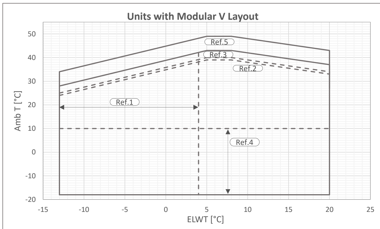
Rys. 1 — Robocze wartości graniczne dla kilku jednostek V-Silver
