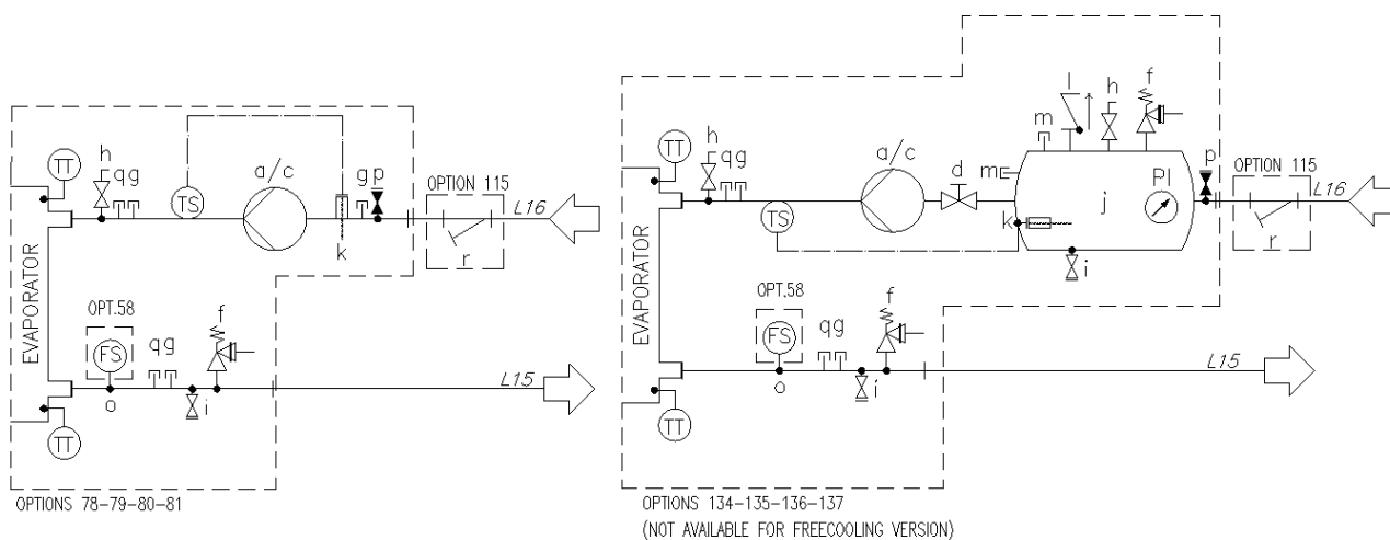
Fig. 12 – Diagrama hidraulică pentru V Modular ( EWATxx0B) (opț. 78-79-80-81/134-135-136-137) (presiune max. de operare 6 bari)
