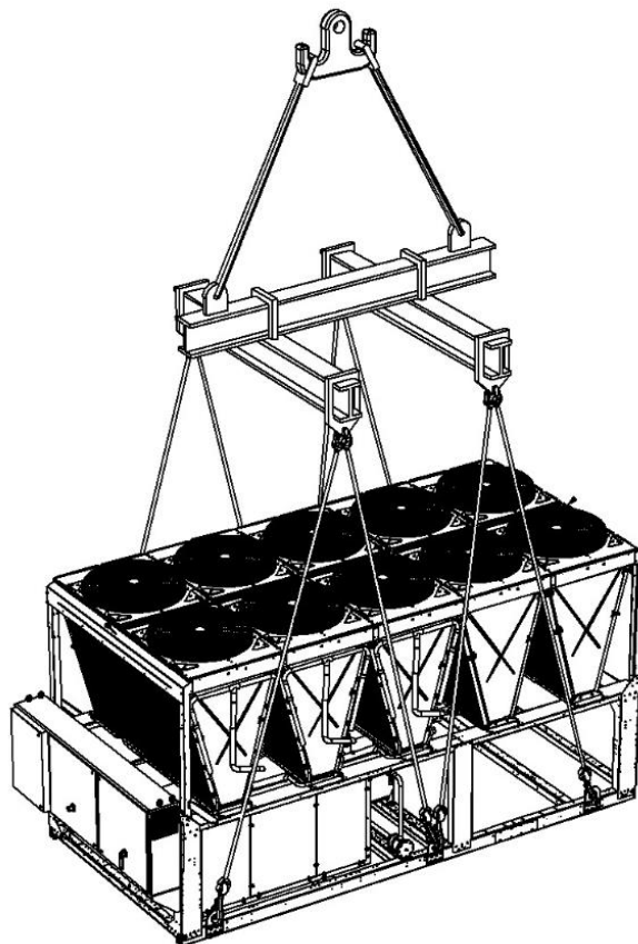
Unitate cu 6 puncte de ridicare
