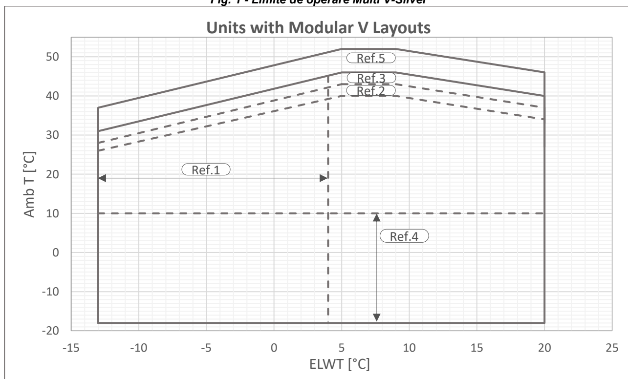
Fig. 2 - Limite de operare Multi V-Gold
