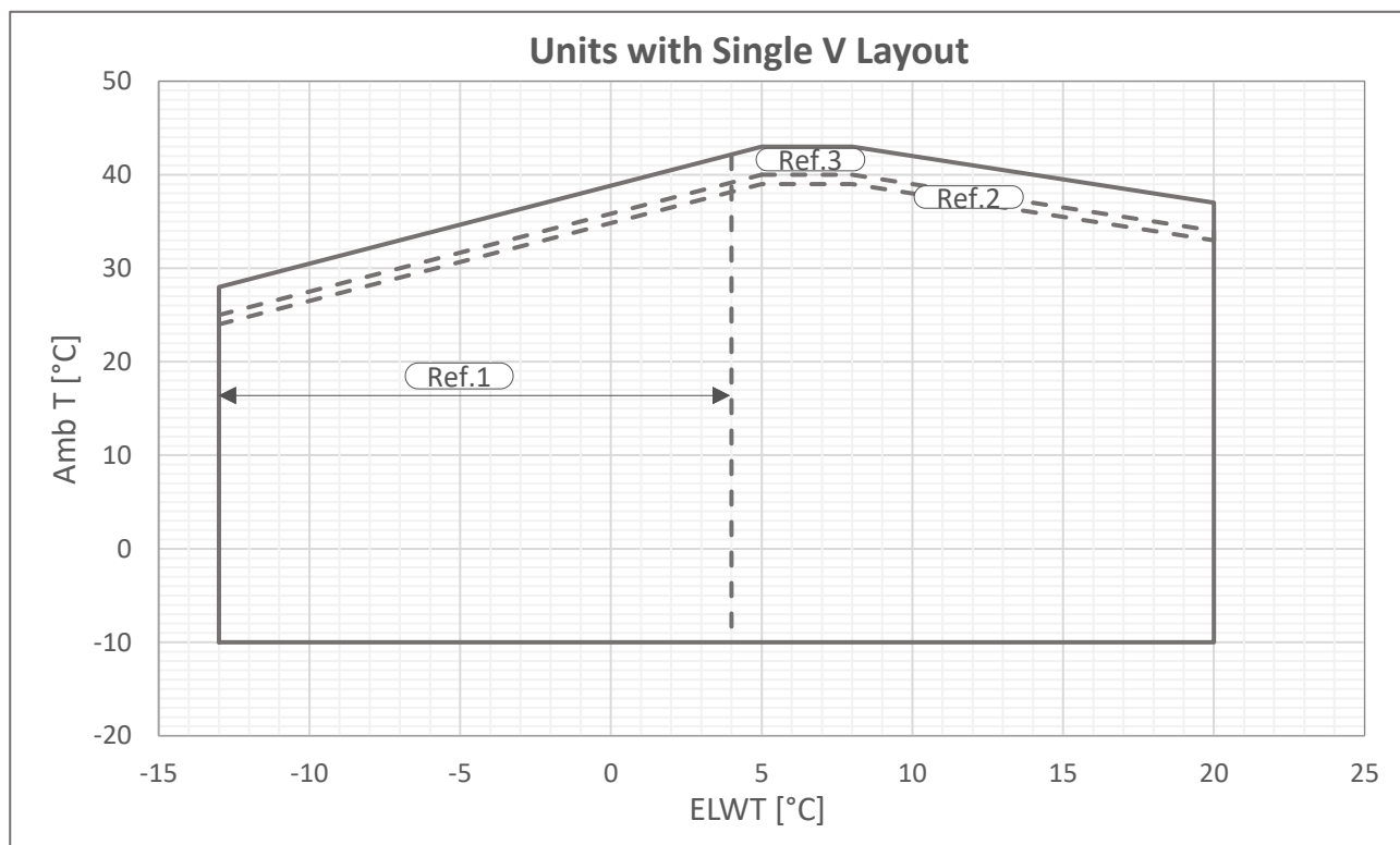
Fig. 3 - Limite de operare Single V-Silver
