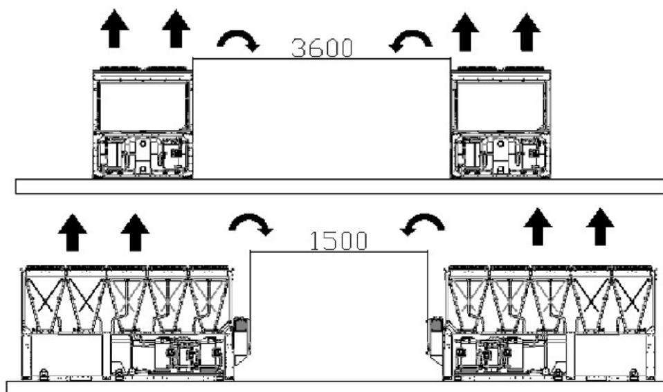
Fig. 7 - Cerințe minime de spațiu
