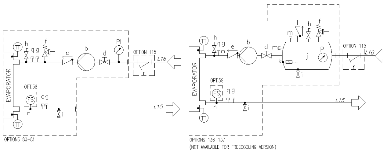
Fig. 11 – Diagrama hidraulică pentru pompa dublă single V ( EWATxx5B) (opț. 80-81/136-137) (presiune max. de operare 6 bari)
