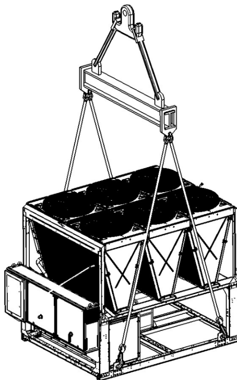
Jednotka so 4 zdvíhacími bodmi
