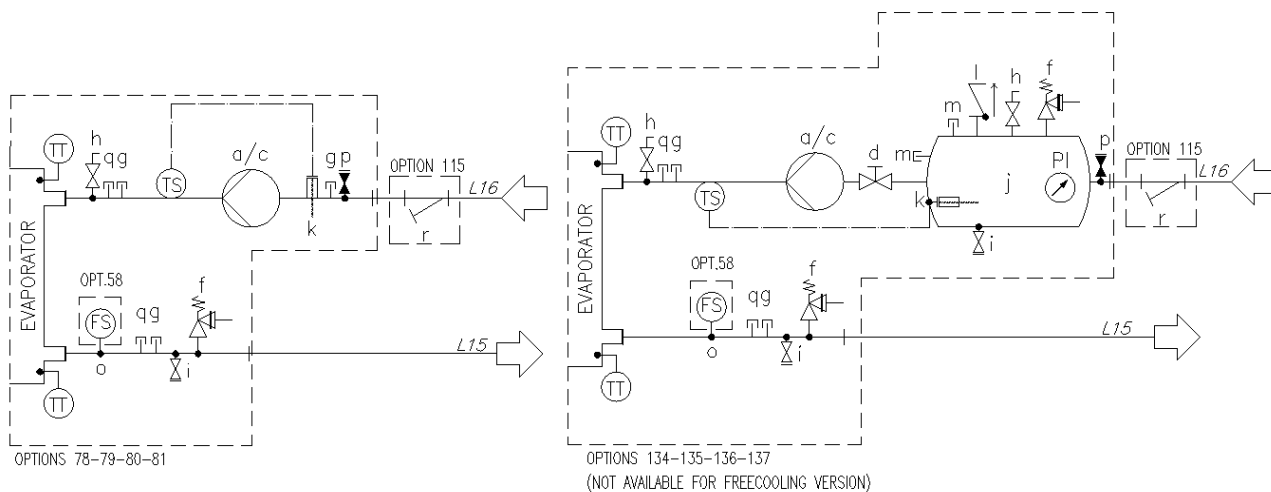
Obr. 12 – Hydraulická schéma pre Modular V (EWATxx0B) (vol. 78-79-80-81/134-135-136-137) (max. prevádzkový tlak 6 barov)
