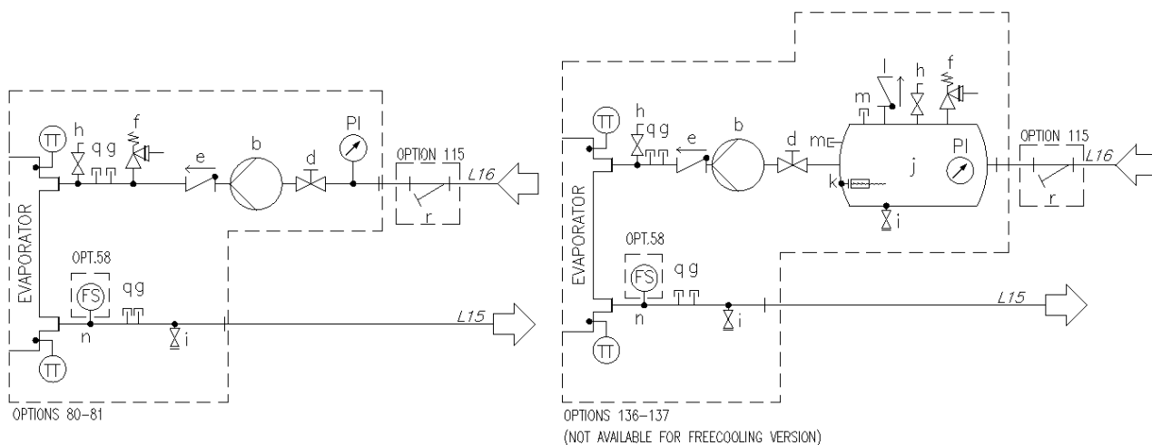
Obr. 11 – Hydraulická schéma pre dvojité čerpadlo Single V (EWATxx5B) (vol. 80-81/136-137) (max. prevádzkový tlak 6 barov)
