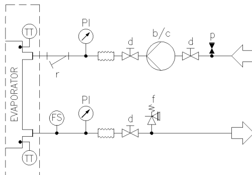
Obr. 9 – Hydraulická schéma bez čerpadla(-iel) (maximálny prevádzkový tlak 20 bar)
