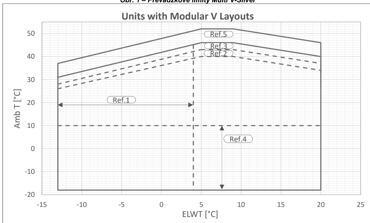
Obr. 2 – Prevádzkové limity Multi V-Gold
