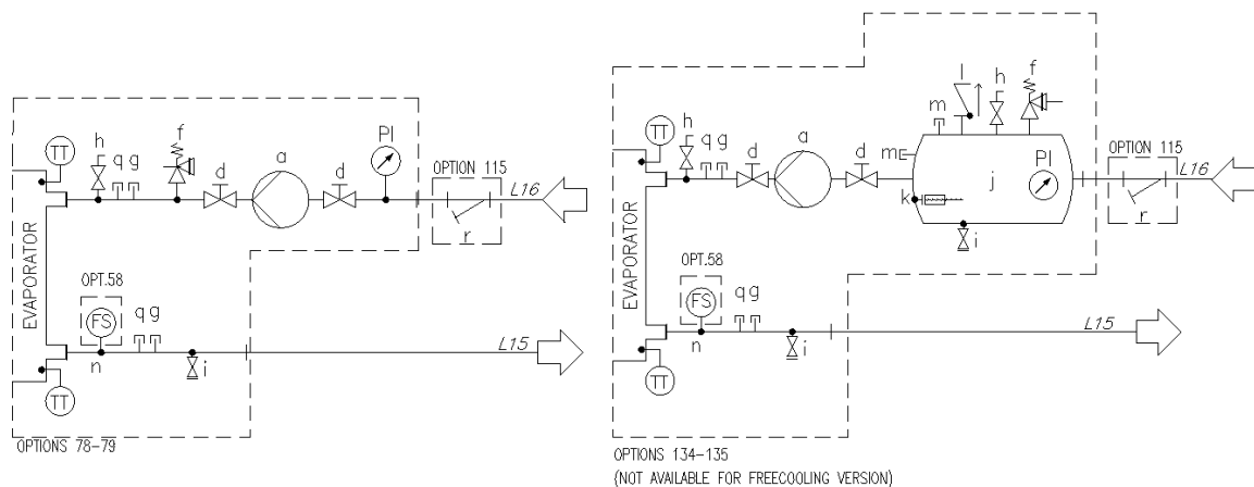
Obr. 10 – Hydraulická schéma pre samostatné čerpadlo Single V (EWATxx5B) (vol. 78-79/134-135) (max. prevádzkový tlak 6 barov)
