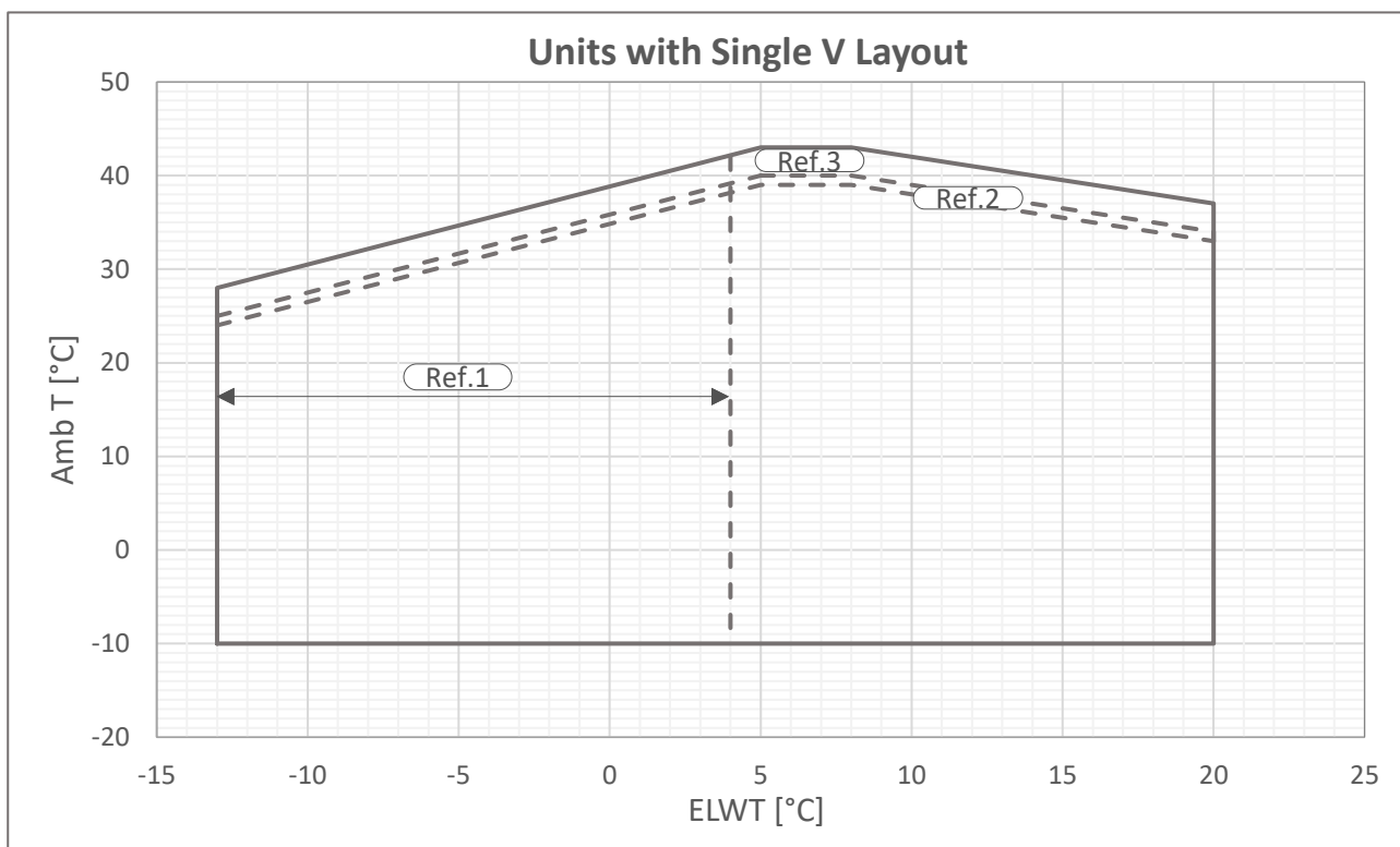
Obr. 3 – Prevádzkové limity Single V-Silver
