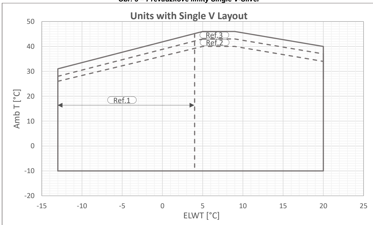
Obr. 4 – Prevádzkové limity Single V-Gold
