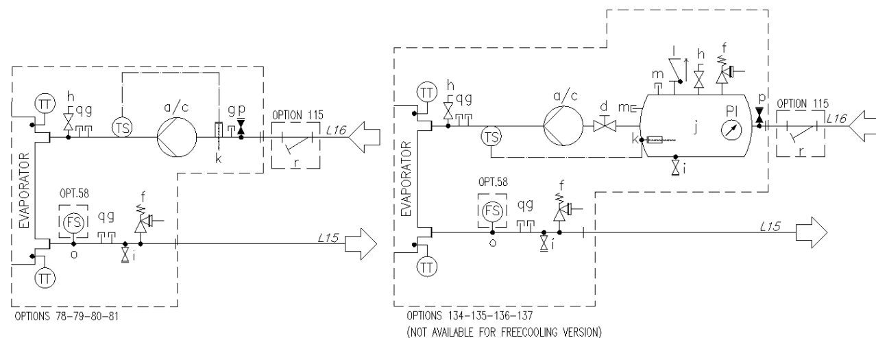
Slika 12 – hidravlična shema za modularno V (EWATxx0B) (št. 78-79-80-81/134-135-136-137) (max. operating pressure 6 bar)
