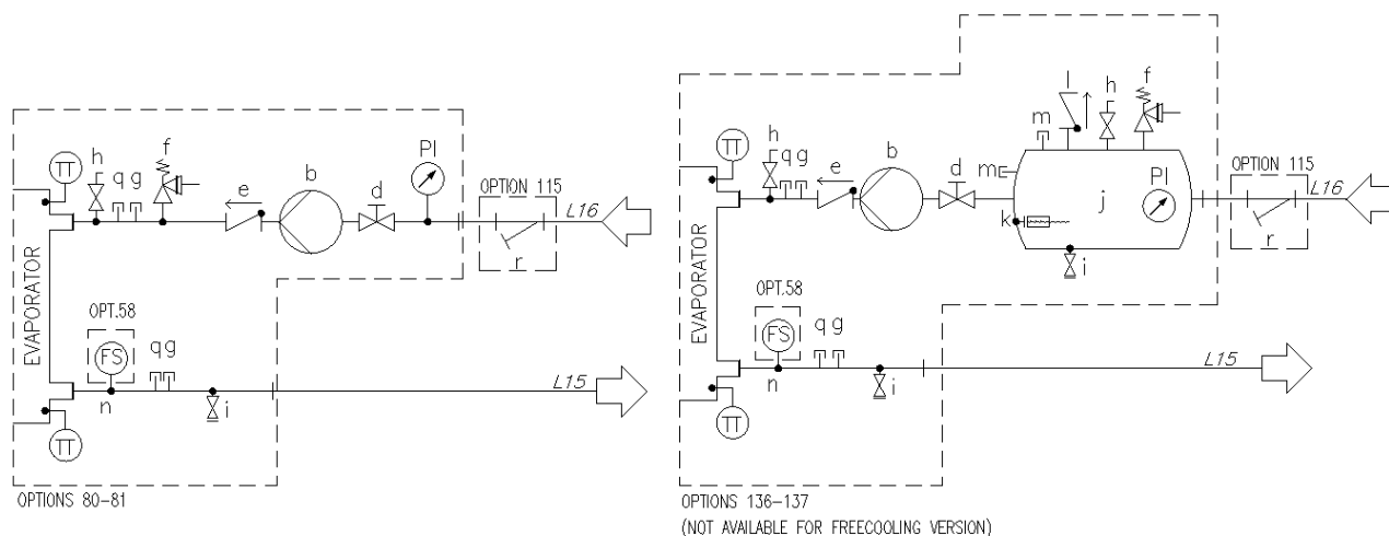
Slika 11 – hidravlična shema za eno V (EWATxx5B) z dvojno črpalko (št. 80-81/136-137) (max. operating pressure 6 bar)
