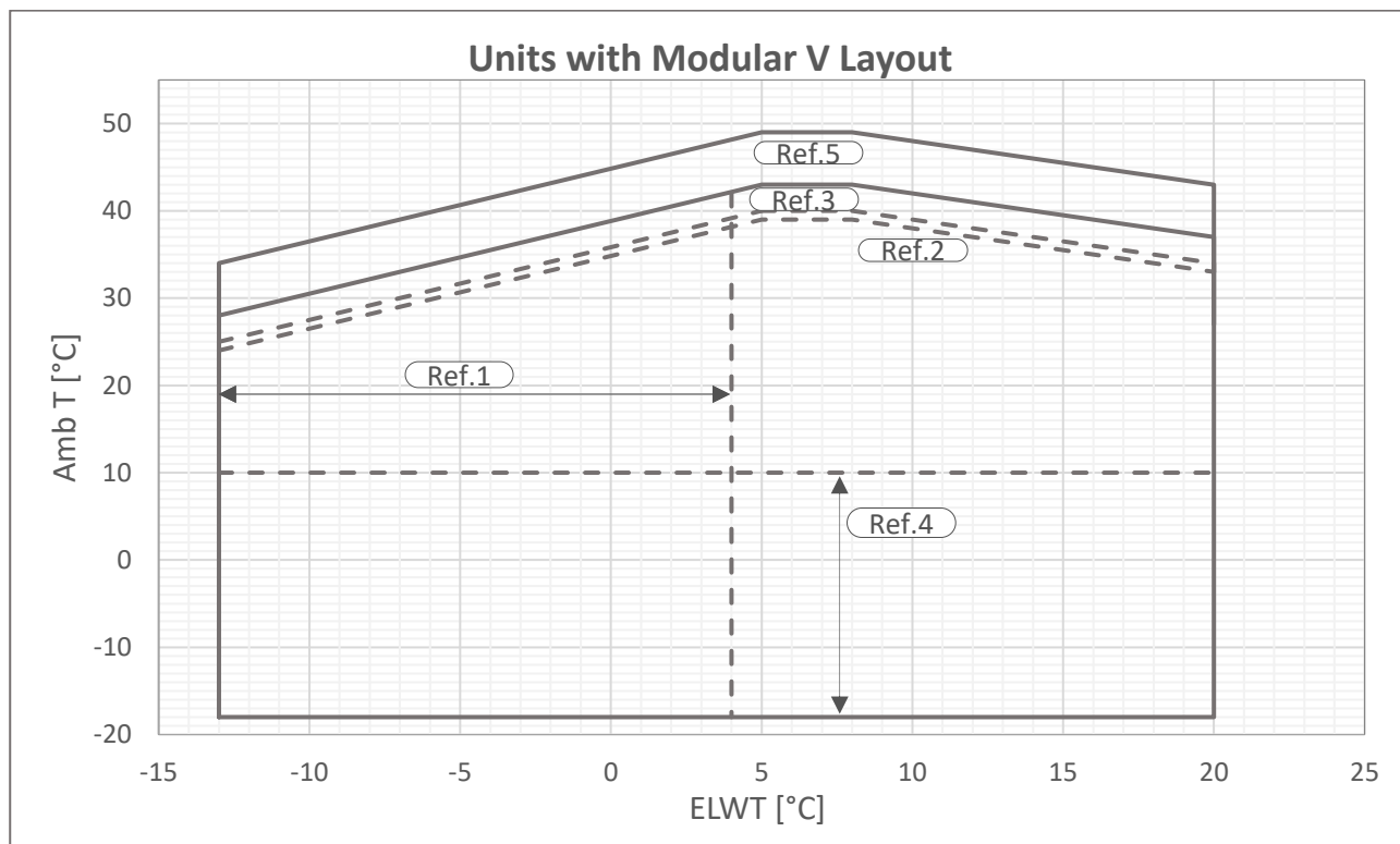
Slika 1 – Mejne delovne vrednosti za več enot V-Silver
