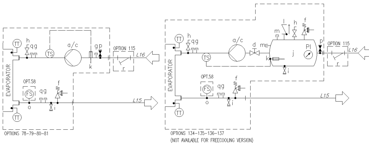
Fig. 12 – Hydrauliskt diagram för modulär V (EWATxx0B) (alt.78-79-80-81/134-135-136-137) (max arbetstryck 6 bar)
