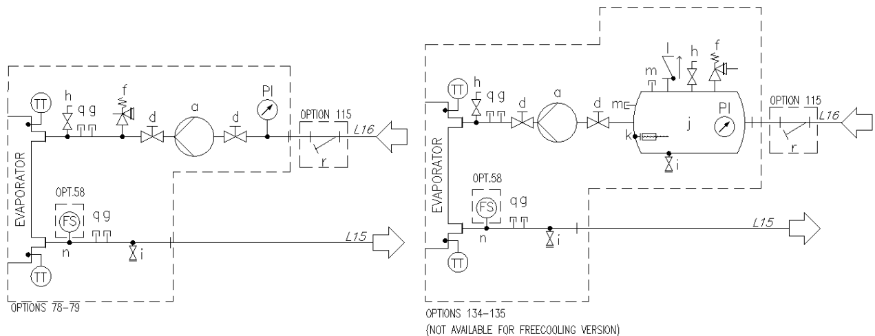
Fig. 10 – Hydrauliskt diagram för enkel V (EWATxx5B) enkel pump (alt.78-79/134-135) (max arbetstryck 6 bar)
