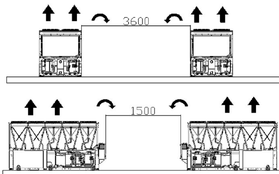
Fig. 7 - Krav på minsta utrymme
