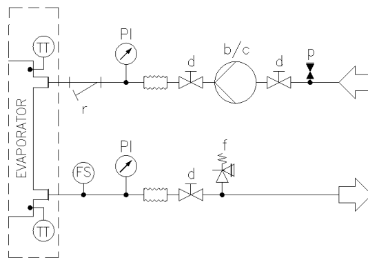
Fig. 9 – Hydrauliskt diagram utan pump(ar) ombord (max. arbetstryck 20 bar)
