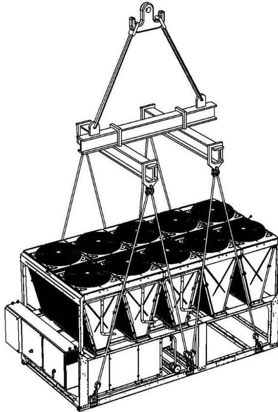
Enhet med sex lyftpunkter Ritningen visar bara modellen med 10 fläktar. Lyftläget är detsamma oavsett antal fläktar.
