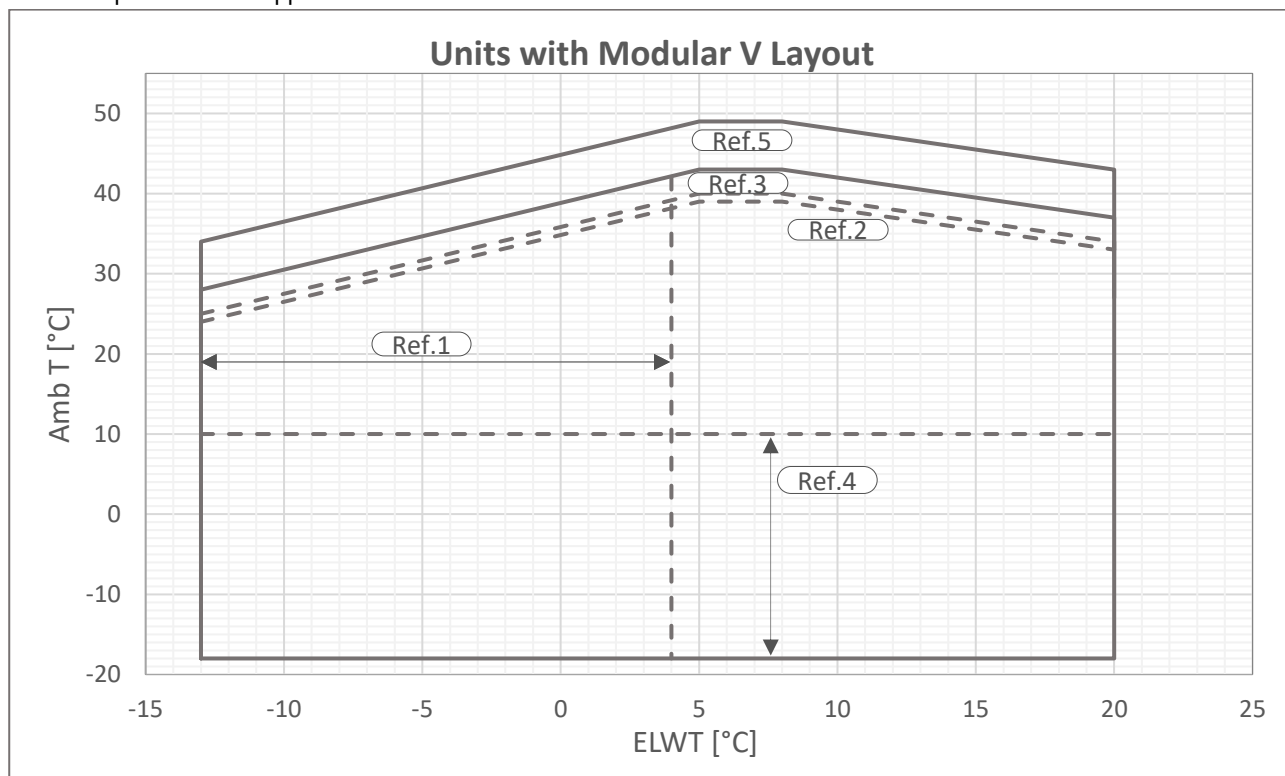
Fig. 1 - Multi V-Silver Driftgränser
