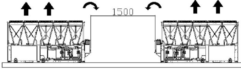
Şekil 7 - Minimum alan gereksinimleri
