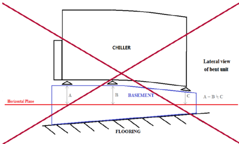
Şekil 6 - Birimin tesviyesi
