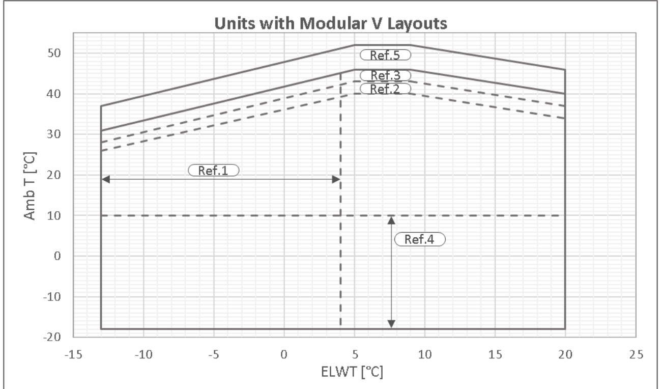
Şekil 2 - Çoklu V-Altın Çalışma sınırları
