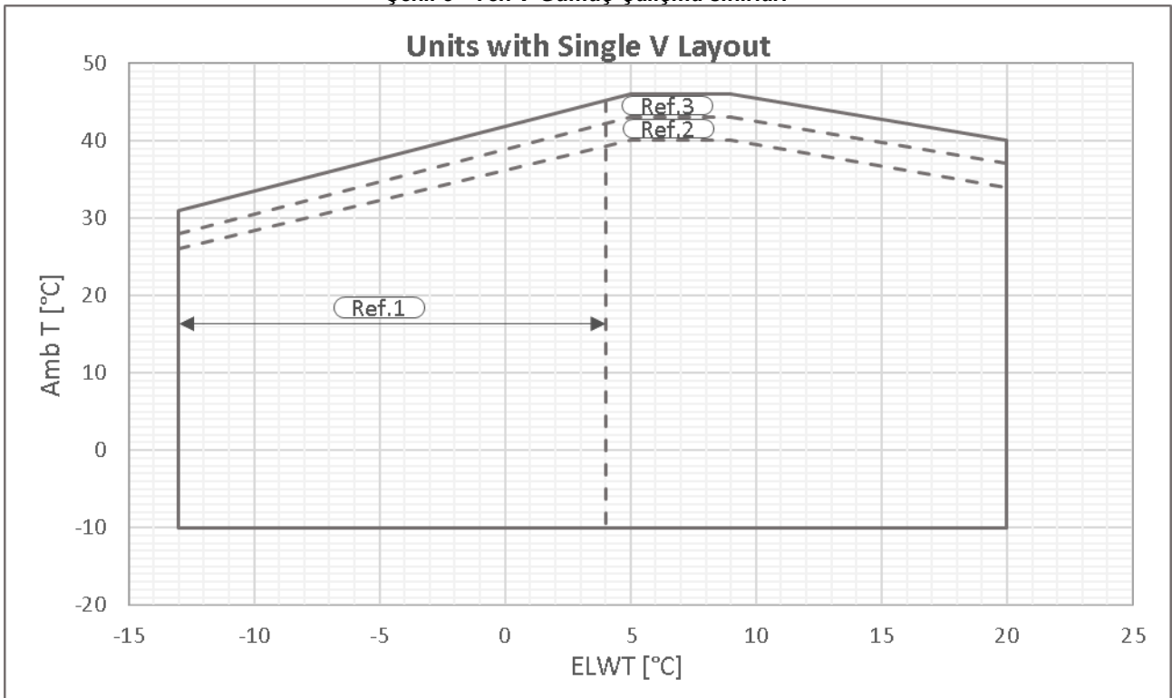
Şekil 4 - Tek V-Altın Çalışma sınırları
