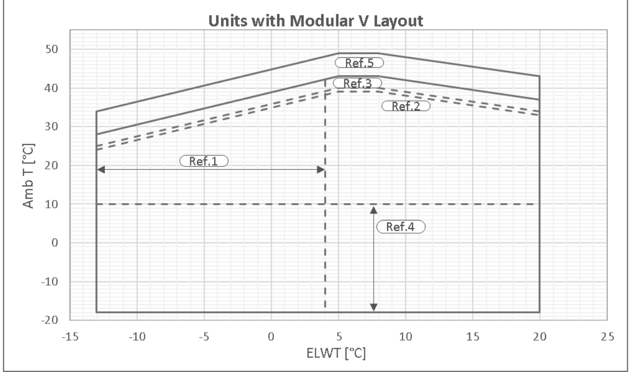
Şekil 1 - Çoklu V-Gümüş Çalışma sınırları
