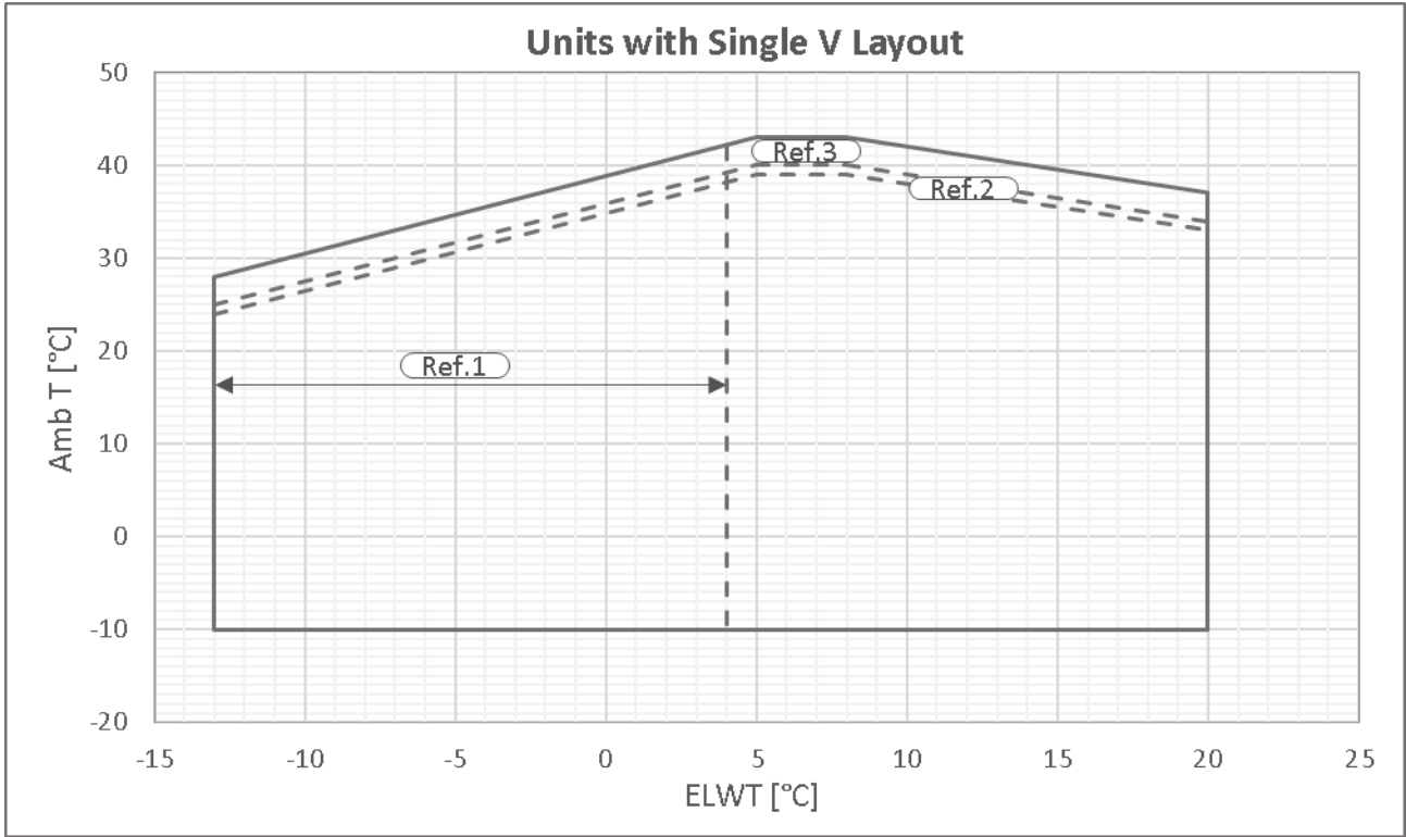
Şekil 3 - Tek V-Gümüş Çalışma sınırları
