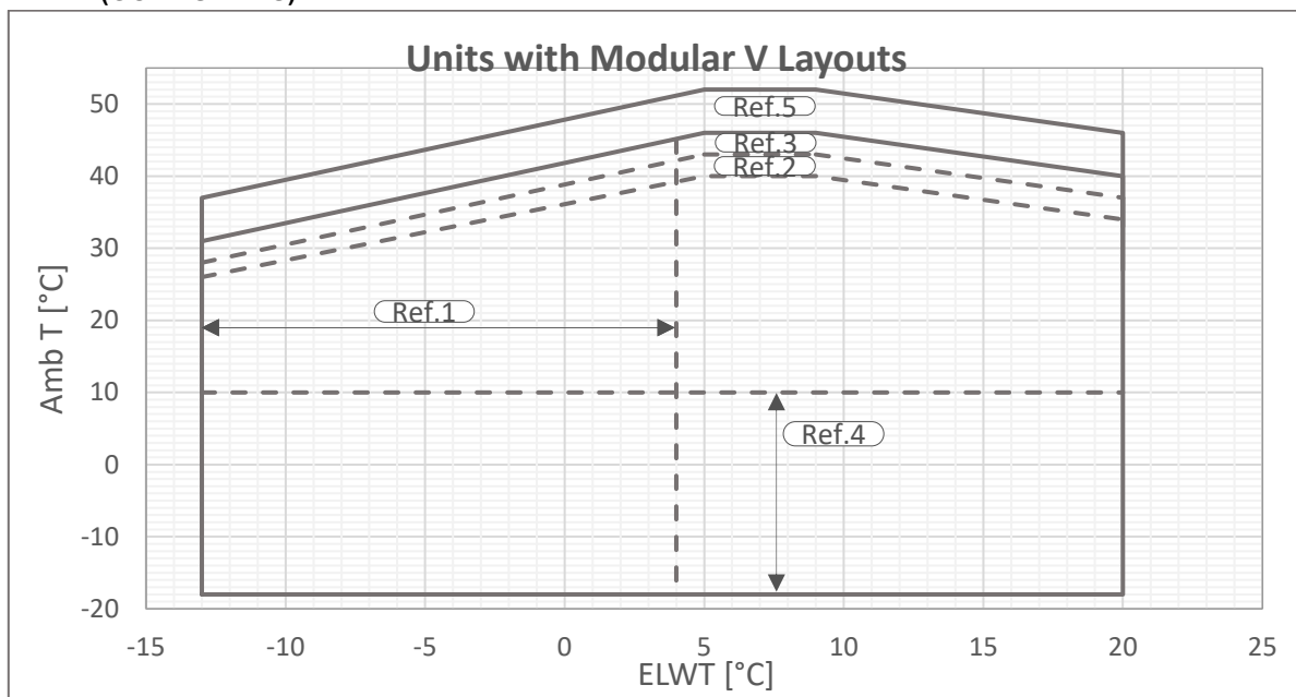
Obrázek 3 - Provozní limity Multi V-Gold
