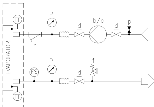
Obrázek 9- Návrh hydrauliky bez čerpadla (čerpadel) (max. provozní tlak 20 bar)
