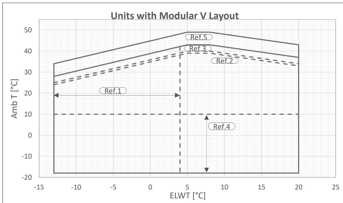
Obrázek 2 - Provozní limity Multi V-Silver
