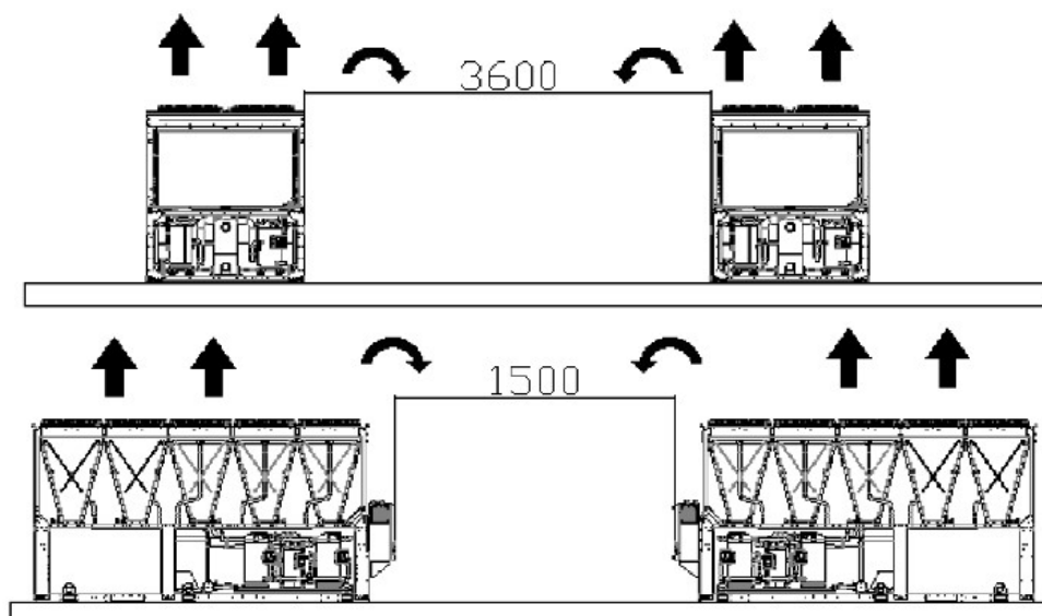
Obrázek 7- Požadavky minimálního prostoru
