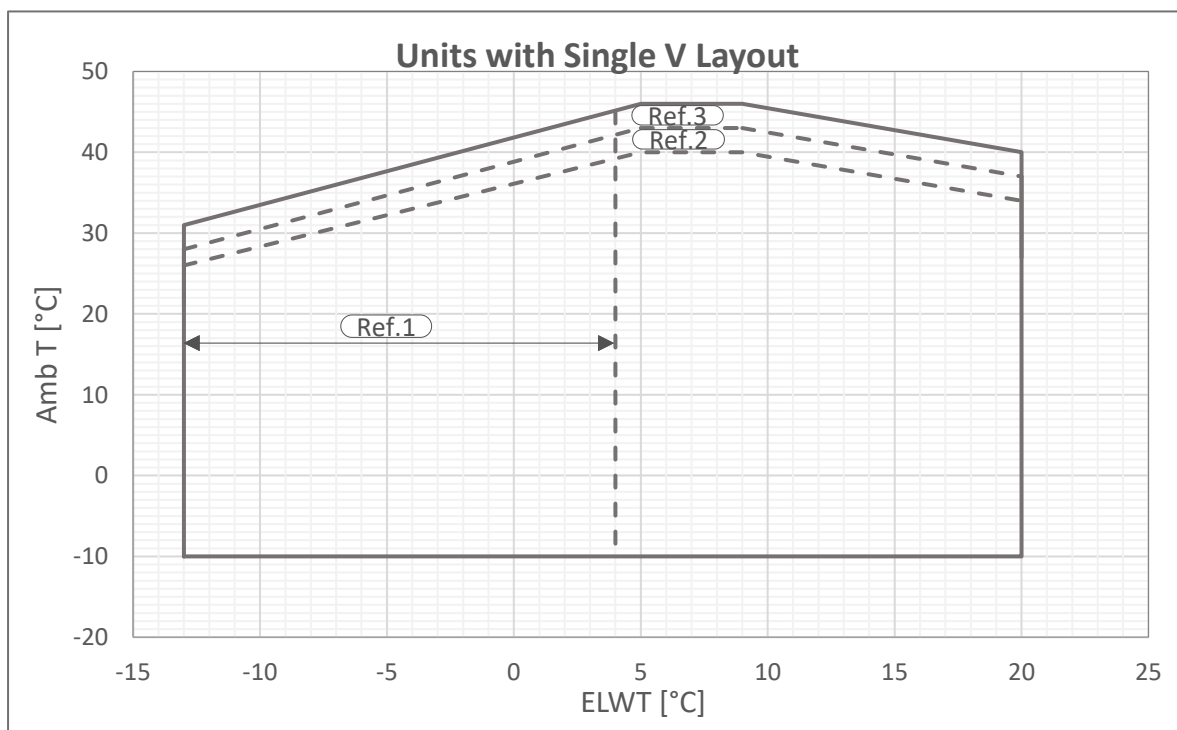
Obrázek 4 - Provozní limity Single V-Gold
