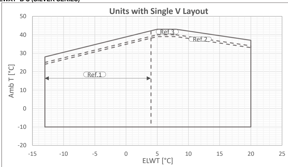
Obrázek 1- Provozní limity Single V-Silver
