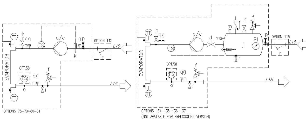
Obrázek 12- Hydraulické schéma pro modulární V (EWATxx0B) (vol. 78-79-80-81/134-135-136-137) (max. provozní tlak 6 bar)
