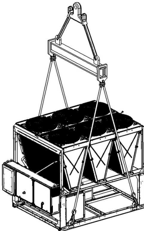
Jednotka se 4 zvedacími body
