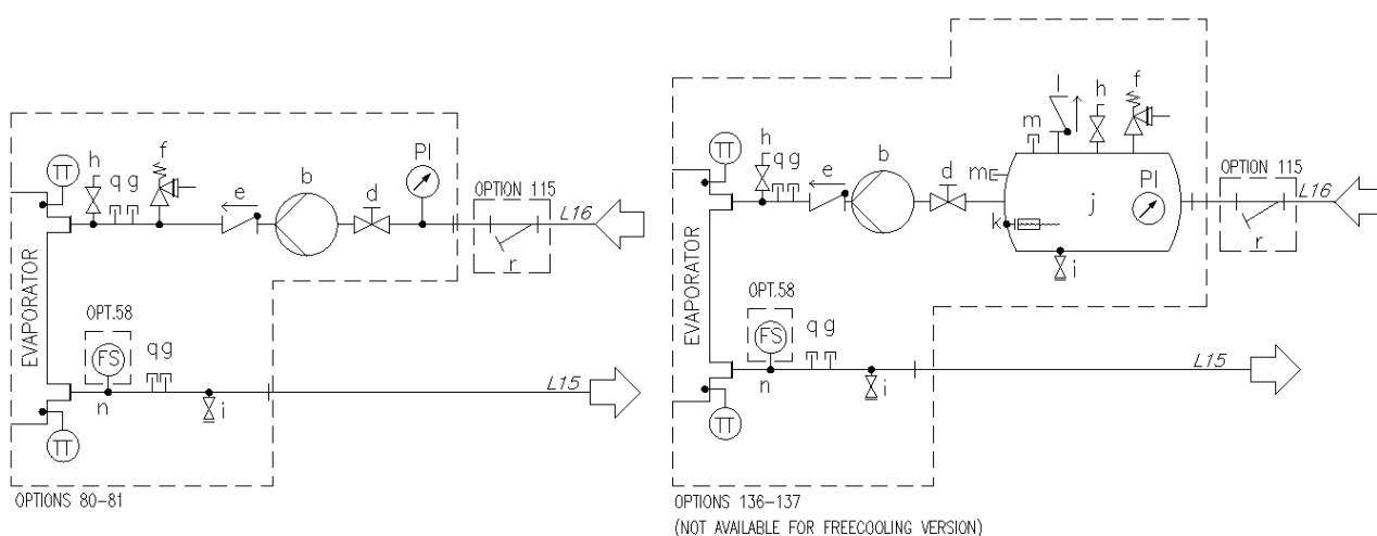
Obrázek 11 - Schéma hydraulické soustavy pro dvojité V (EWATxx5B) čerpadlo (vol. 80-81/136-137) (max. provozní tlak 6 bar)
