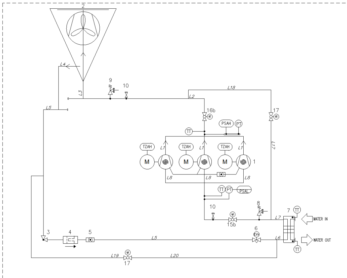
Obrázek 14- Náčrtes chladicího okruhu (P&ID) jednotka se slabým chlazením venkovním vzduchem jedním okruhem
