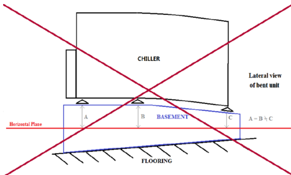
Obrázek 6- Vyvážení jednotky
