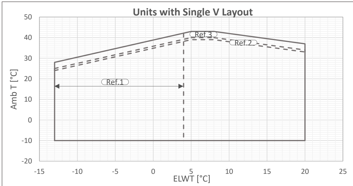
Abb. 1 - Einzelner V-Silber Betriebsgrenzen
