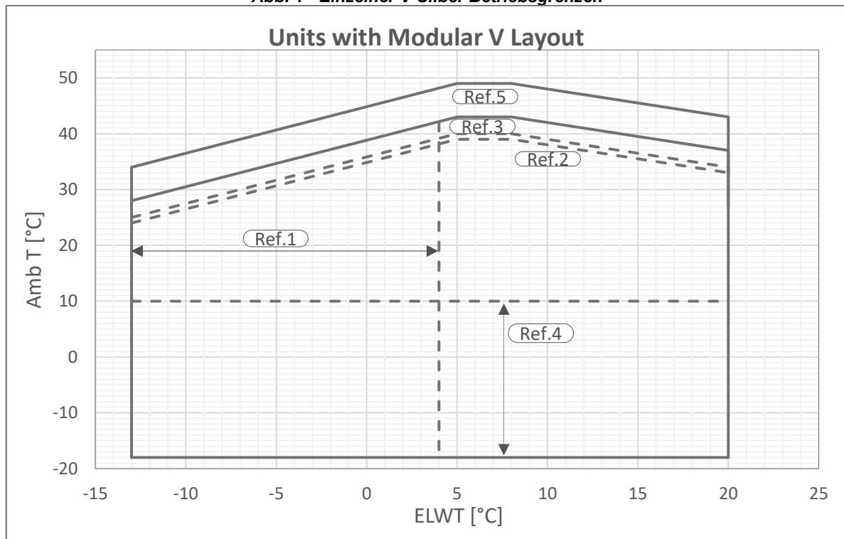
Abb. 10 - Multi-V-Silber Betriebsgrenzen
