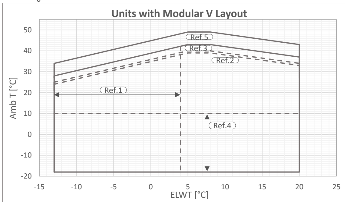
Fig. 1 - Límites operativos de Multi V-Plata
