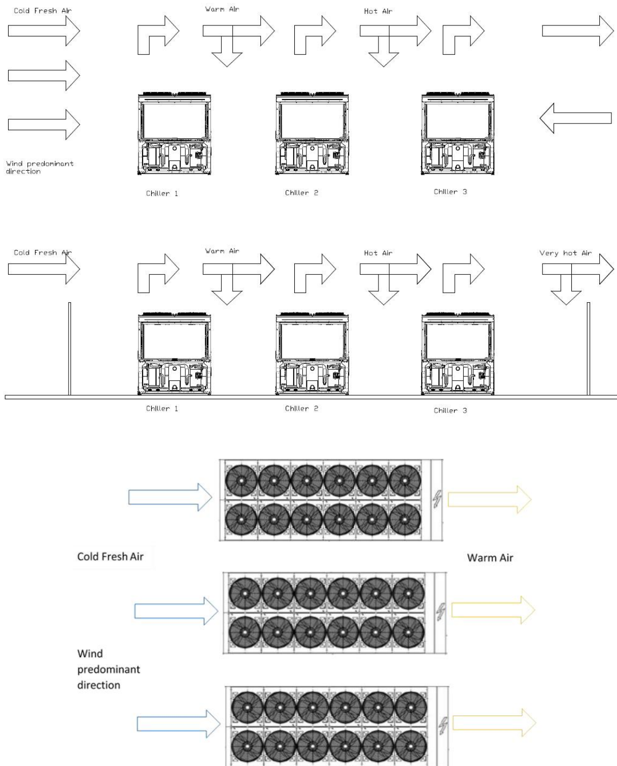
Fig. 8 – Instalación de Múltiples Refrigeradores
