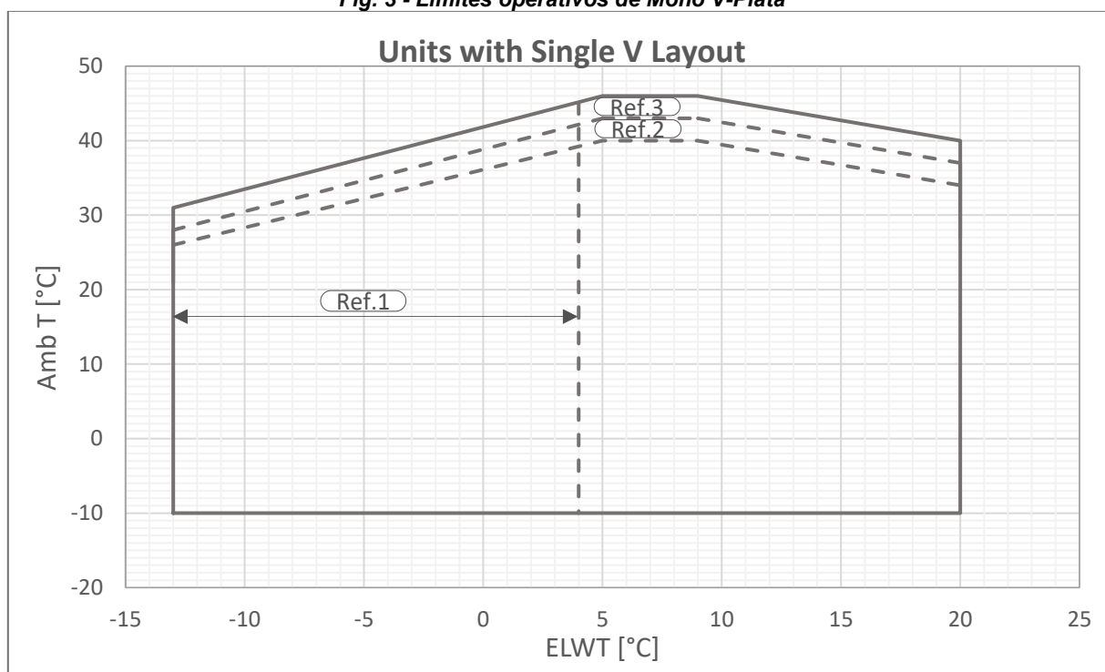
Fig. 4 - Límites operativos de Mono V-Oro
