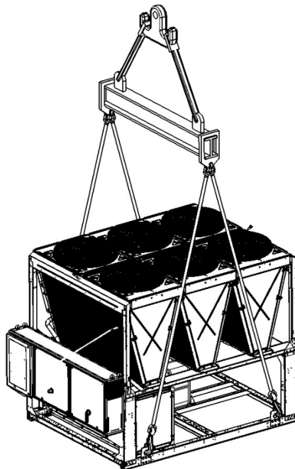
Unidad con 4 puntos de elevación
