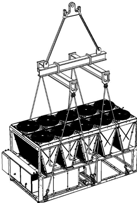
Unidad con 6 puntos de elevación
