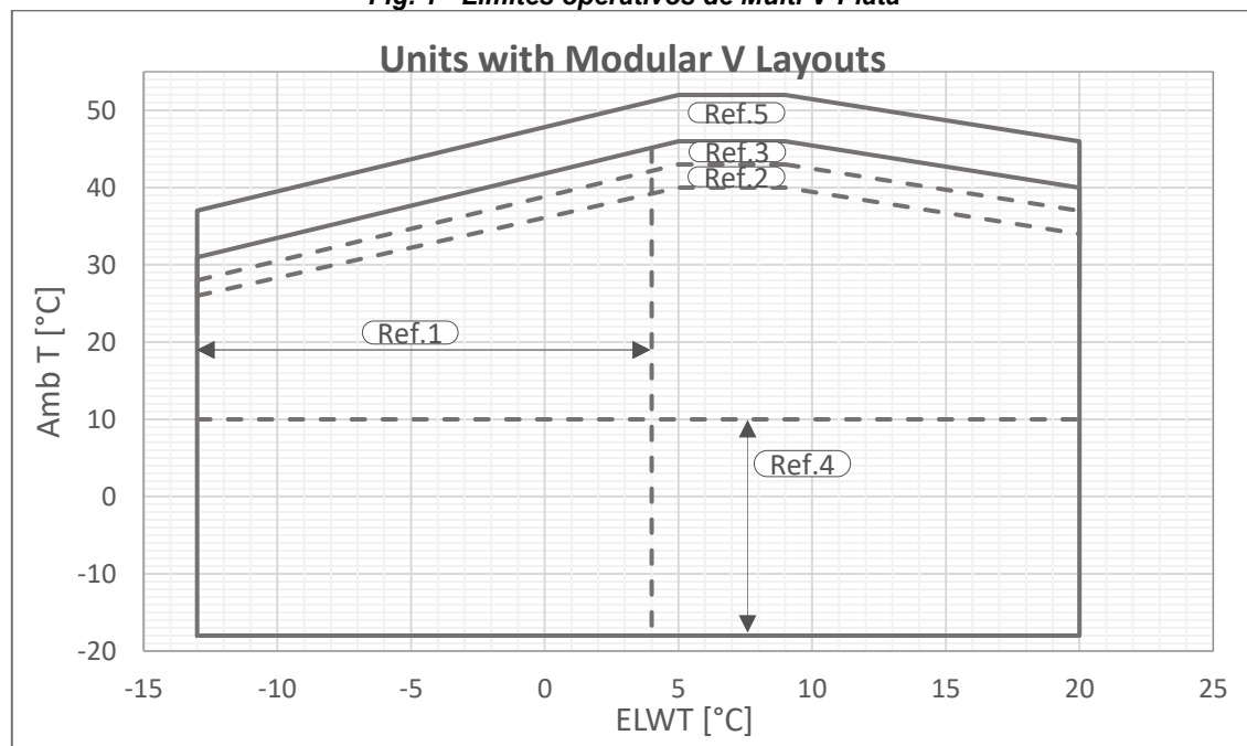
Fig. 2 - Límites operativos de Multi V-Oro
