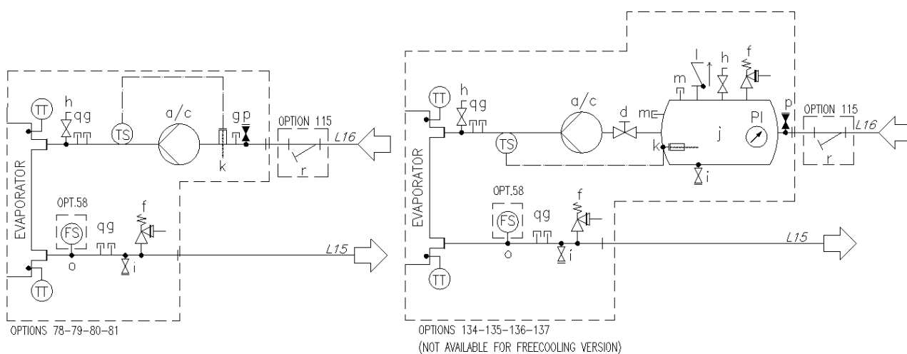
Fig. 11 – Diagrama hidráulico para mono V (EWATxx5B) bomba doble (opc. 80-81/136-137) (presión operativa máxima 6 bares)
