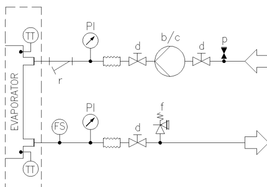
Fig. 9 – Diagrama hidráulico con bomba(s) a bordo (presión operativa máxima 20 bares)
