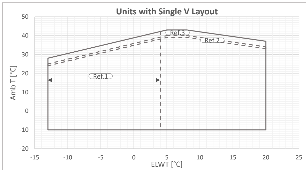
Fig. 3 - Límites operativos de Mono V-Plata
