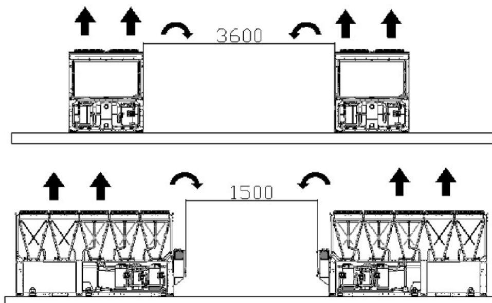
Fig. 7 - Encombrement minimal
