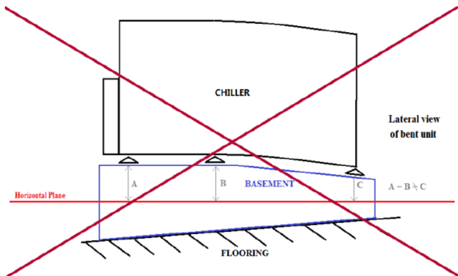
Fig. 6 - Nivellement de l'unité
