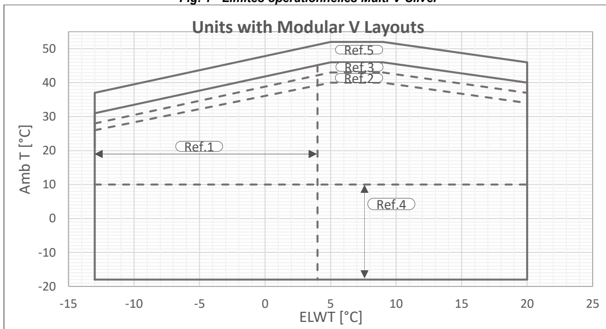
Fig. 2 - Limites opérationnelles Multi V-Gold
