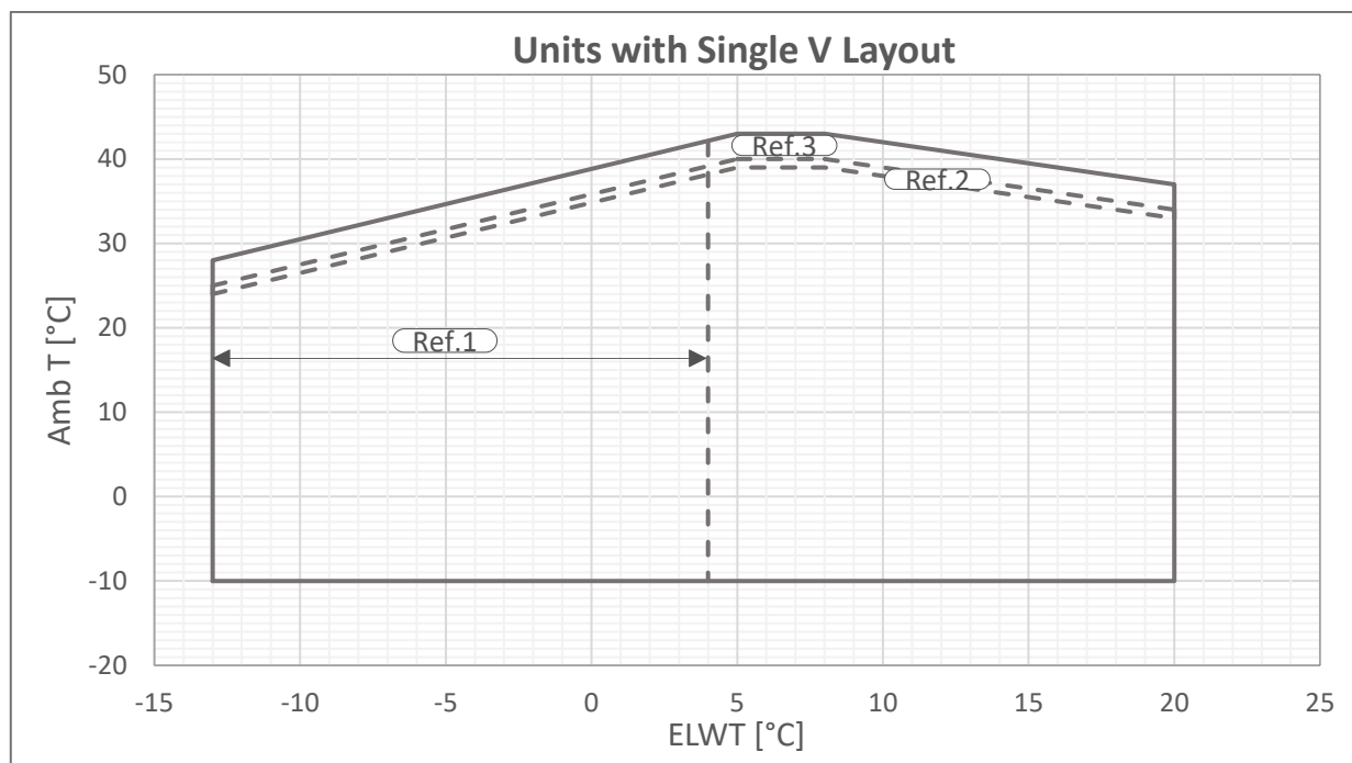
Fig. 3 - Limites opérationnelles Single V-Silver
