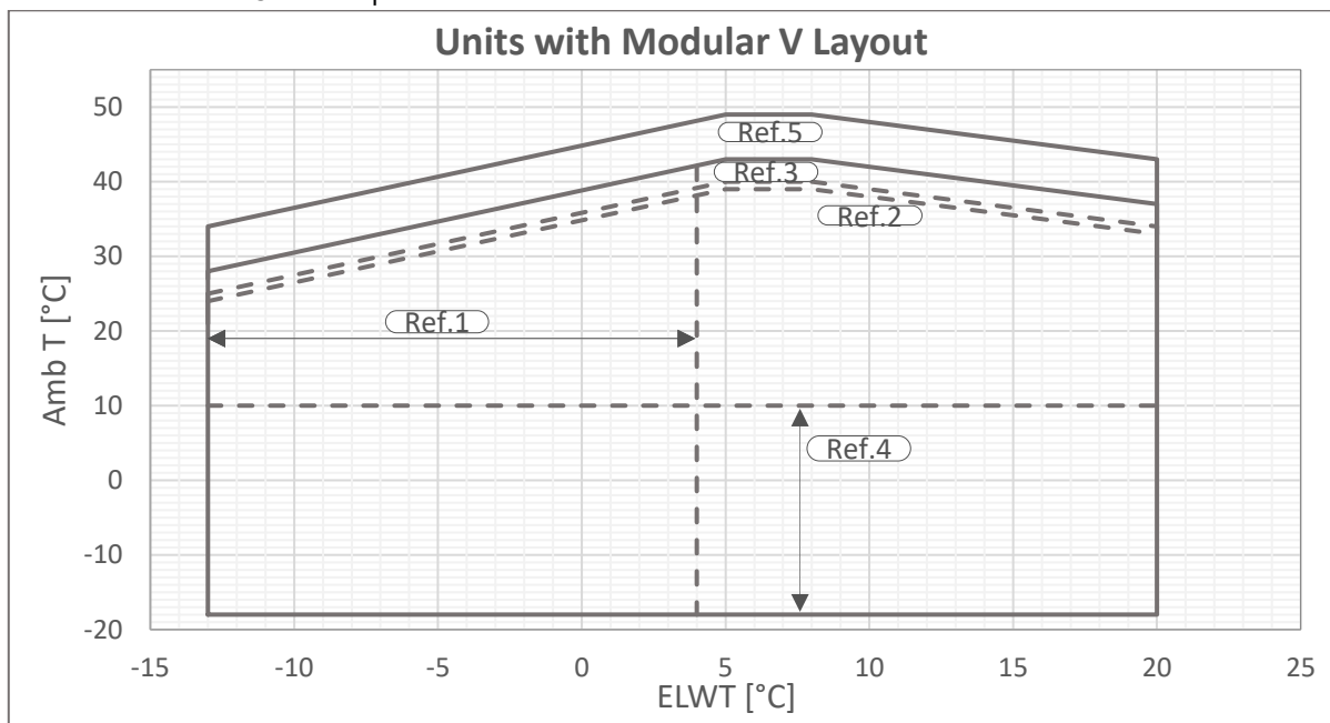
Fig. 1 - Limites opérationnelles Multi V-Silver
