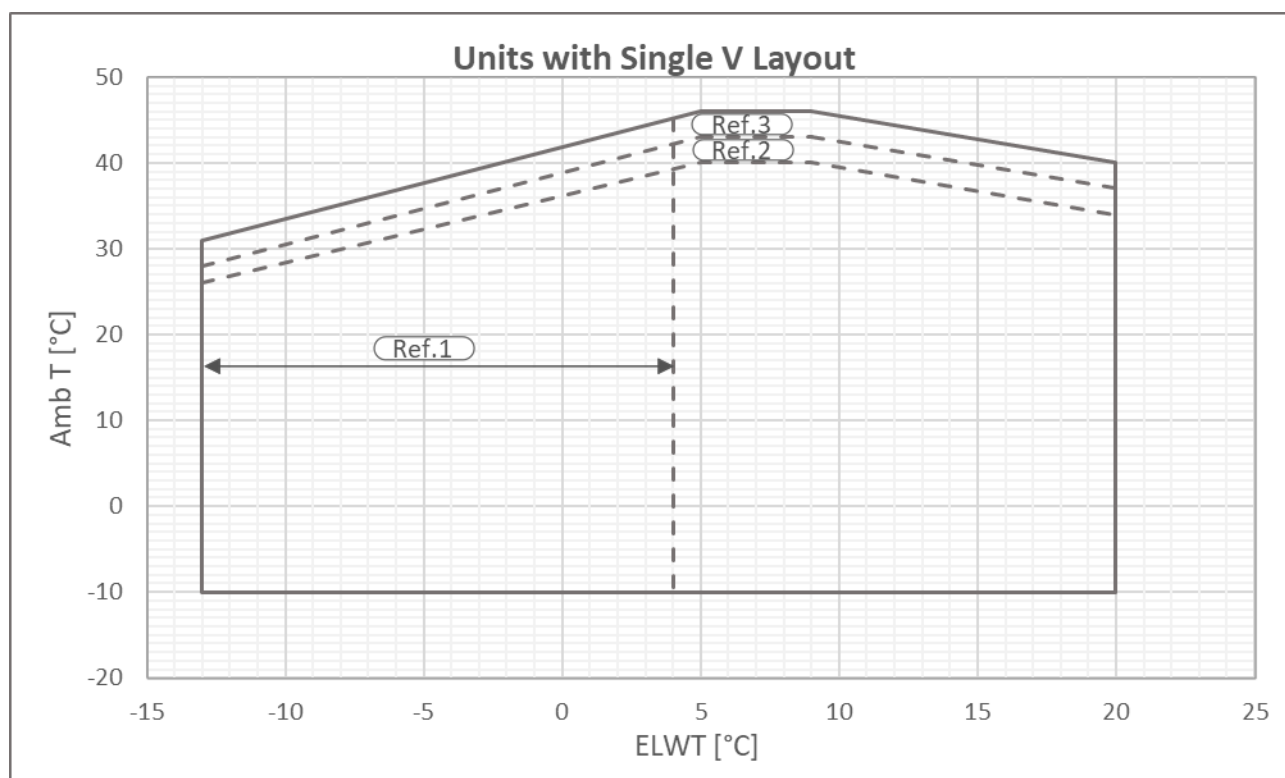
Slika 4 – Jednostruka V-zlatna radna ograničenja
