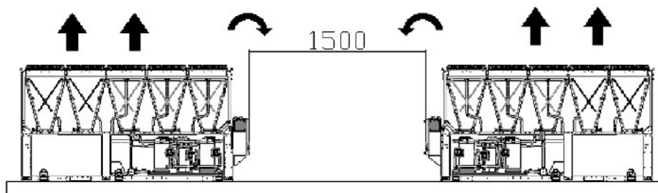
Slika 7 – Minimalni zahtjevi za prostor
