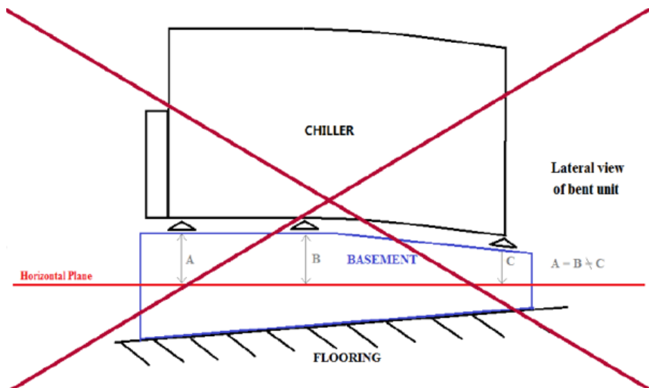
Slika 6 – Niveliranje jedinice
