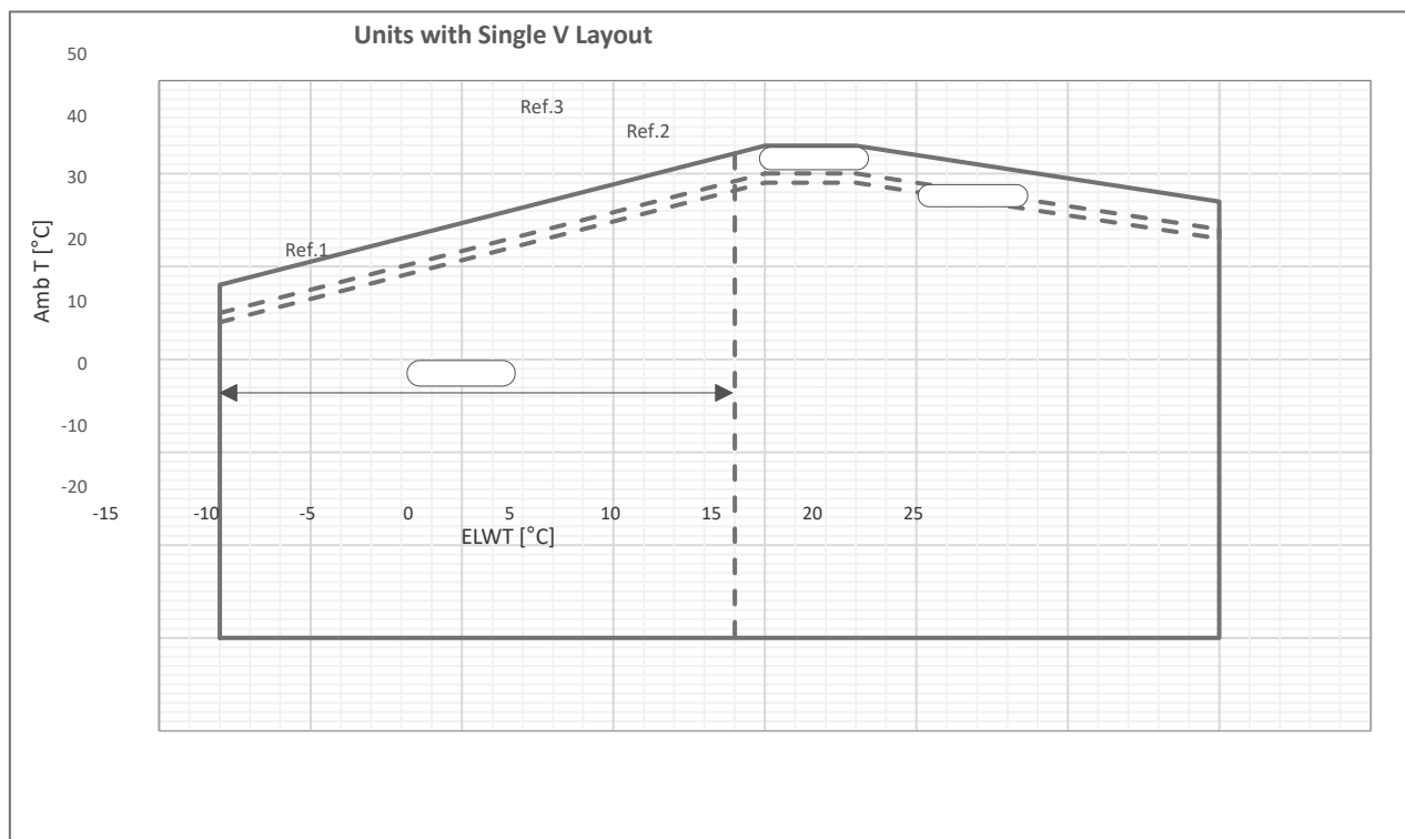
Slika 3 – Jednostruka V-srebrna radna ograničenja
