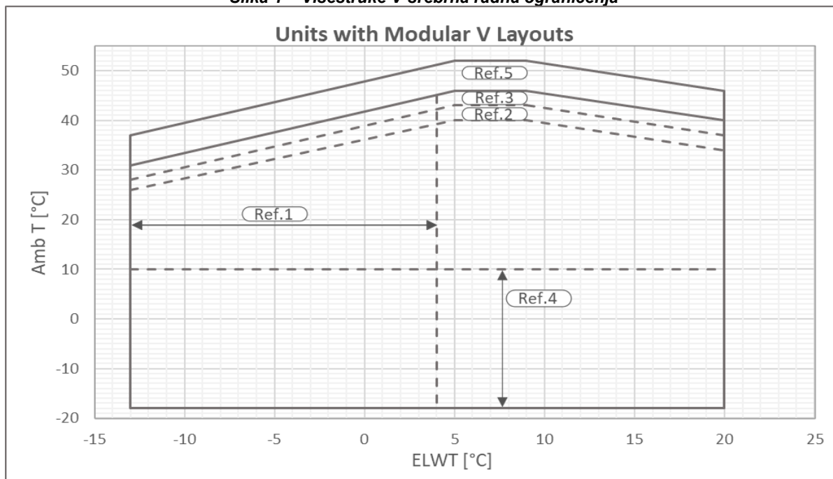
Slika 2 – Višestruka V-zlatna radna ograničenja
