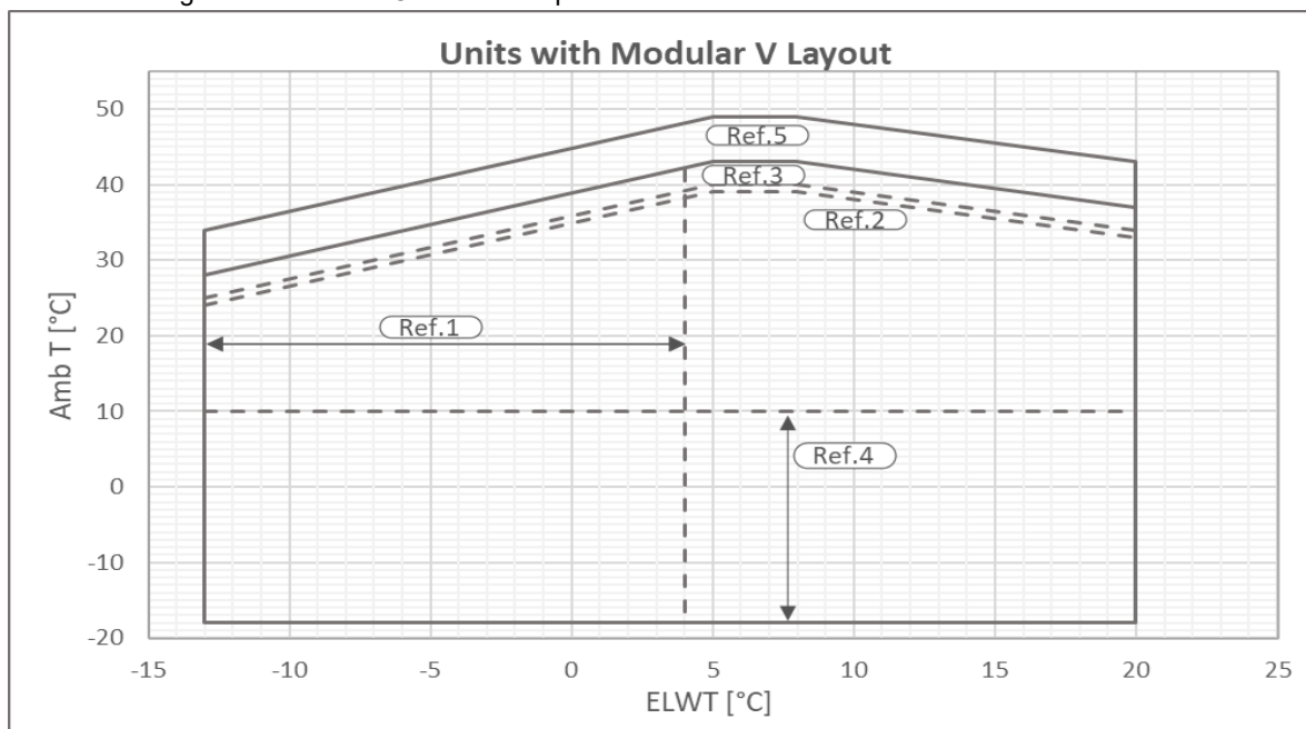
Slika 1 – Višestruke V-srebrna radna ograničenja
