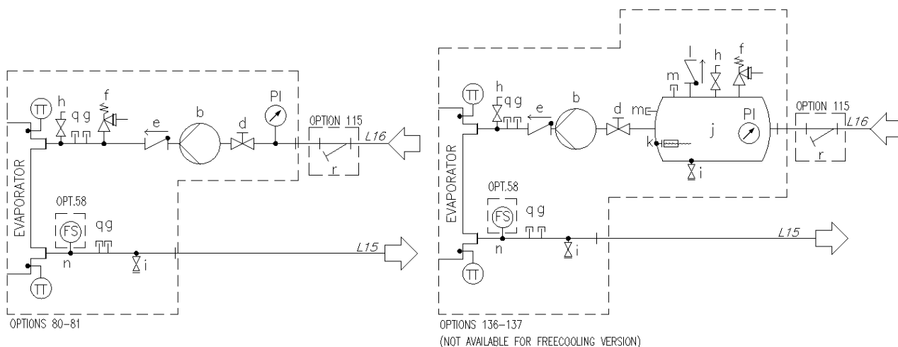
11. ábra – Hidraulikai ábra egy ventilátoros (EWATxx5B) dupla szivattyús géphez (opt. 80-81/136-137) (max. üzemi nyomás 6 bar)
