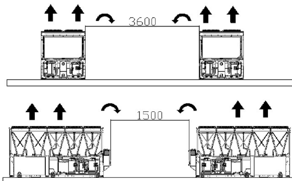
7. ábra - Minimális térszükséglet
