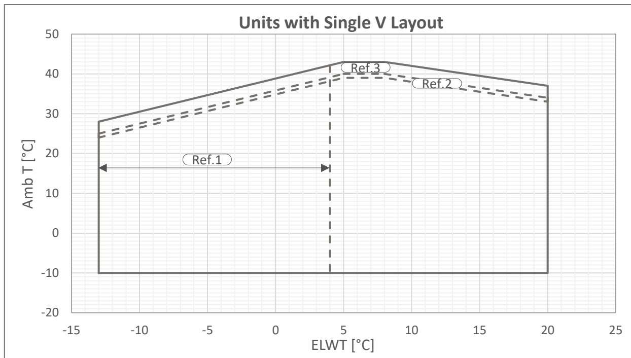
3. ábra - Egy ventilátoros V-Silver egység üzemi tartományai
