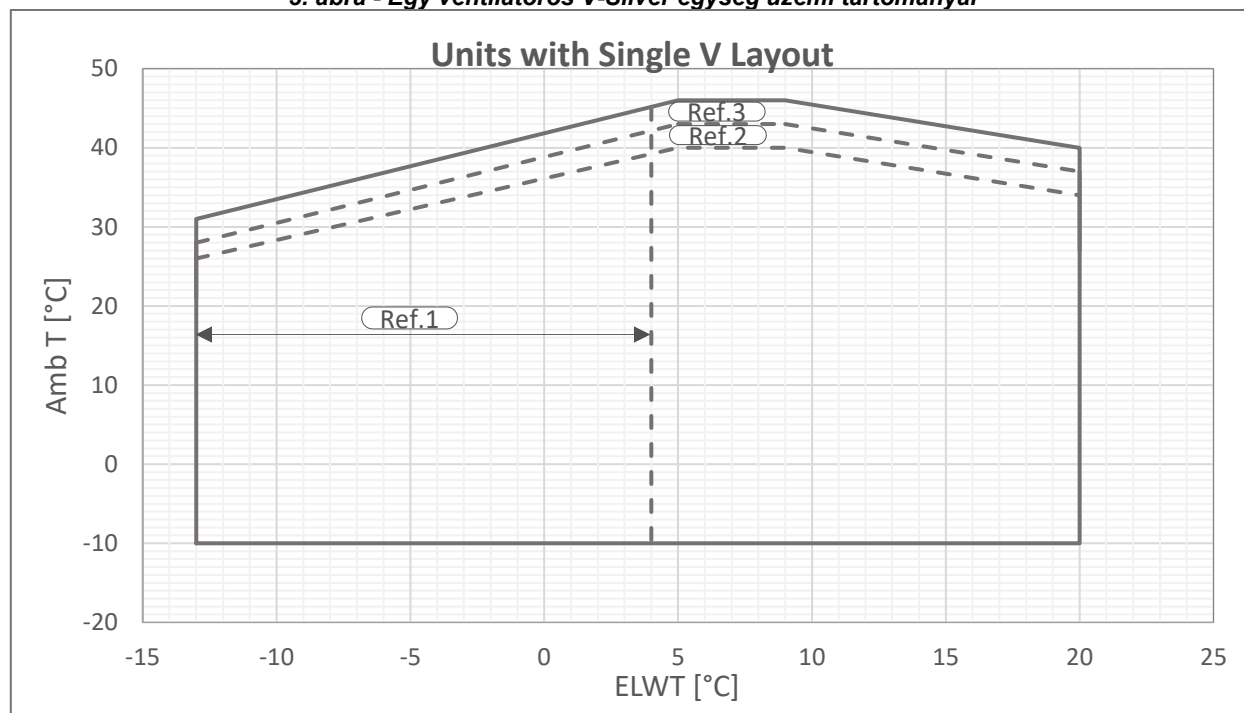
4. ábra - Egy ventilátoros V-Gold egység üzemi tartományai
