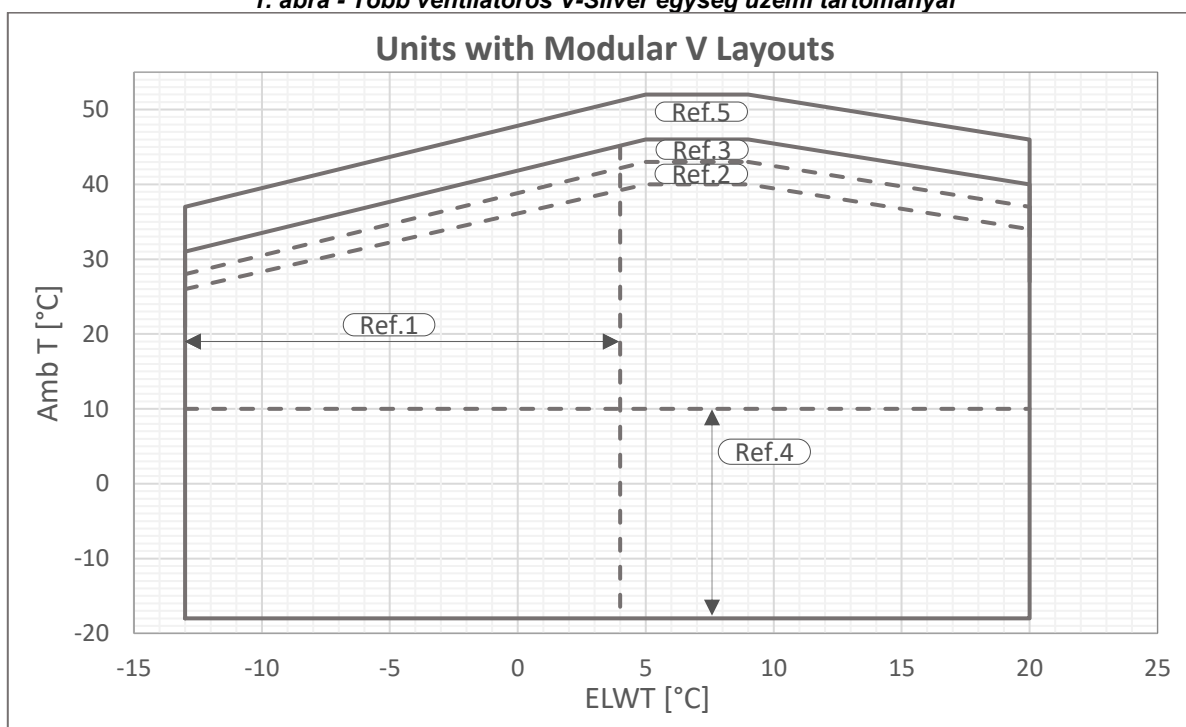
2. ábra - Több ventilátoros V-Gold egység üzemi tartományai
