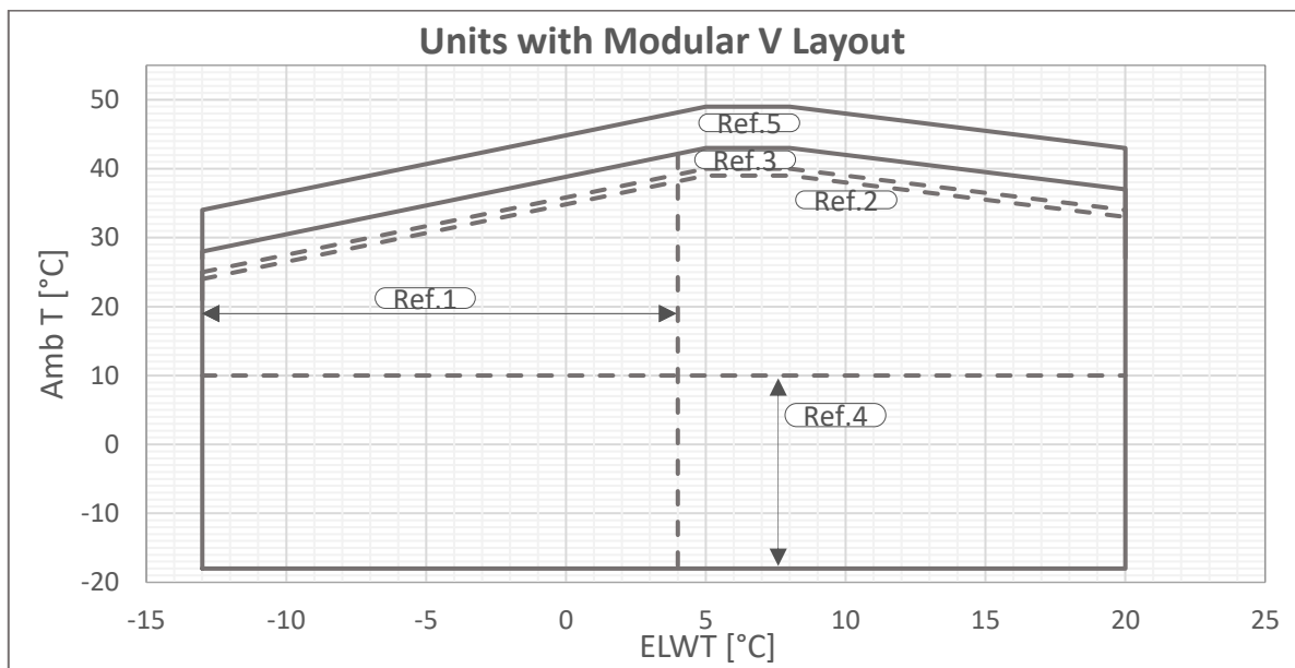
1. ábra - Több ventilátoros V-Silver egység üzemi tartományai
