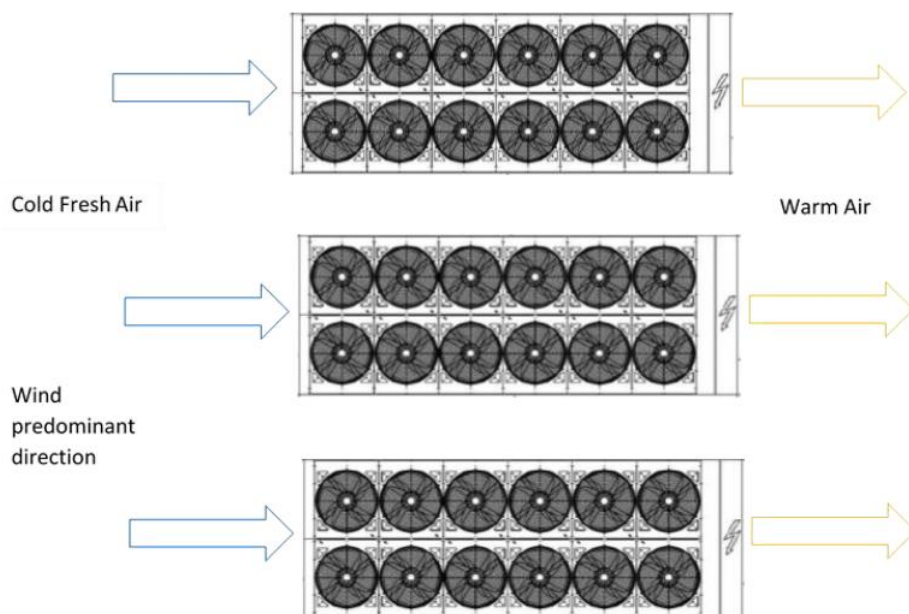
Fig. 8 - Installazione di chiller multipli
