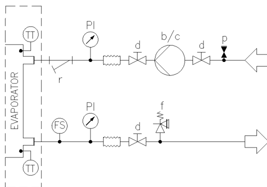
Fig. 9 – Schema idraulico senza pompa/e a bordo (pressione massima operativa 20 bar)
