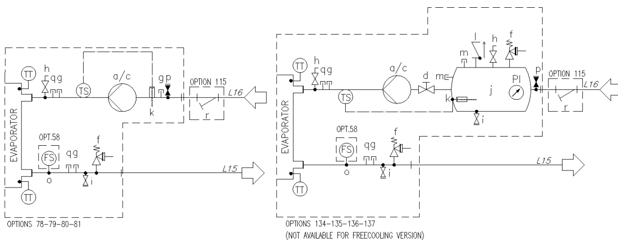
Fig. 12 - Schema idraulico per Modular V (EWATxx0B) (opz. 78-79-80-81/134-135-136-137) (pressione massima operativa 6 bar)
