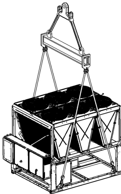
Unità con 4 punti di sollevamento
