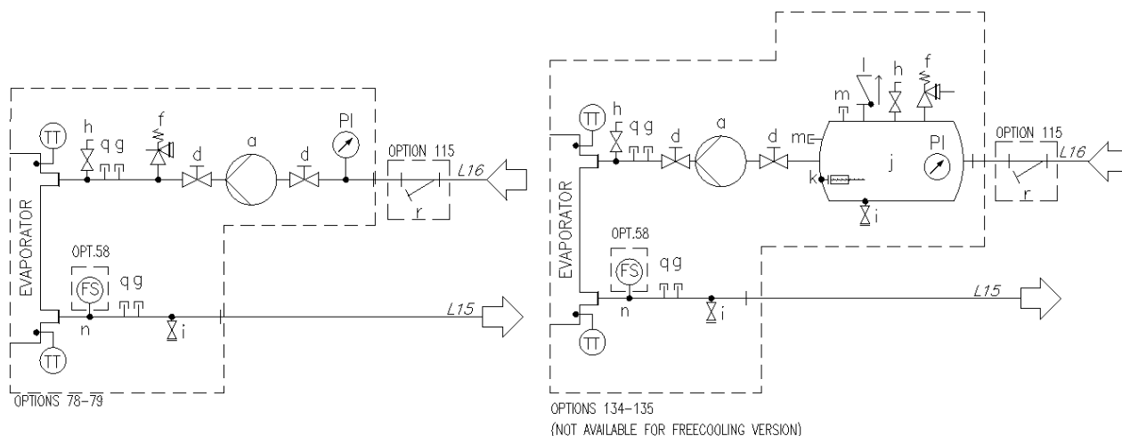
Fig. 10 – Schema idraulico per pompa singola single V (EWATxx5B) (opz. 78-79/134-135) (pressione massima operativa 6 bar)
