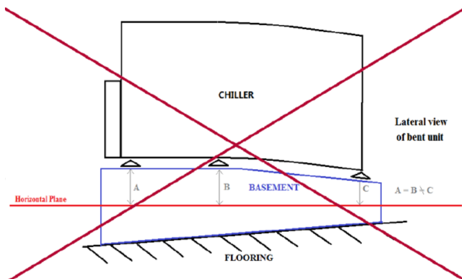
Fig. 6 - Livellamento unità
