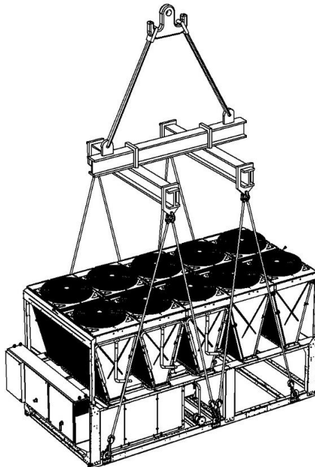
Unità con 6 punti di sollevamento
