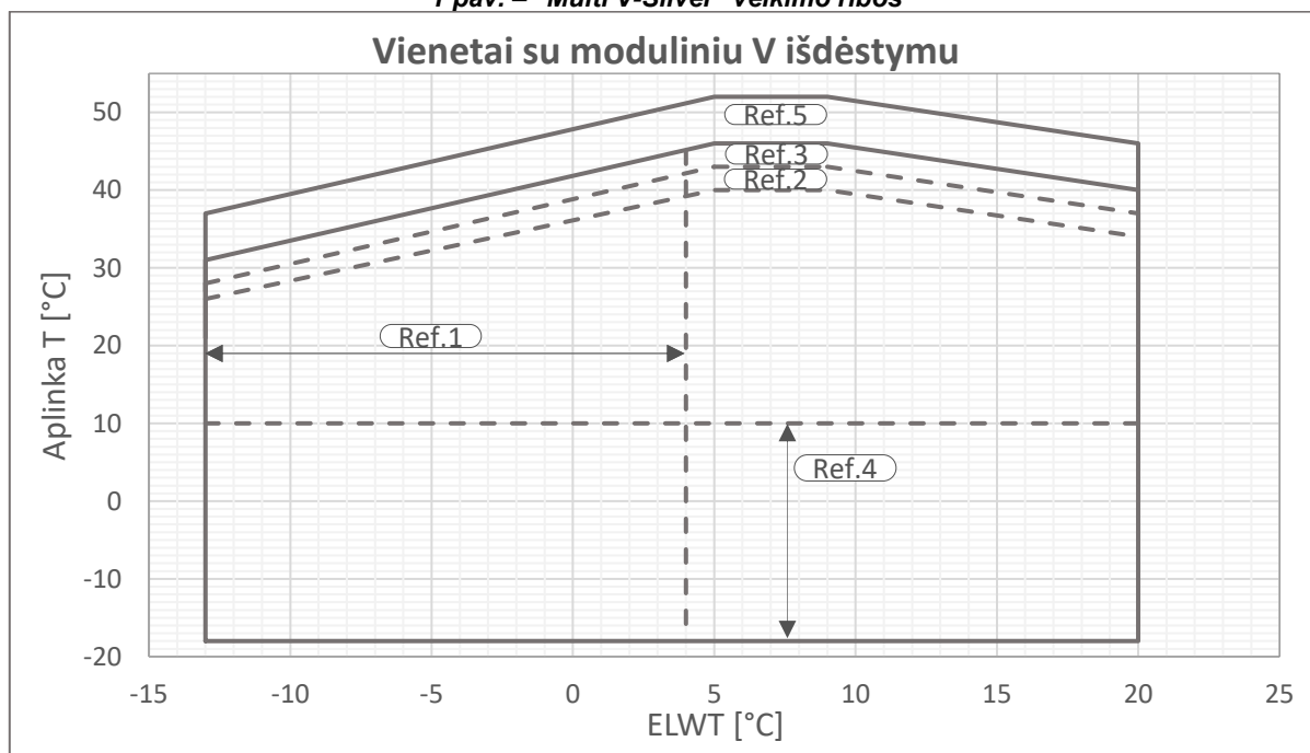
2 pav. – "Multi V-Gold" veikimo ribos
