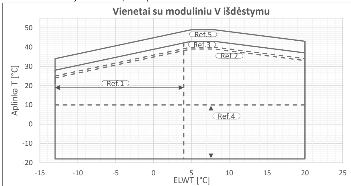
1 pav. – "Multi V-Silver" veikimo ribos
