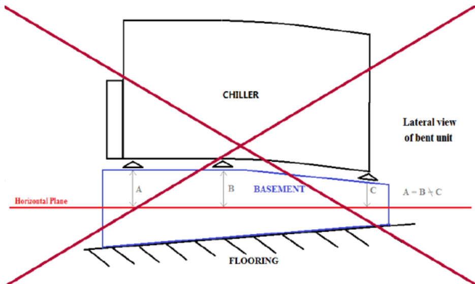
6 pav. – Įrenginio lygiavimas
