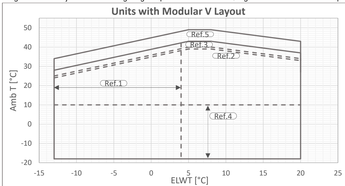
Afb. 1 - Multi V-Silver Bedrijfslimieten
