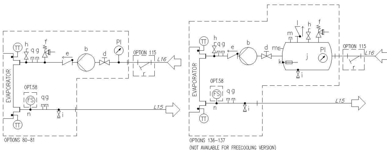
Afb. 11 – Hydraulisch schema voor enkele V (EWATxx5B) dubbele pomp (optie 80-81/136-137) (max. bedrijfsdruk 6 bar)
