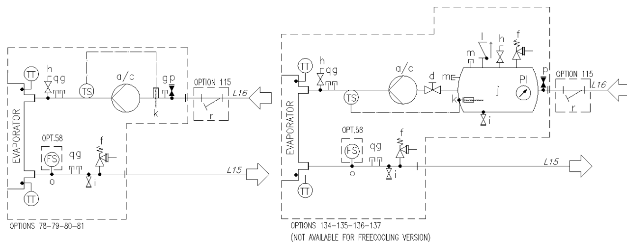
Afb. 12 - Hydraulisch schema voor modulaire V (EWATxx0B) (optie 78-79-80-81/134-135-136-137) (max. bedrijfsdruk 6 bar)
