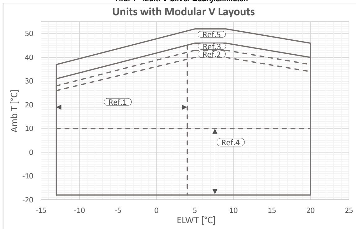
Afb. 2 - Multi V-Gold Bedrijfslimieten
