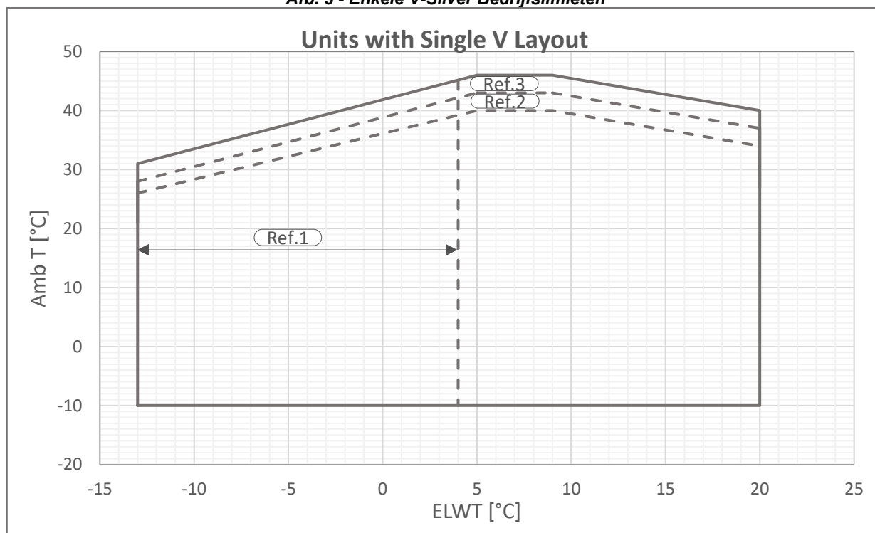
Afb. 4 - Enkele V-Gold Bedrijfslimieten
