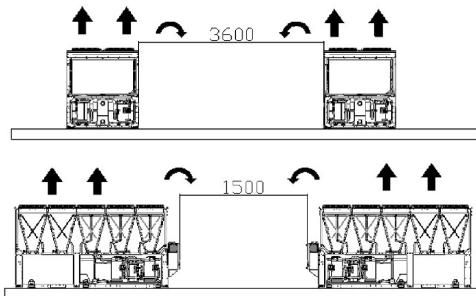
Afb. 7 - Minimaal vereiste afstanden
