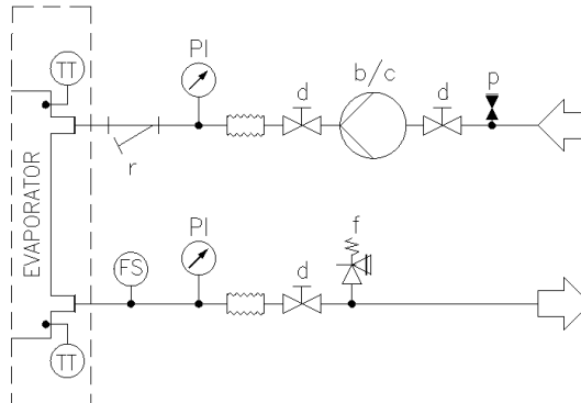
Afb. 9 – Hydraulisch schema zonder pomp(en) aan boord (max. bedrijfsdruk 20 bar)
