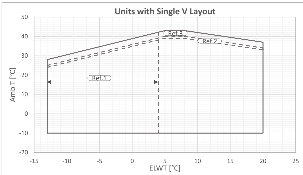
Afb. 3 - Enkele V-Silver Bedrijfslimieten
