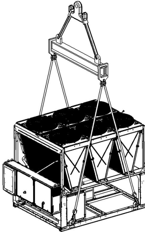
Systeem met 4 hefpunten
