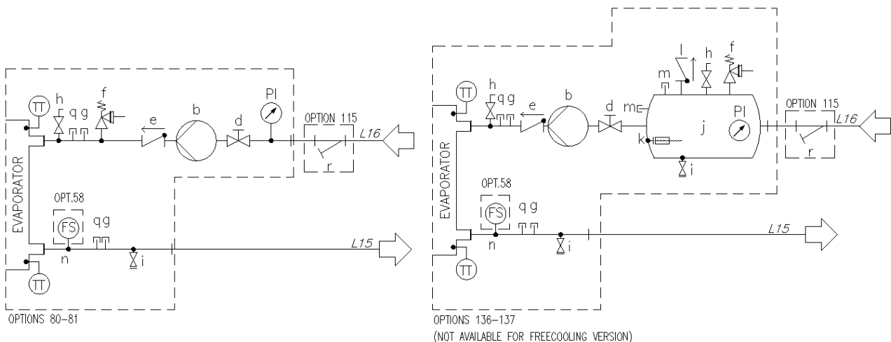
Afb. 10 – Hydraulisch schema voor enkele V (EWATxx5B) enkele pomp (optie 78-79/134-135) (max. bedrijfsdruk 6 bar)
