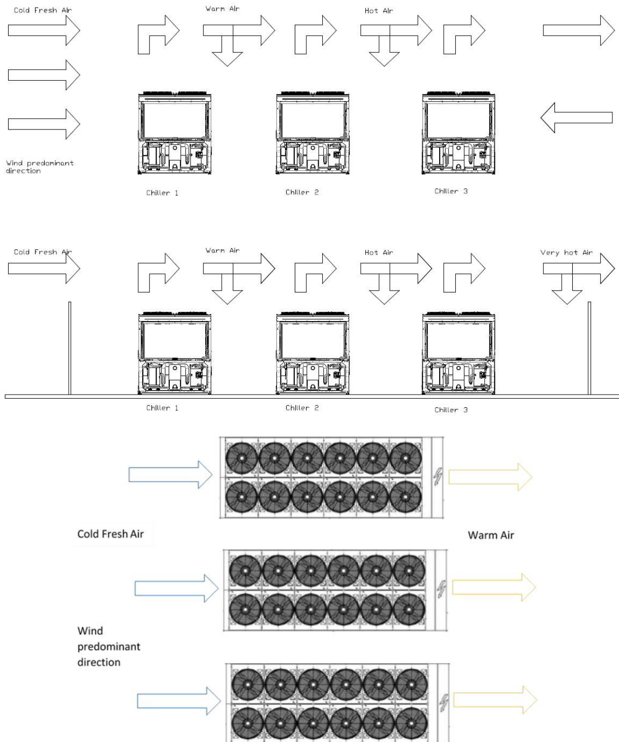
Afb. 8 – Installatie meerdere koelers
