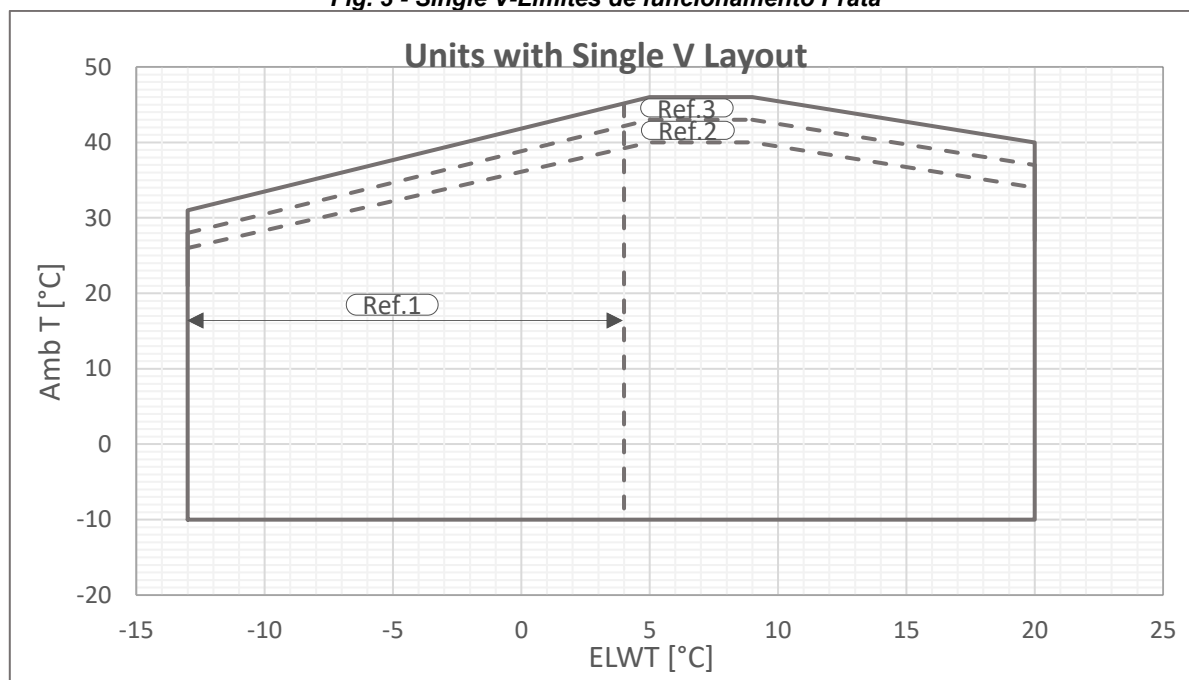
Fig. 4 - Single V-Limites de funcionamento Ouro
