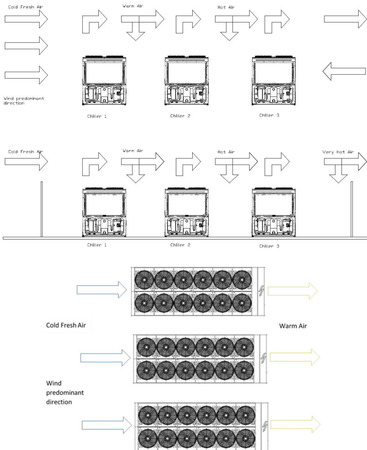
Fig. 8 - Instalação de múltiplos refrigeradores
