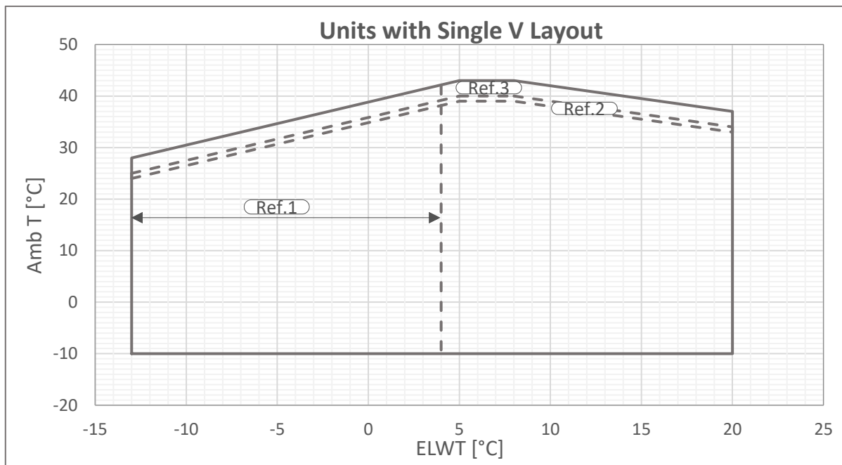
Fig. 3 - Single V-Limites de funcionamento Prata
