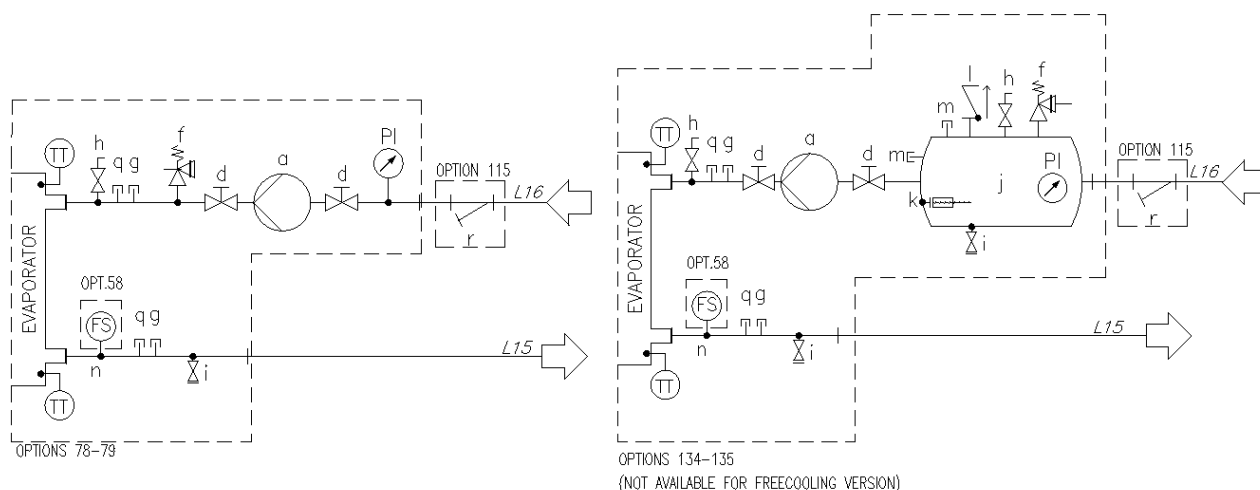
Fig. 10 - Diagrama hidráulico para bomba única V (EWATxx5B) (opc. 78-79/134-135) (pressão máxima de funcionamento 6 bar)
