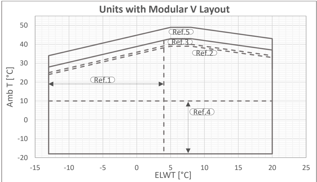
Fig. 1 - Multi V-Limites de funcionamento Prata
