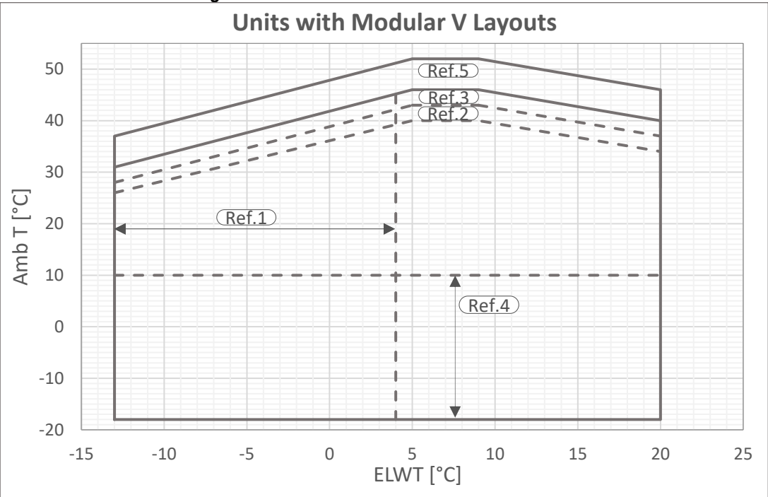
Fig. 2 - Multi V-Limites de funcionamento Ouro
