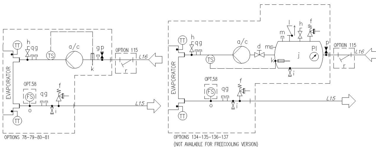
Fig. 12 - Diagrama hidráulico para Modular V (EWATxx0B) (opc. 78-79-80-81/134-135-136-137) (pressão máxima de funcionamento 6 bar)
