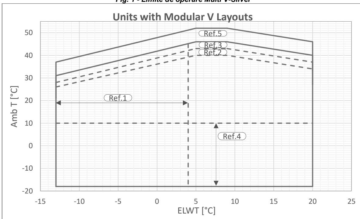
Fig. 2 - Limite de operare Multi V-Gold
