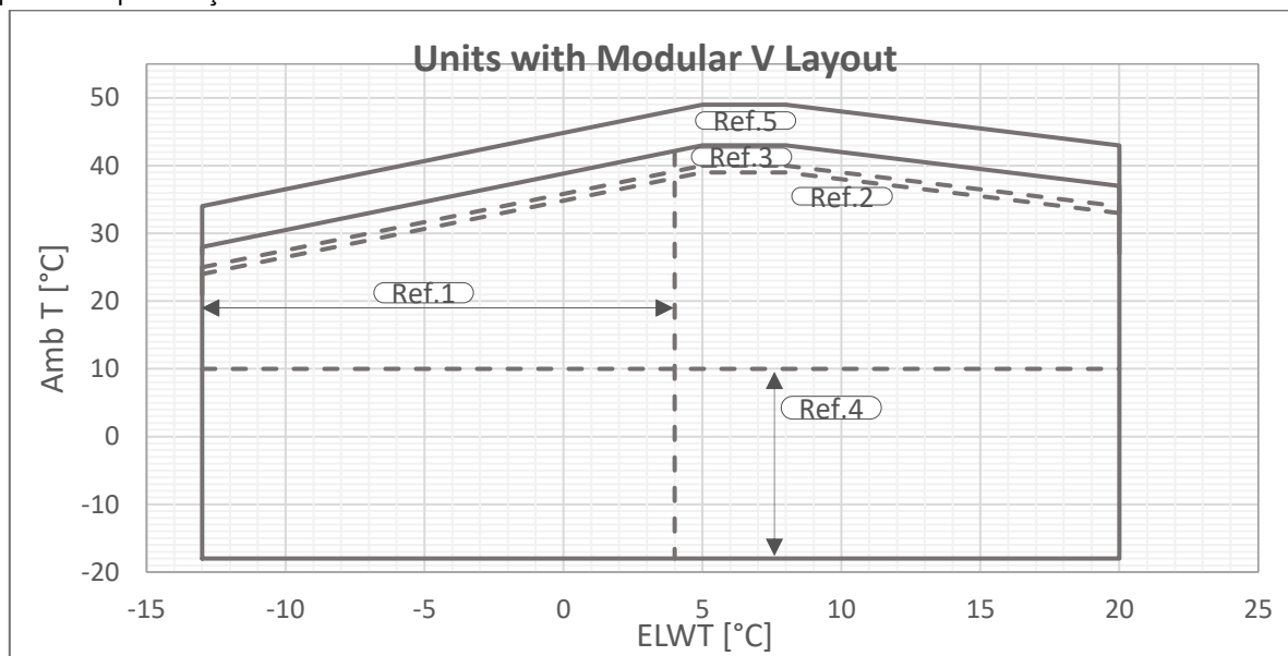
Fig. 1 - Limite de operare Multi V-Silver
