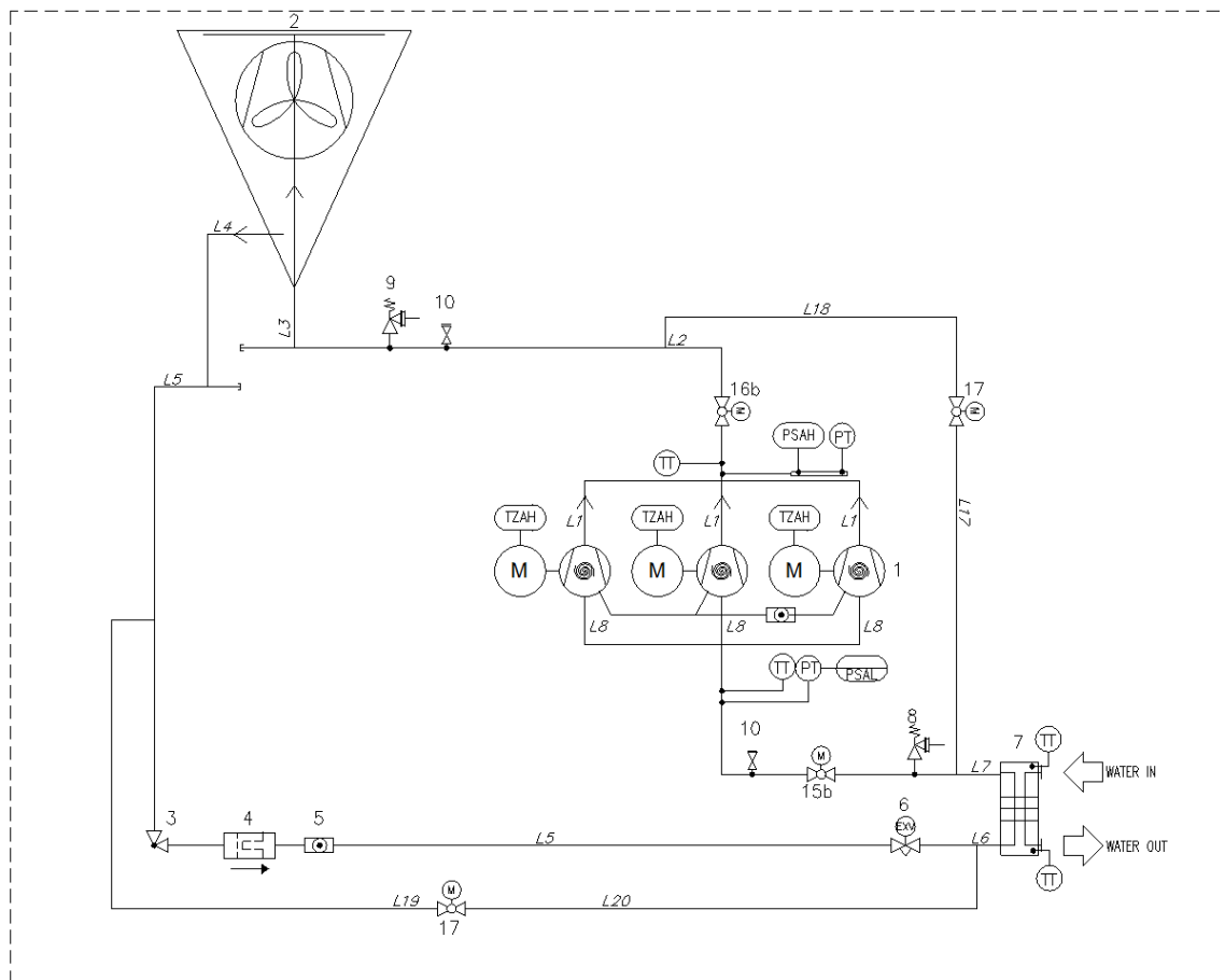
Fig. 14 - Diagrama circuitului frigorific (P & ID), unitate cu un singur circuit cu opțiunea de răcire liberă ușoară
