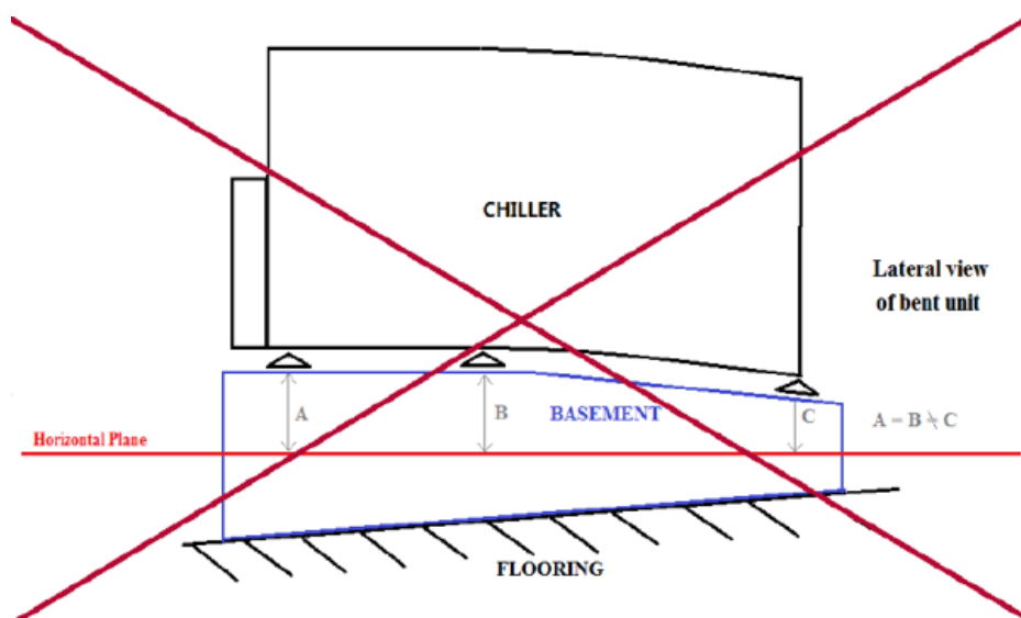
Fig. 6 - Aducerea la nivel a unității
