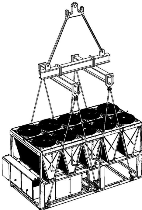
Unitate cu 6 puncte de ridicare
