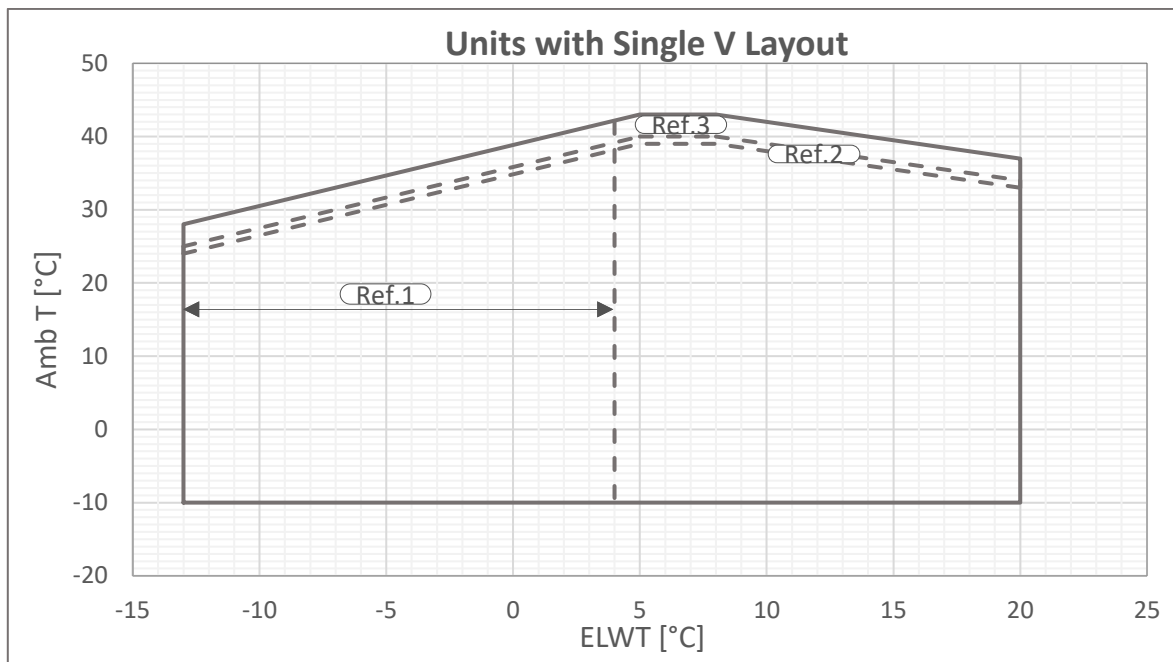
Fig. 3 - Limite de operare Single V-Silver
