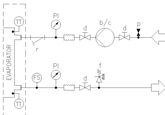
Fig. 9 – Diagrama hidraulică fără pompă (e) la bord (presiune max. de operare 20 de bari)
