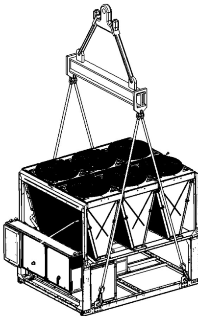
Unitate cu 4 puncte de ridicare
