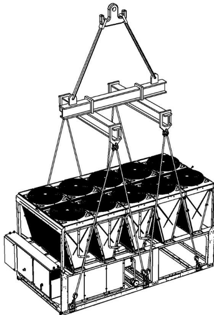
Jednotka so 6 zdvíhacími bodmi
