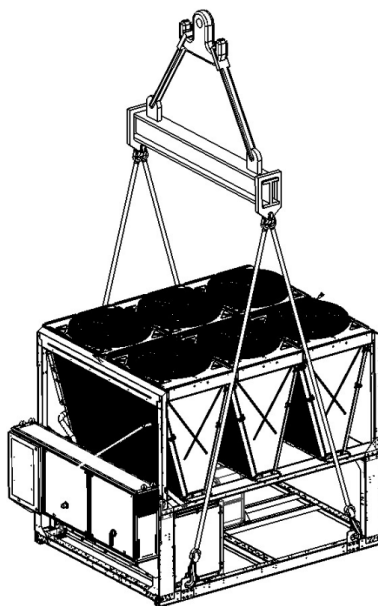
Jednotka so 4 zdvíhacími bodmi
