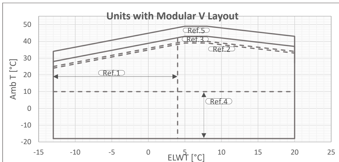
Obr. 1 – Prevádzkové limity Multi V-Silver
