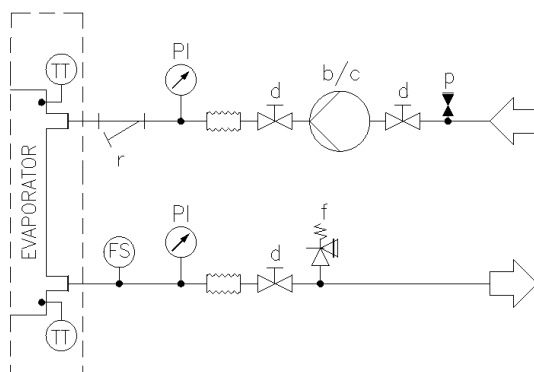
Slika 9 – hidravlična shema brez črpalk(e) na plošči (največji delovni tlak 20 barov)
