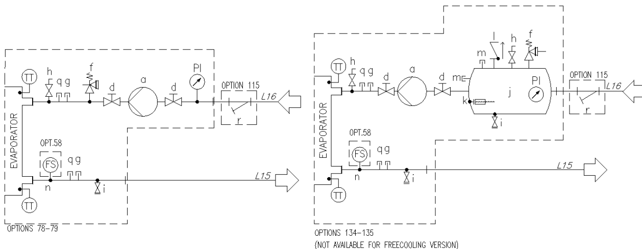
Slika 10 – hidravlična shema za eno V (EWATxx5B) z enojno črpalko (št. 78-79/134-135) (največji delovni tlak 6 bar)
