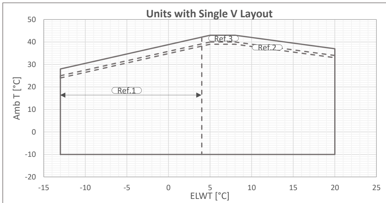
Slika 3 – Mejne delovne vrednosti za eno enoto V-Silver
