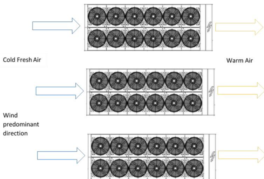
Slika 8 – Namestitev več hladilnikov
