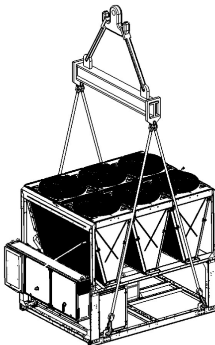
Enota s 4 dvížnimi točkami
