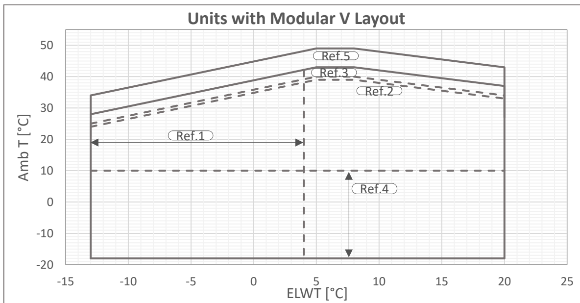
Slika 1 – Mejne delovne vrednosti za več enot V-Silver
