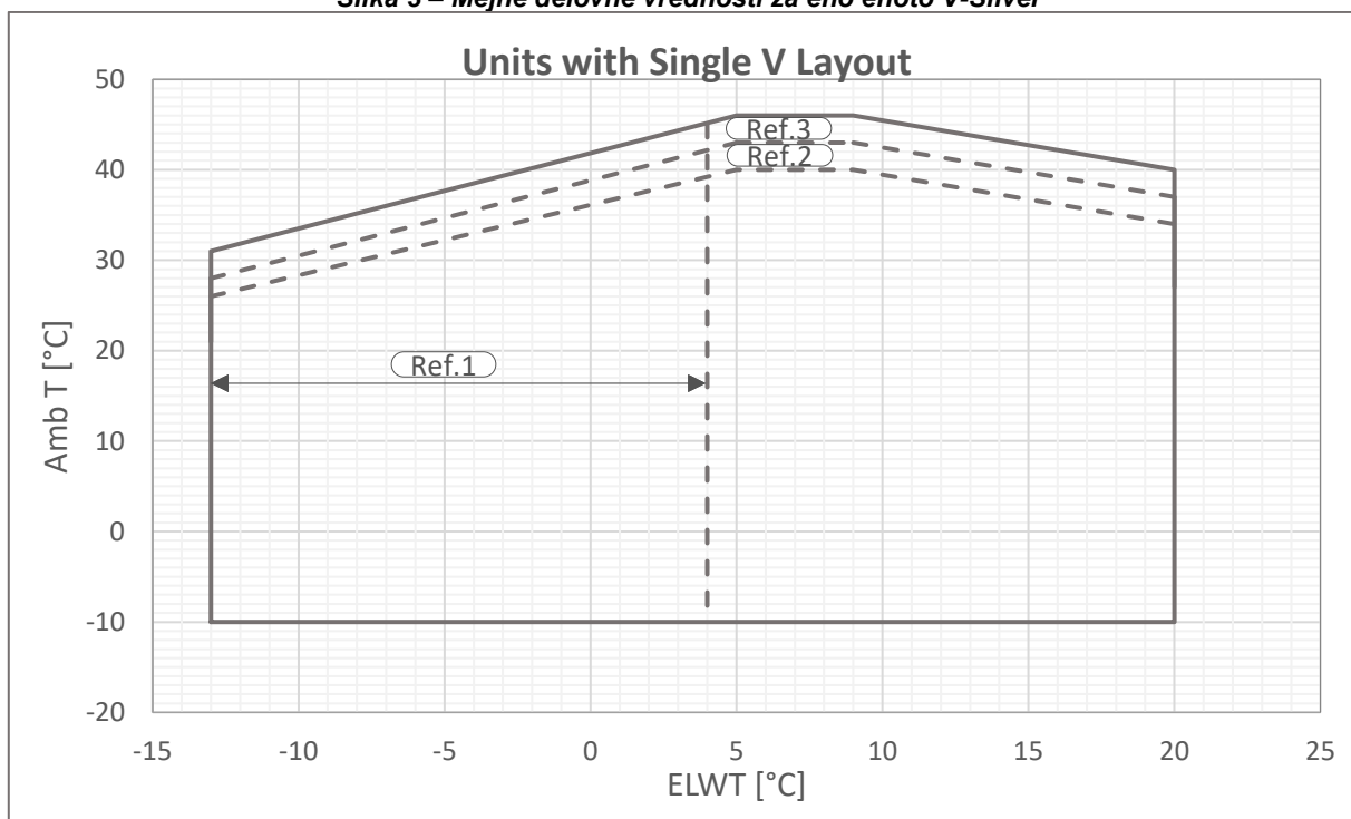
Slika 4 – Mejne delovne vrednosti za eno enoto V-Gold
