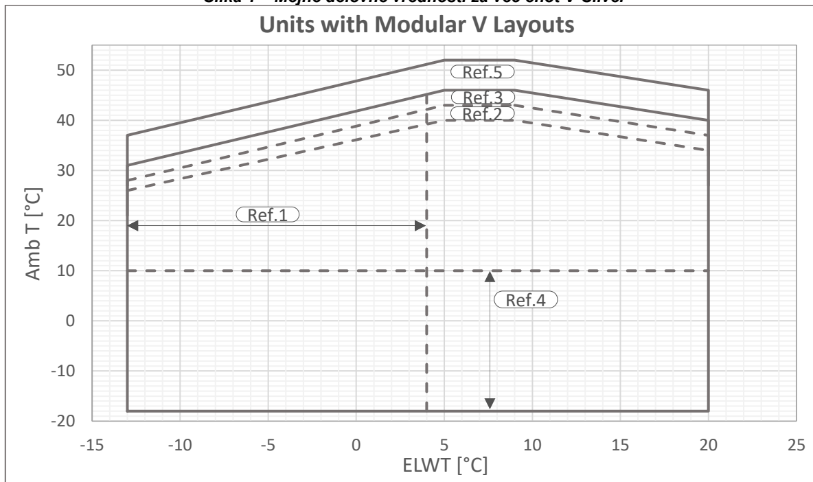
Slika 2 – Mejne delovne vrednosti za več enot V-Gold
