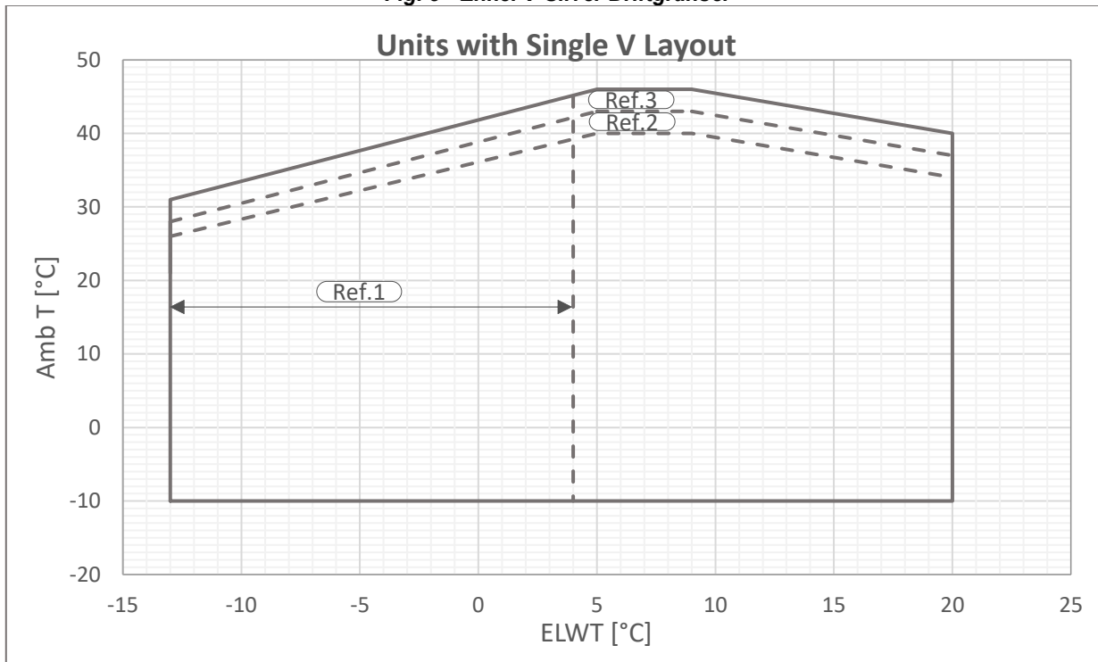
Fig. 4 - Enkel V-Gold Driftgränser
