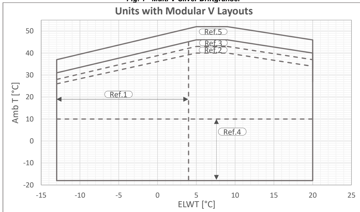
Fig. 2 - Multi V-Gold Driftgränser
