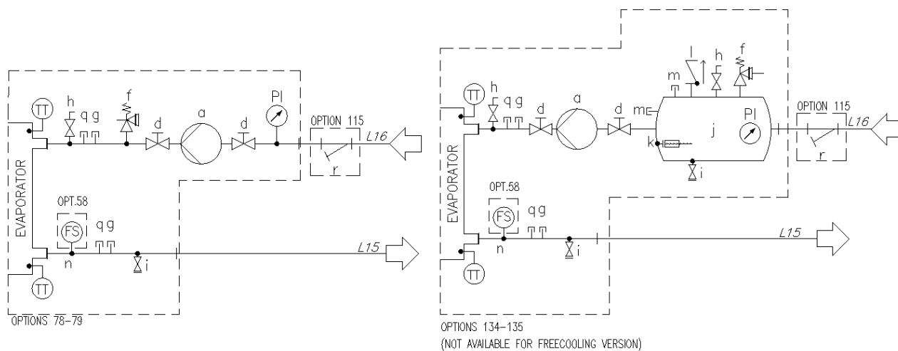
Fig. 10 – Hydraulisk diagram för enkel V (EWATxx5B) enkel pump (alt.78-79/134-135) (max arbetstryck 6 bar)
