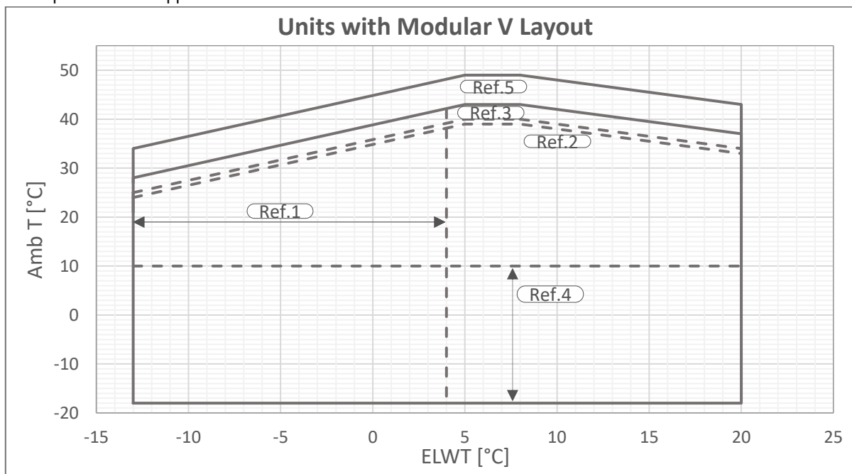
Fig. 1 - Multi V-Silver Driftgränser
