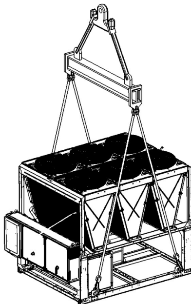
Enhet med fyra lyftpunkter
