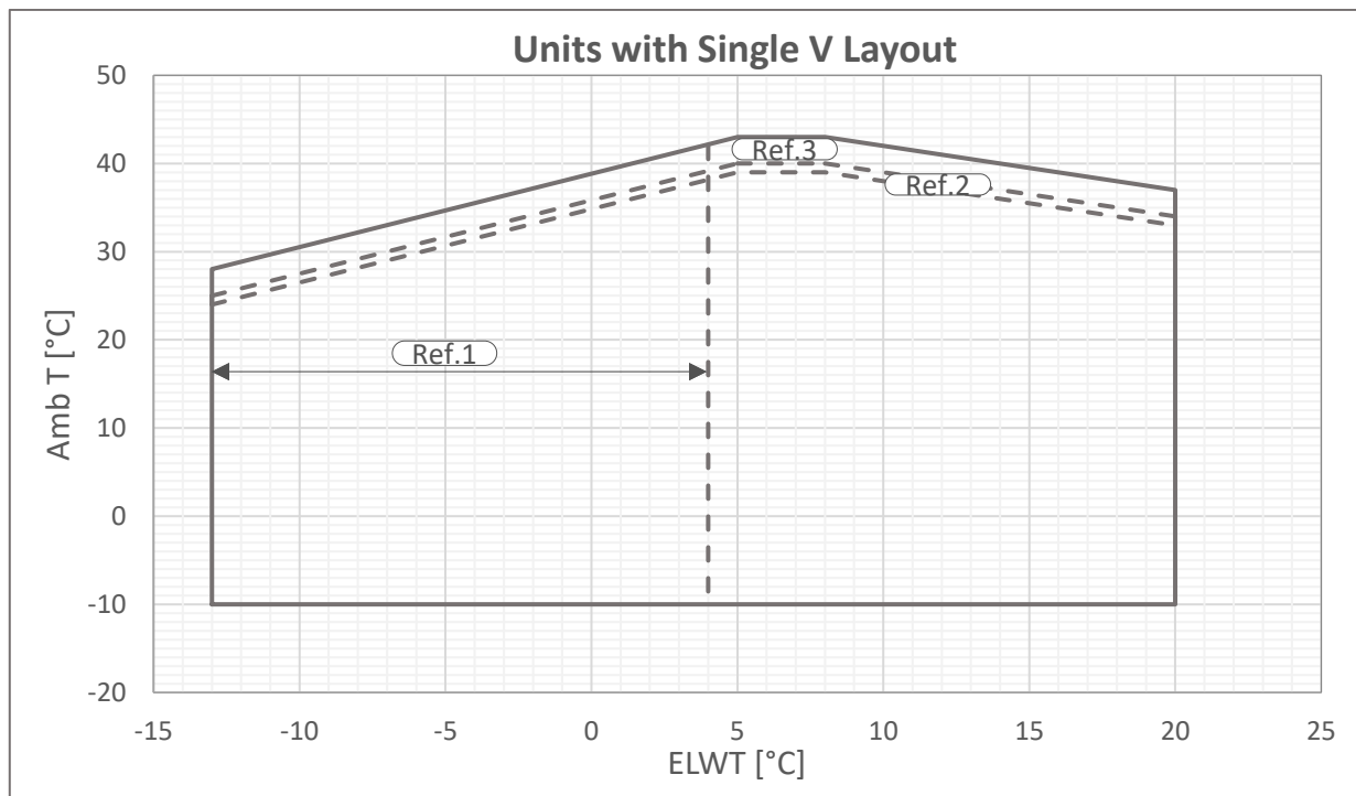
Fig. 3 - Enkel V-Silver Driftgränser
