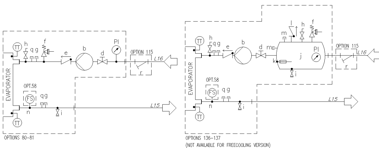
Fig. 11 – Hydrauliskt diagram för enkel V (EWATxx5B) dubbelpump (alt.80-81/136-137) (max arbetstryck 6 bar)
