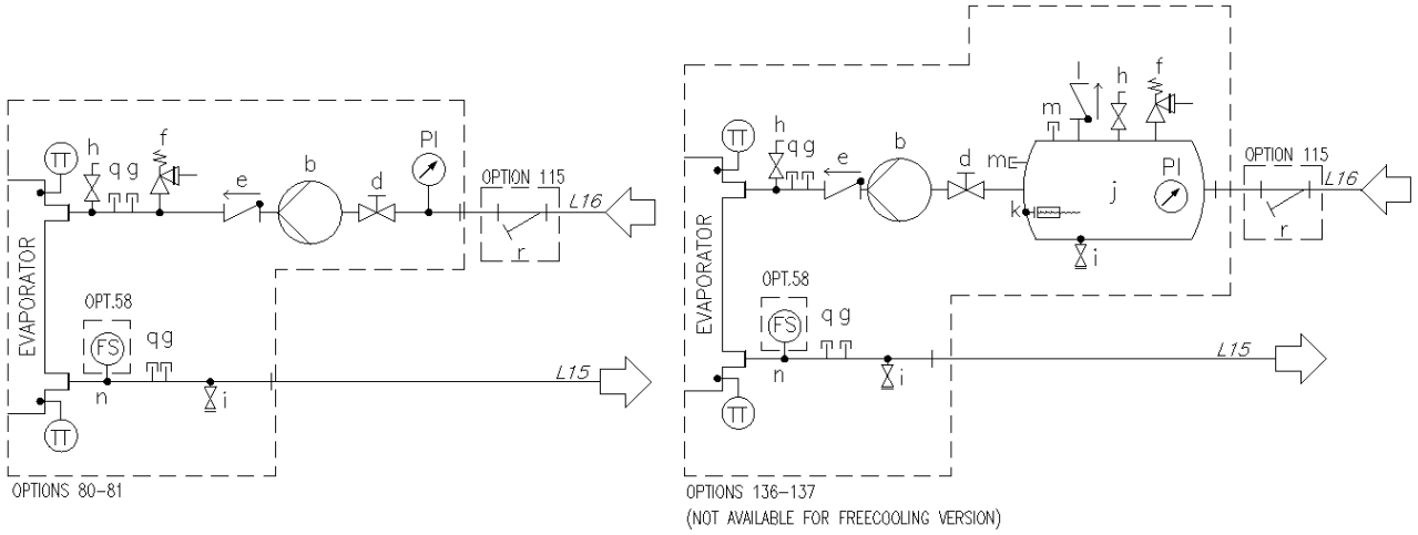
Şekil 11 – Tek V (EWATxx5B) çift pompa için hidrolik diyagram (ops. 80-81/136-137) (maks. çalışma basıncı 6 bar)
