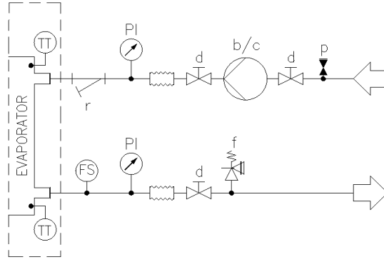
Şekil 9 – Cihazda pompa(lar) olmadan hidrolik diyagram (maks. çalışma basıncı 20 bar)
