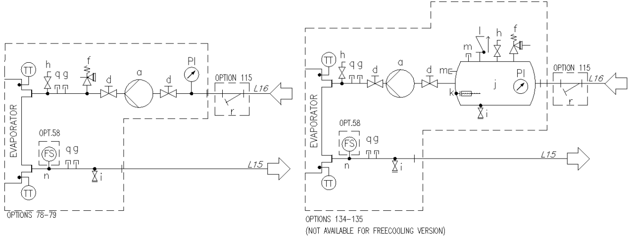
Şekil 10 – Tek V (EWATxx5B) tek pompa için hidrolik diyagram (ops. 78-79/134-135) (maks. çalışma basıncı 6 bar)
