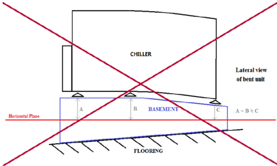
Şekil 6 - Birimin tesviyesi
