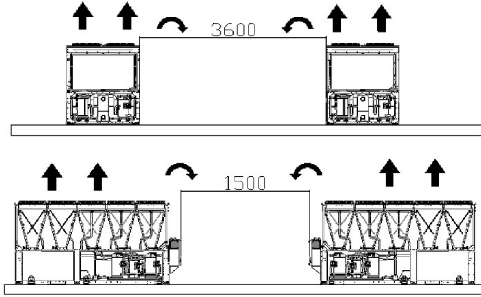
Şekil 7 - Minimum alan gereksinimleri
