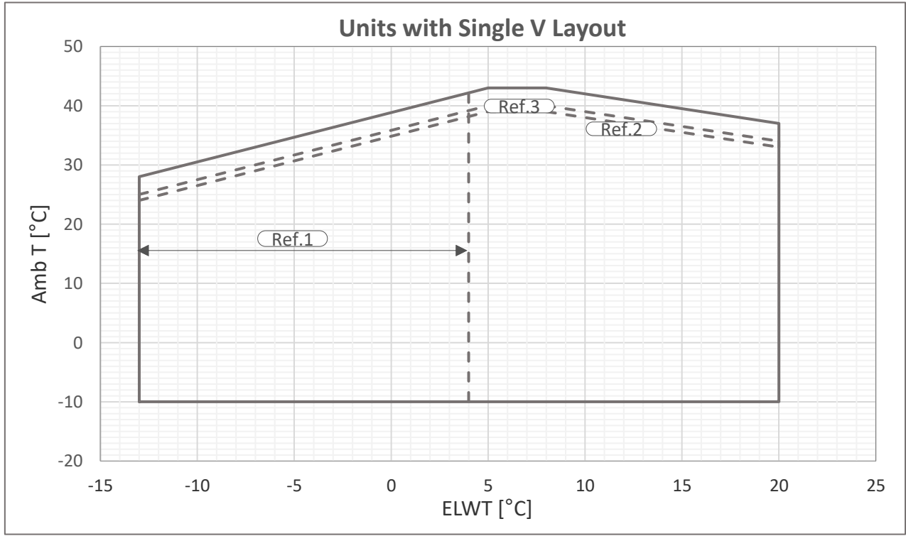
Şekil 3 - Tek V-Gümüş Çalışma sınırları
