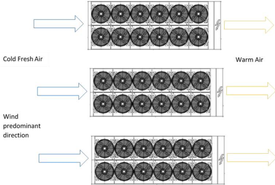
Şekil 8 – Çoklu Soğutucu Kurulumu
