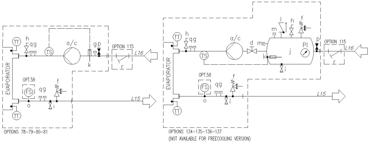
Şekil 12 - Modüler V (EWATxx0B) için hidrolik diyagram (ops. 78-79-80-81/134-135-136-137) (maks. çalışma basıncı 6 bar)
