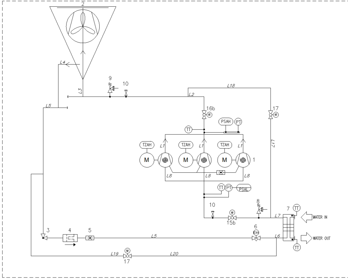
Şekil 14 - Hafif serbest soğutma opsiyonlu tek devre üniteli soğutucu akışkan devre şeması (P&ID)
